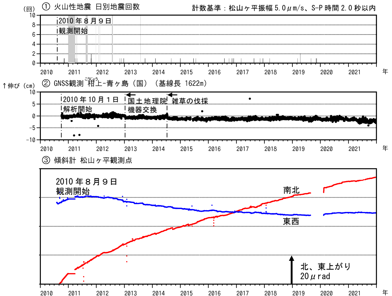
図3 青ヶ島 火山活動経過図 (2010年8月9日～2021年12月31日)
