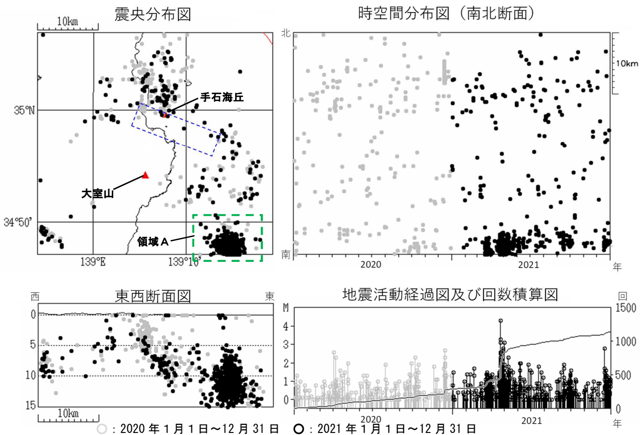
図2 伊豆東部火山群 広域地震観測網による震源分布図（2020年1月～2021年12月）
