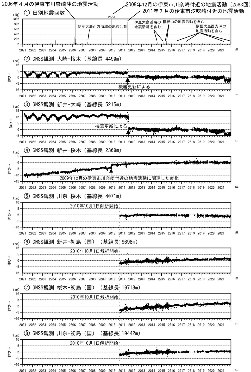
図3 伊豆東部火山群 最近の火山活動経過図 (2001年1月～2021年12月)
