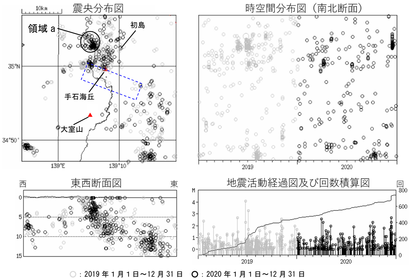
図2 伊豆東部火山群 広域地震観測網による震源分布図 (2019年1月~2020年12月)
