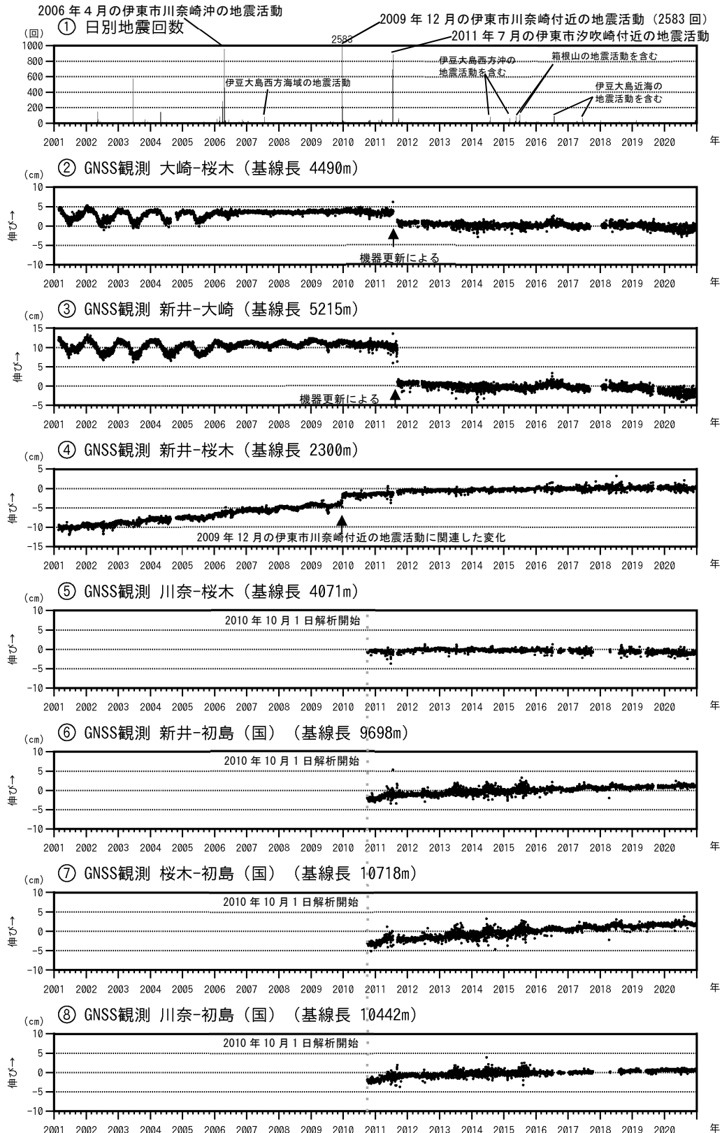
図3 伊豆東部火山群 最近の火山活動経過図 (2001年1月~2020年12月)
