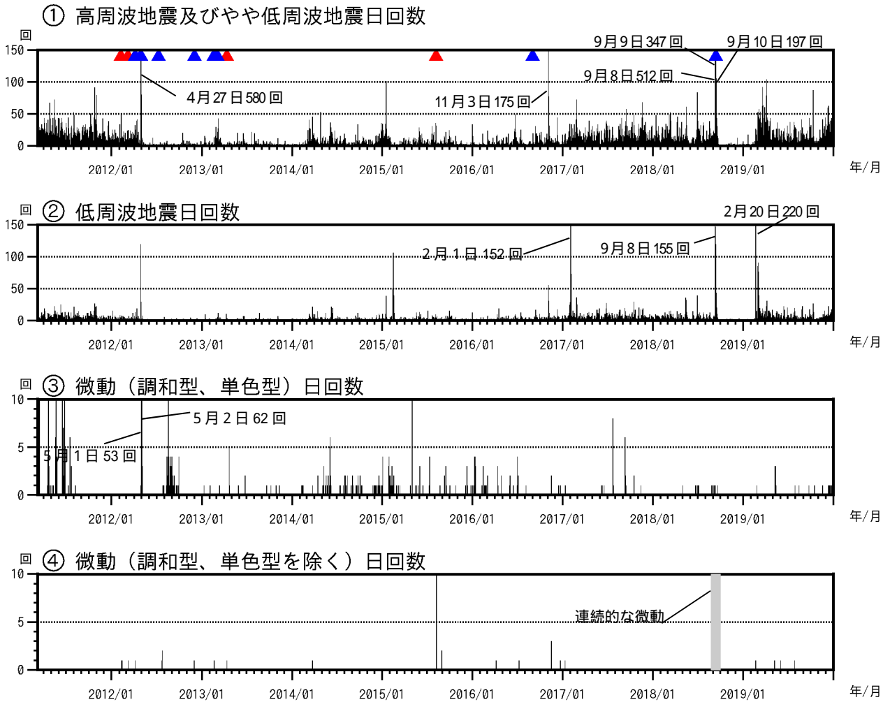
図4 硫黄島 火山活動経過図（2011年3月8日～2019年12月31日）
