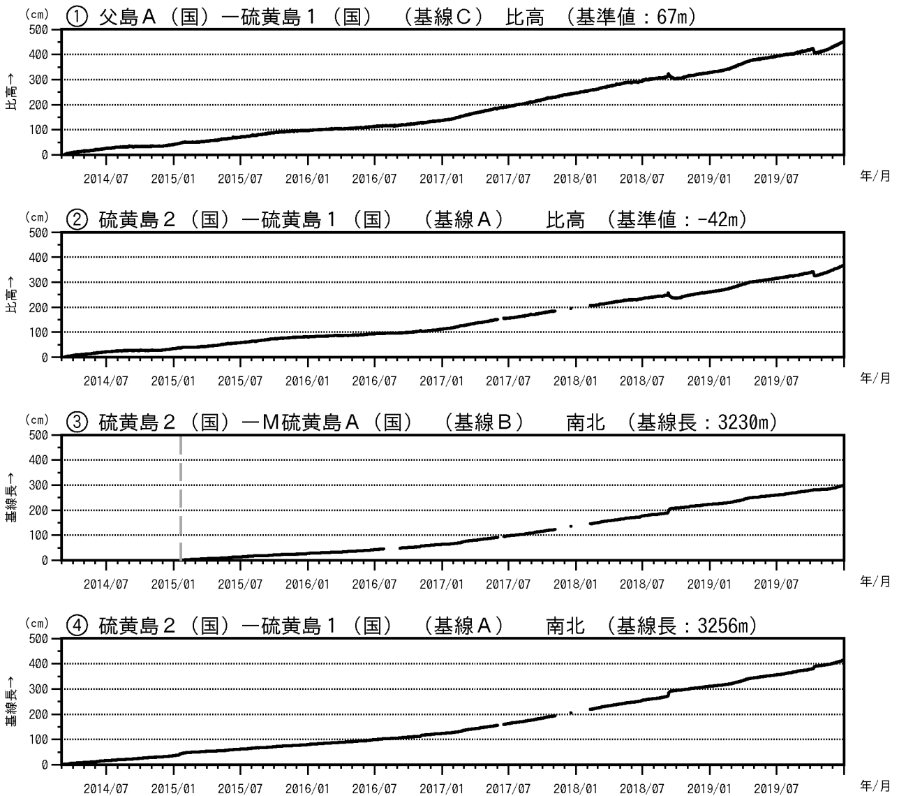
図5 硫黄島 GNSS 連続観測結果 (2014年3月1日~2019年12月31日)
