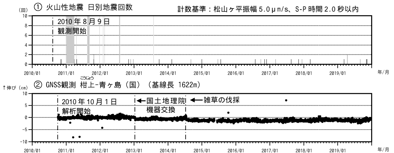
図3 青ヶ島 火山活動経過図（2010年8月9日～2019年12月31日） グラフの灰色部分は機器障害による欠測。 （国）：国土地理院、図4のGNSS基線 に対応。グラフの空白部分は欠測。
