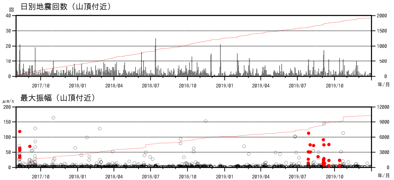
図4 焼岳 山頂付近の地震回数、および南峰南東観測点上下動最大振幅 (2017年8月1日～2019年12月31日)
