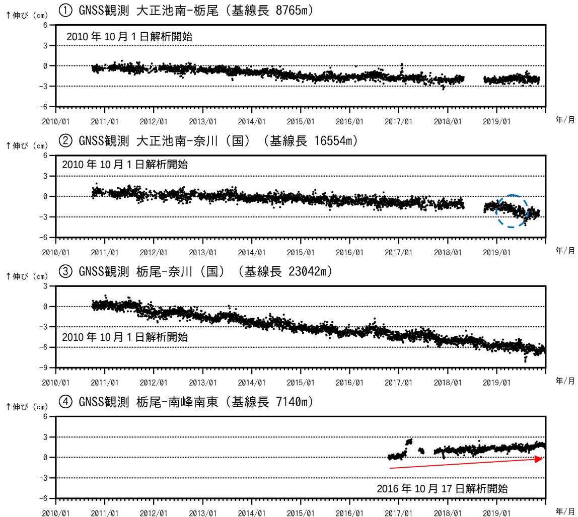
図6 焼岳 GNSS 連続観測による基線長変化 (2010年10月1日～2019年12月31日)
