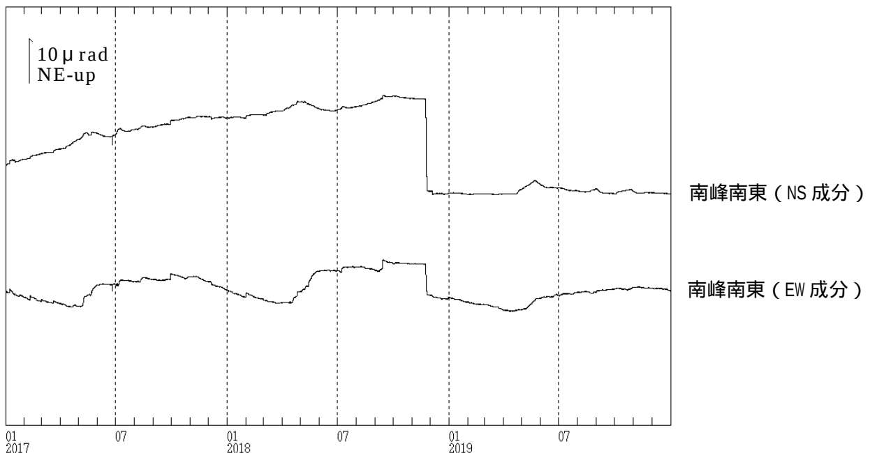
図7 焼岳 南峰南東観測点における傾斜データ (2017年1月1日～2019年12月31日)
