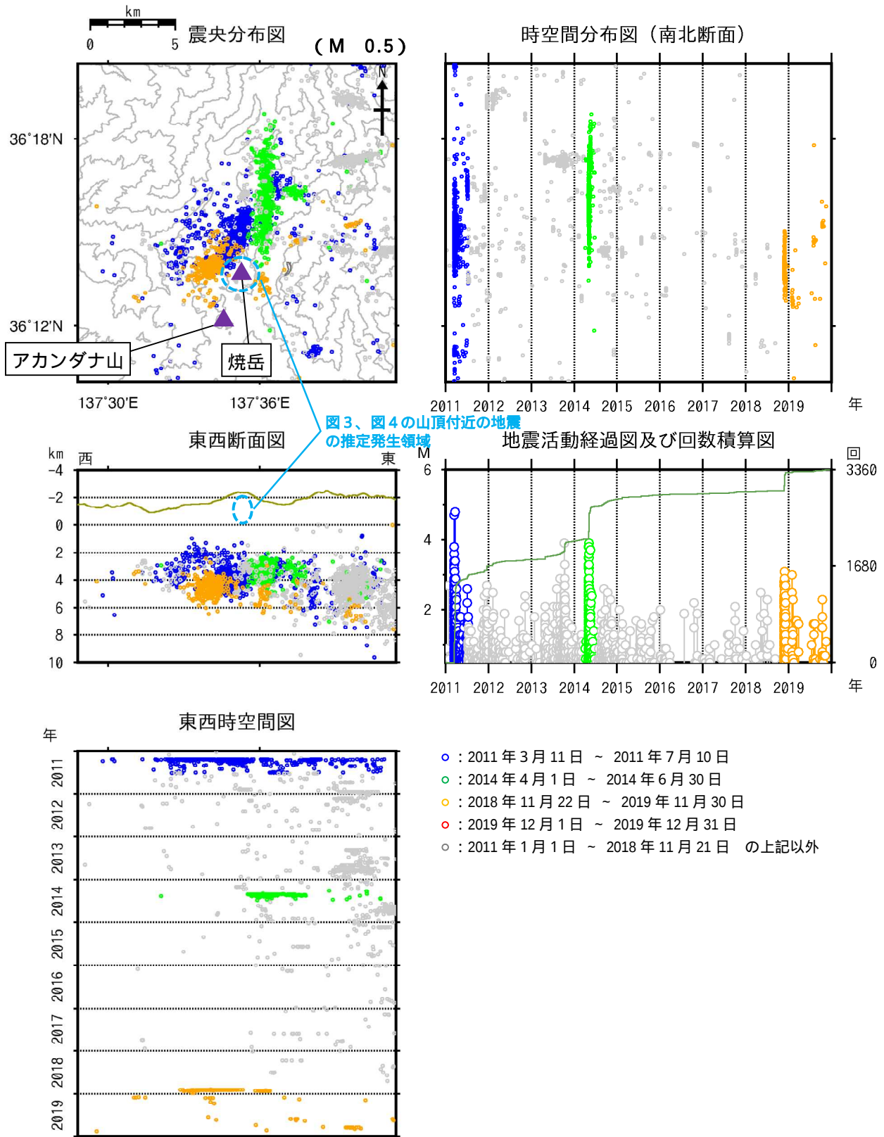
図5 焼岳 広域地震観測網による山体及び周辺の地震活動(2011年1月1日～2019年12月31日)
