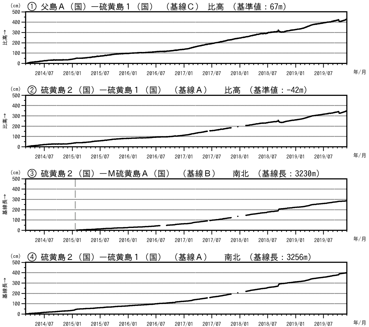
図5 硫黄島 GNSS 連続観測結果（2014年3月1日～2019年11月30日）
