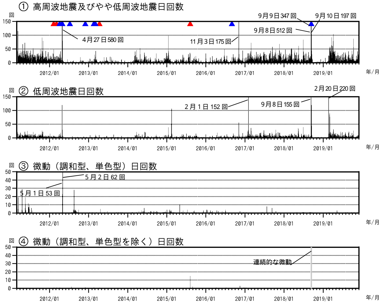
図4 硫黄島 火山活動経過図（2011年3月8日～2019年11月30日）
