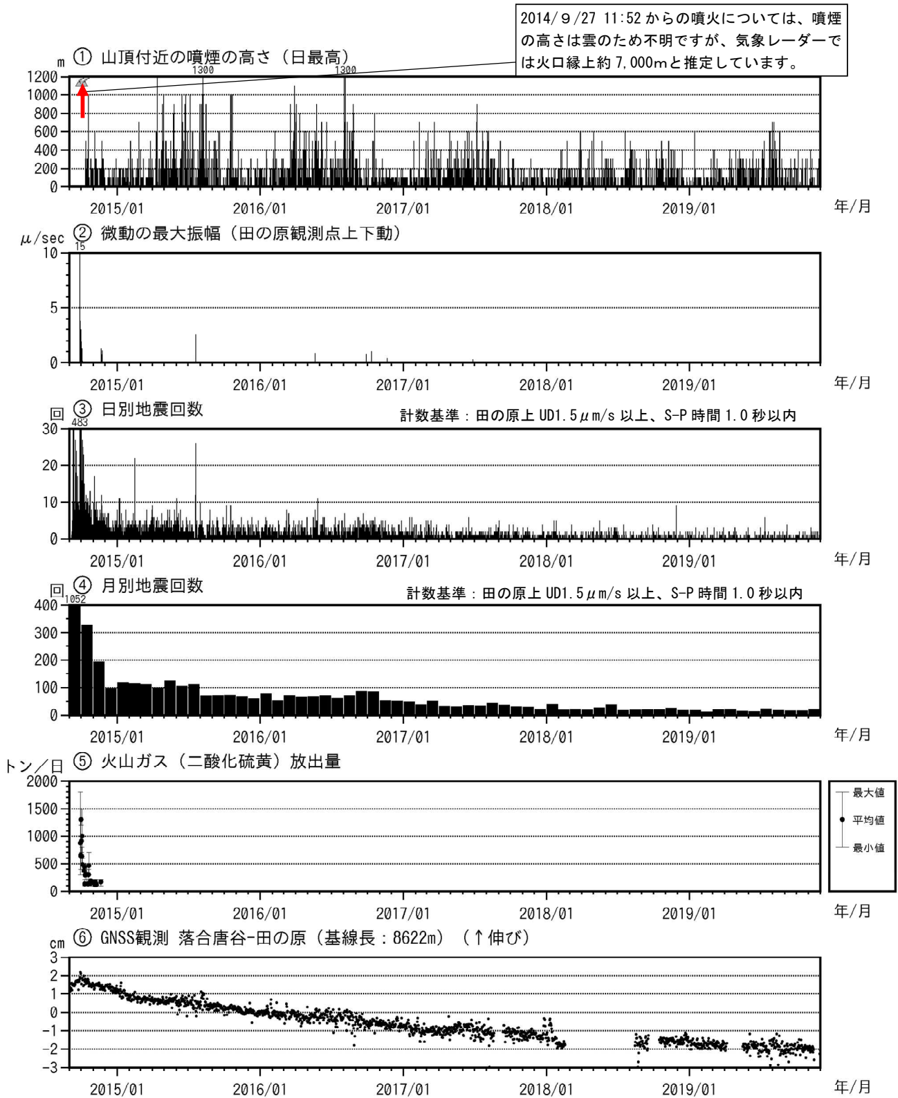
図4 御嶽山 最近の火山活動経過図（2014年9月1日～2019年11月30日）
