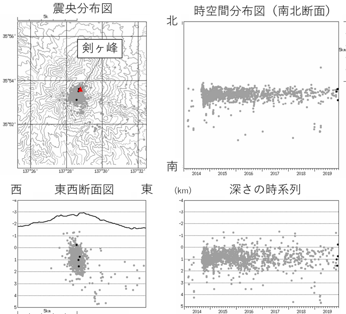
図2 御嶽山 震源分布図（2014年1月1日～2019年11月30日）
