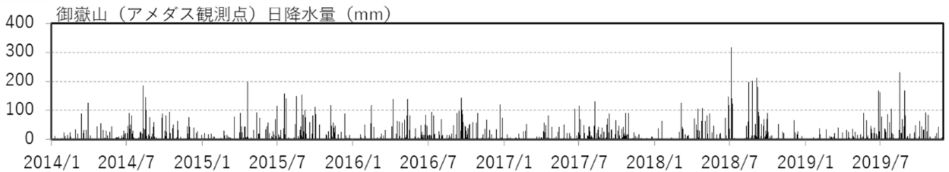
図7 御嶽山 田の原観測点の傾斜変動（2014年1月1日～2019年11月30日）
