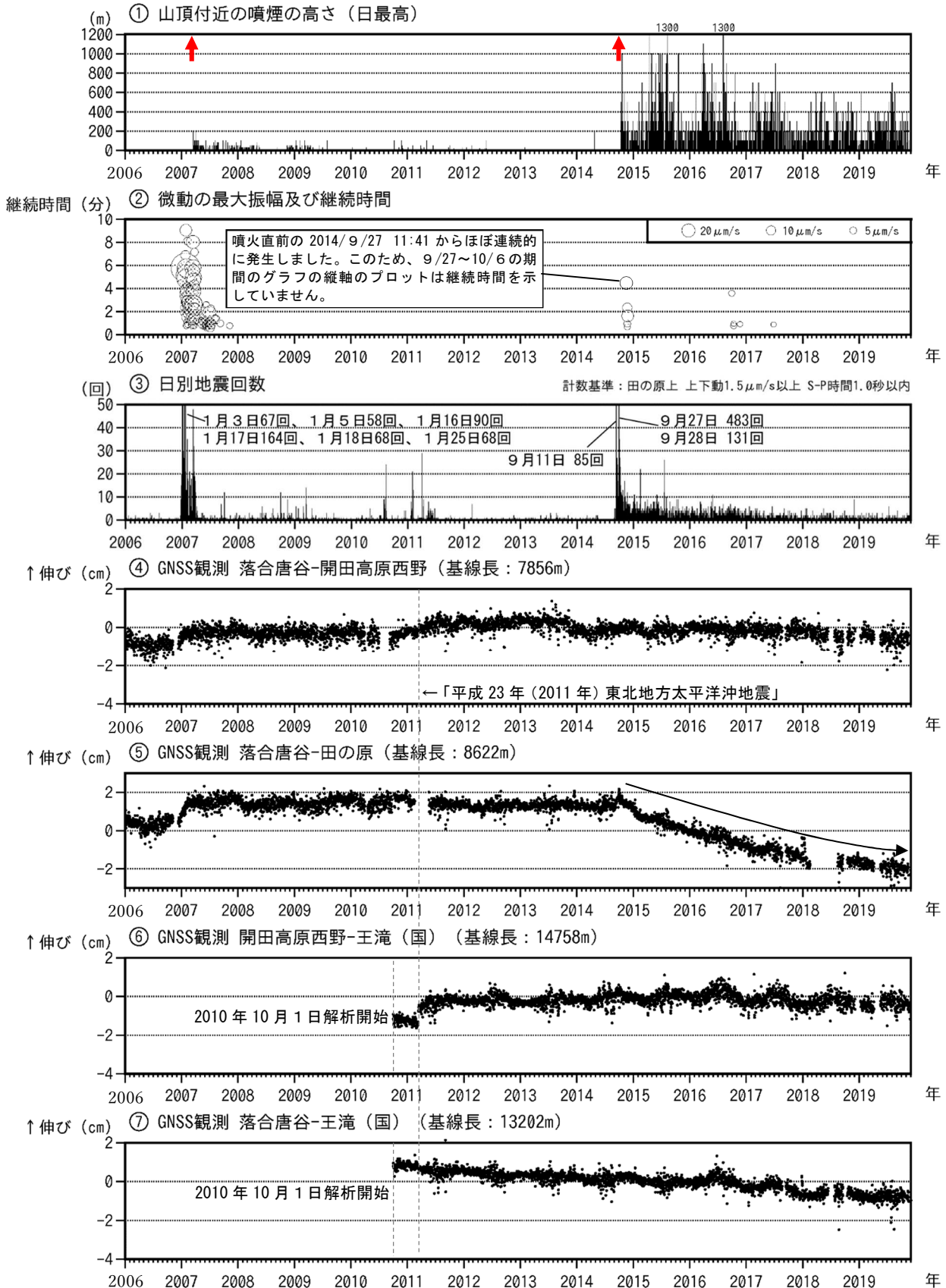
図5 御嶽山 長期間の火山活動経過図（2006年1月1日～2019年11月30日）
