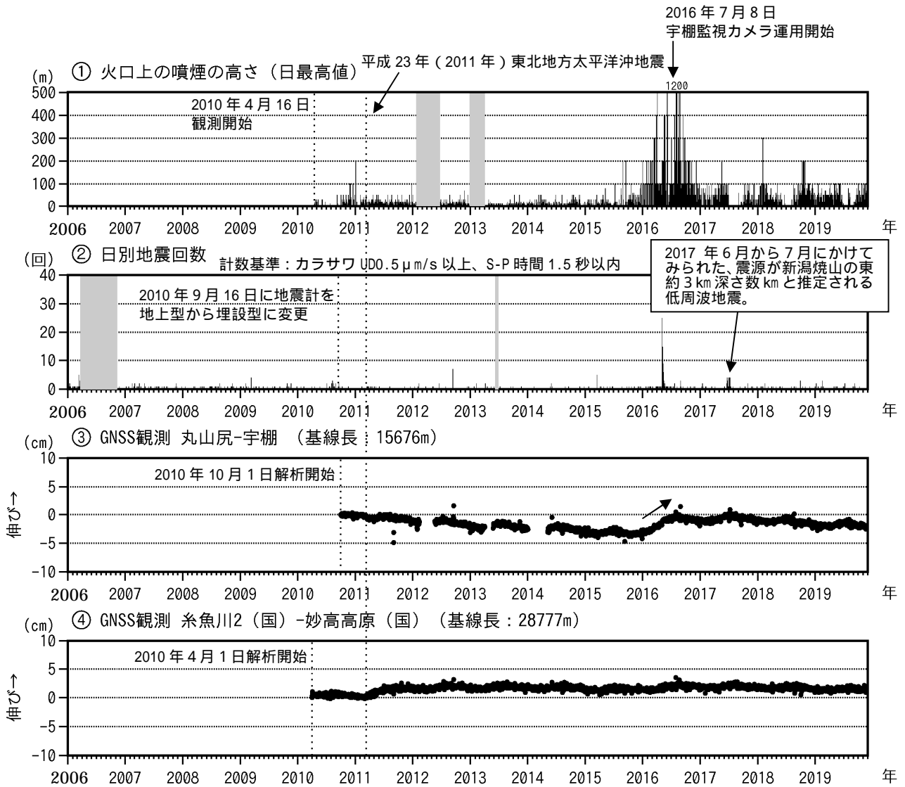
図3 新潟焼山 火山活動経過図（2006年1月1日～2019年11月30日）
