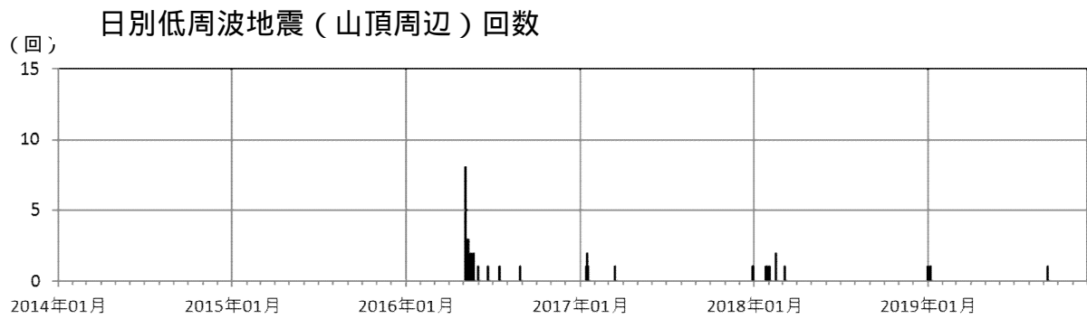
図6 新潟焼山 日別地震回数（2014年1月1日～2019年11月30日）
