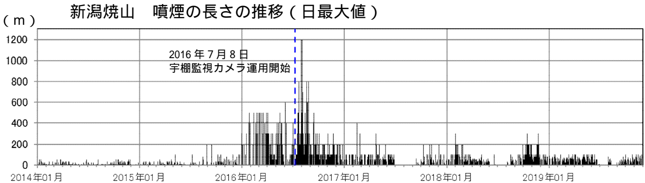
図4 新潟焼山 噴煙高度と噴煙の長さの推移
