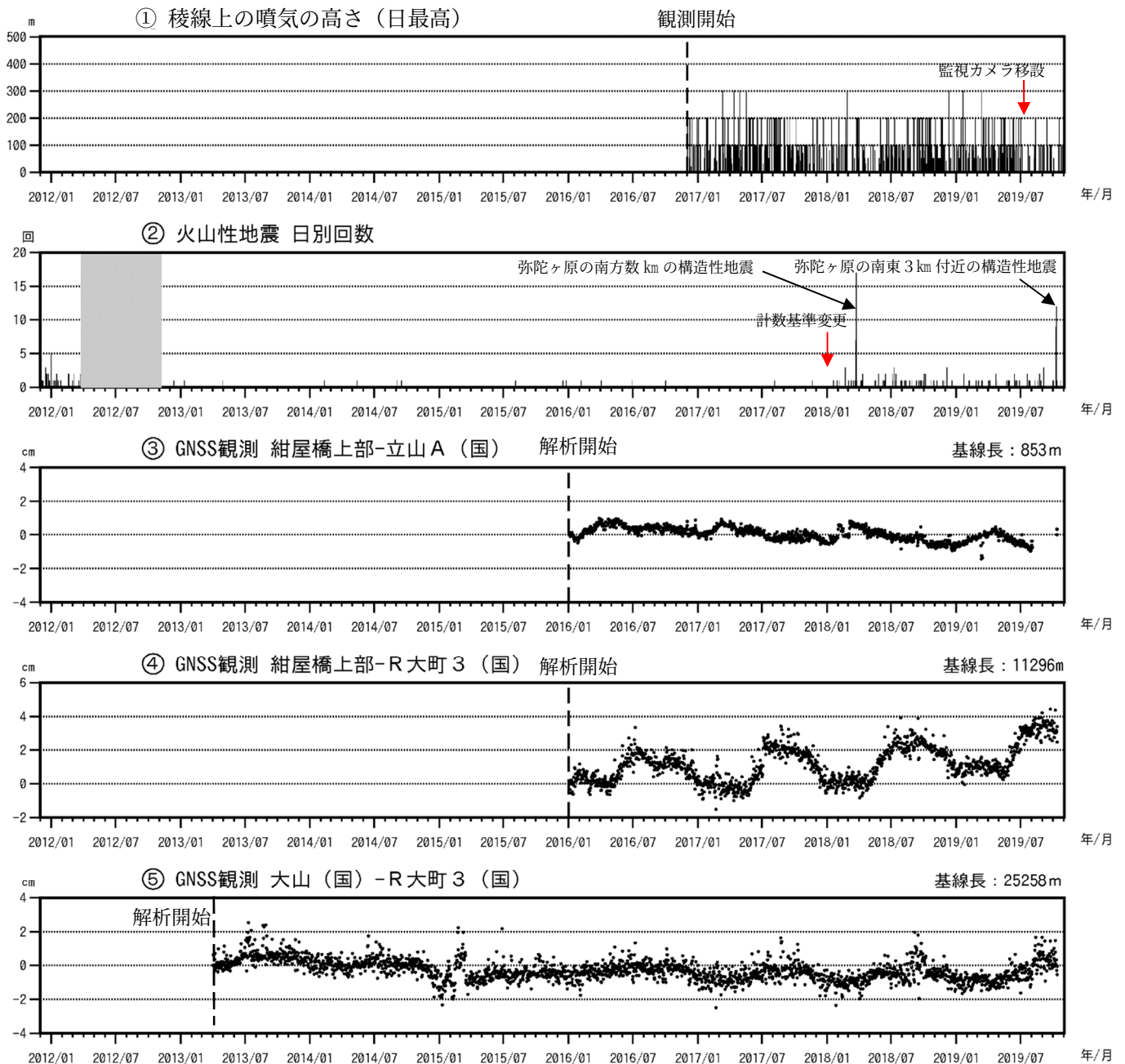
図3 弥陀ヶ原 火山活動経過図（2011 年 12 月 1 日～2019 年 10 月 31 日）
