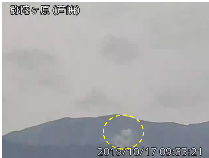
図 1 弥陀ヶ原 地獄谷からの噴気の状況（黄丸）（10 月 17 日、芦峯監視カメラによる）
