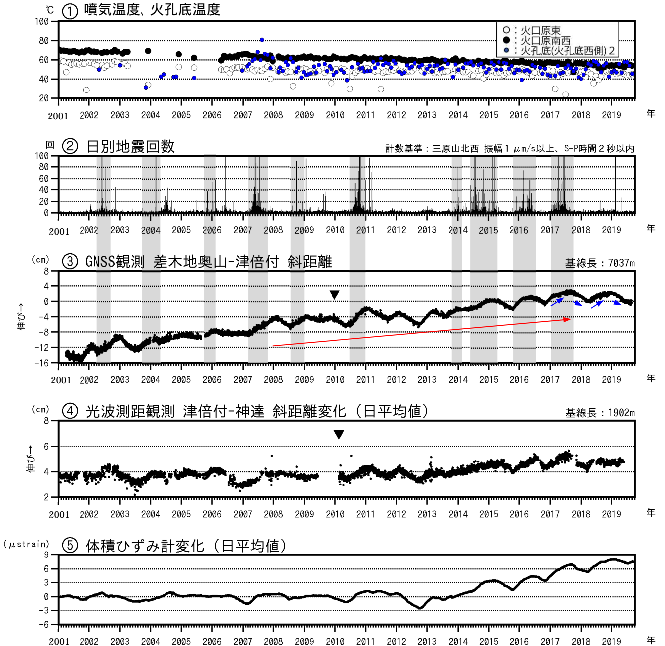
図2 伊豆大島 最近の火山活動経過図（2001年1月～2019年9月30日）
