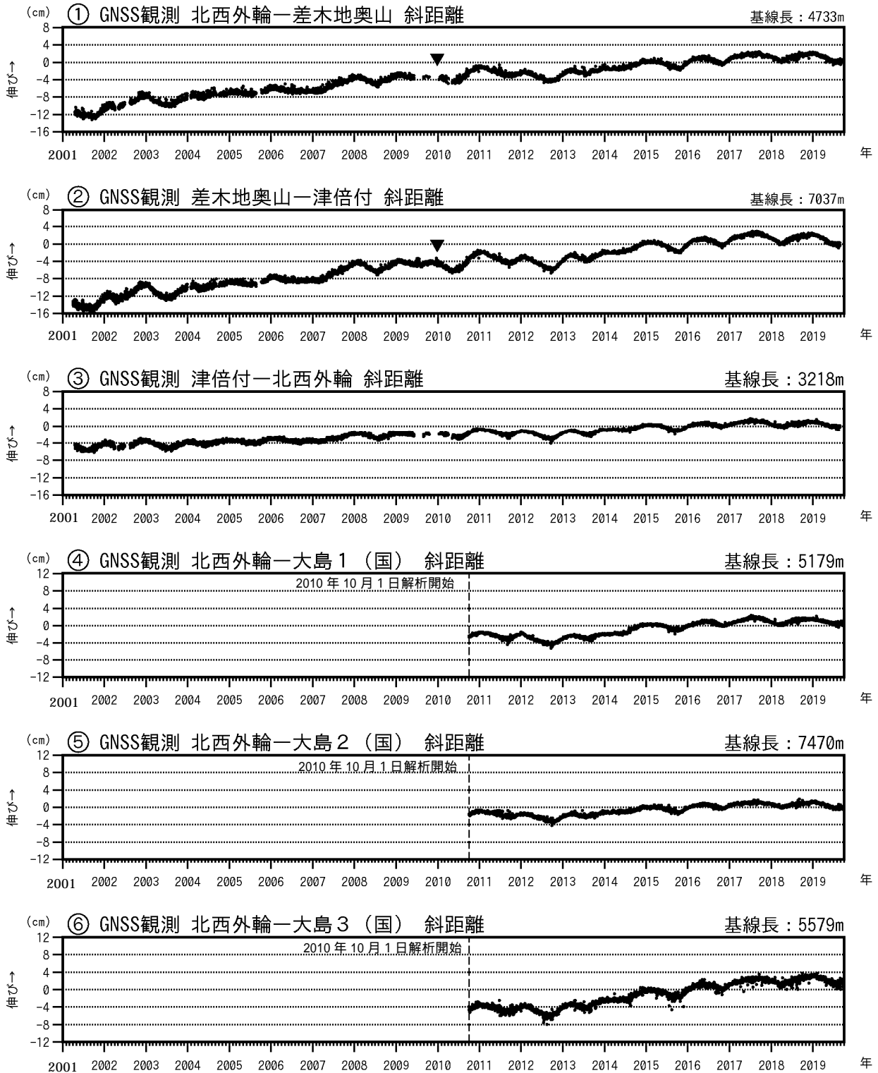
図 3 - 1 伊豆大島 GNSS 連続観測による基線長変化(2001 年 1 月 ~ 2019 年 9 月 30 日)
