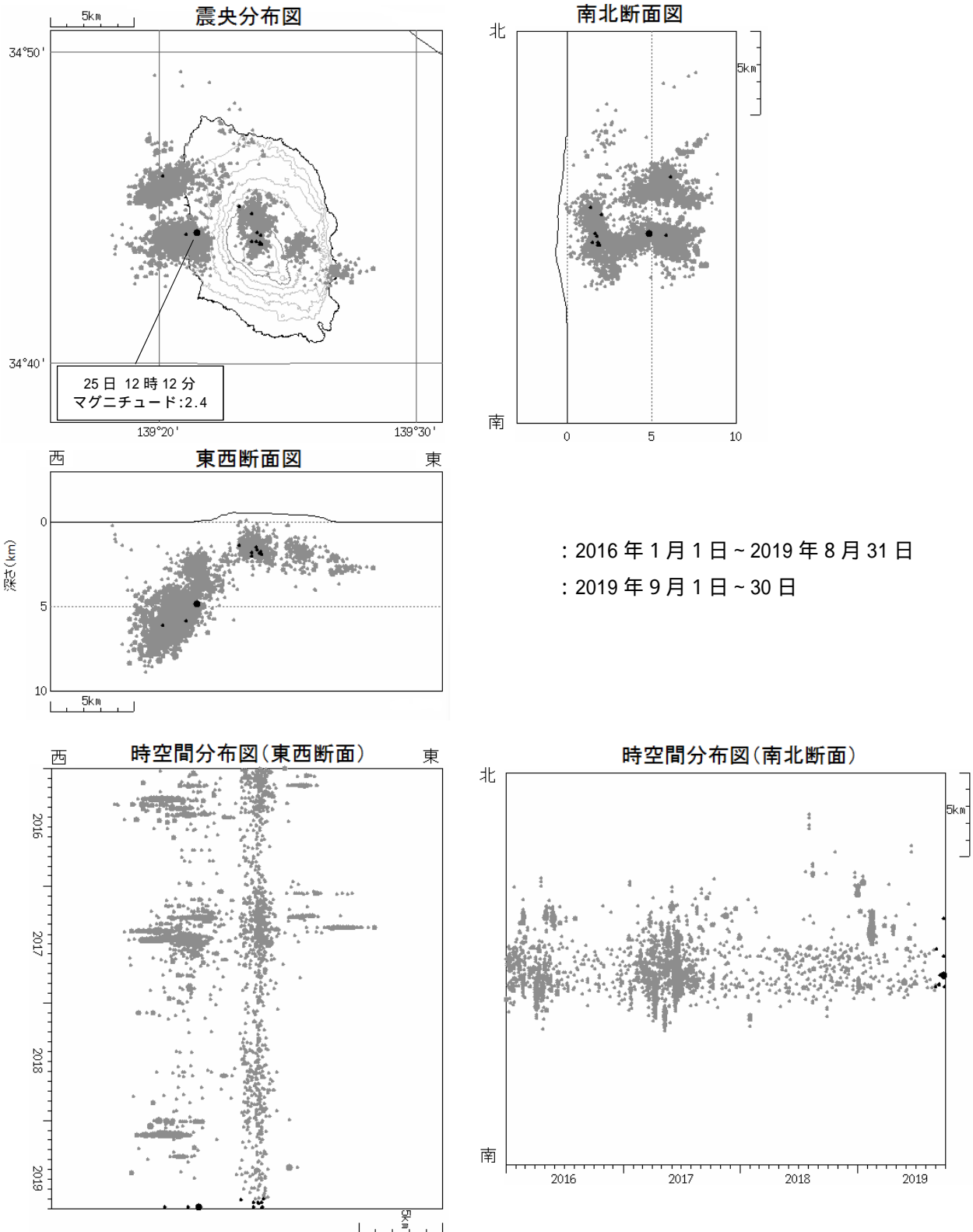
図4 伊豆大島 震源分布図（2016年1月1日～2019年9月30日）
