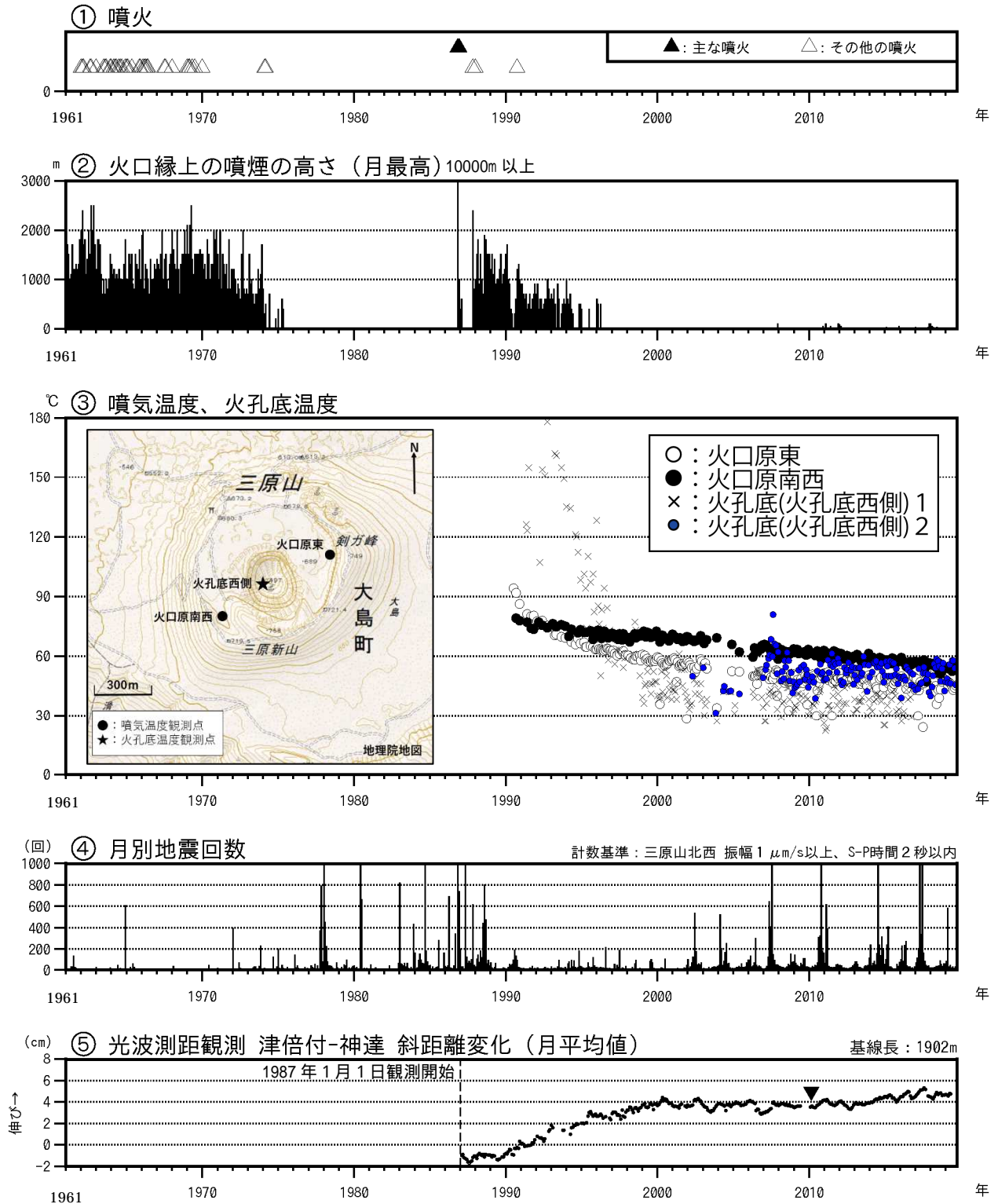
図1 伊豆大島 長期間の火山活動経過図（1961年1月～2019年9月30日） 1991年12月18日までは火口縁上130m以上、2002年2月28日までは火口縁上300m以上の噴煙の高さを観測していました。 火口原東、火口原南西：サーミスタ温度計により直接測定した噴気温度。 火孔底(火孔底西側)1：赤外放射温度計により離れた場所から測定した火孔底温度。 火孔底(火孔底西側)2：赤外熱映像装置により離れた場所から測定した火孔底温度。 地震回数には伊豆大島周辺海域で発生した地震も一部含まれています。 グラフの空白部分は欠測、 は機器更新。
