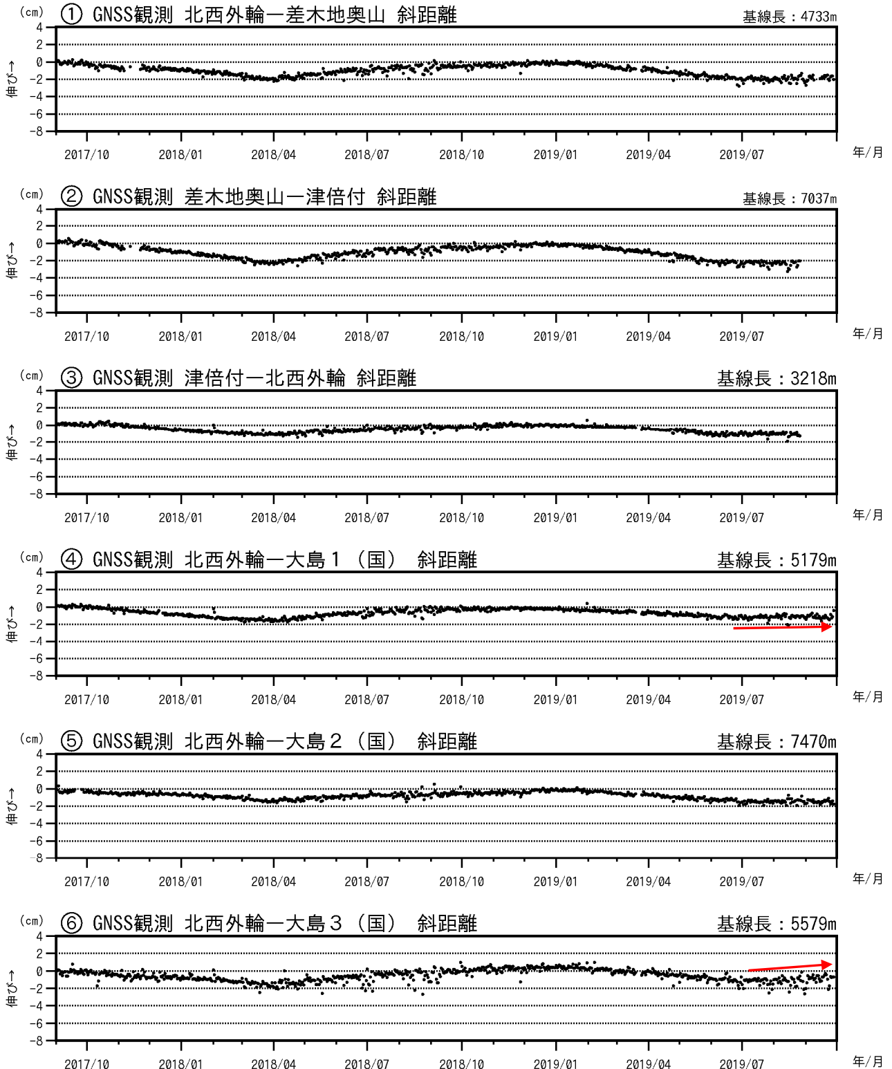
図3-2 伊豆大島 GNSS連続観測による基線長変化(2017年8月~2019年9月30日)
