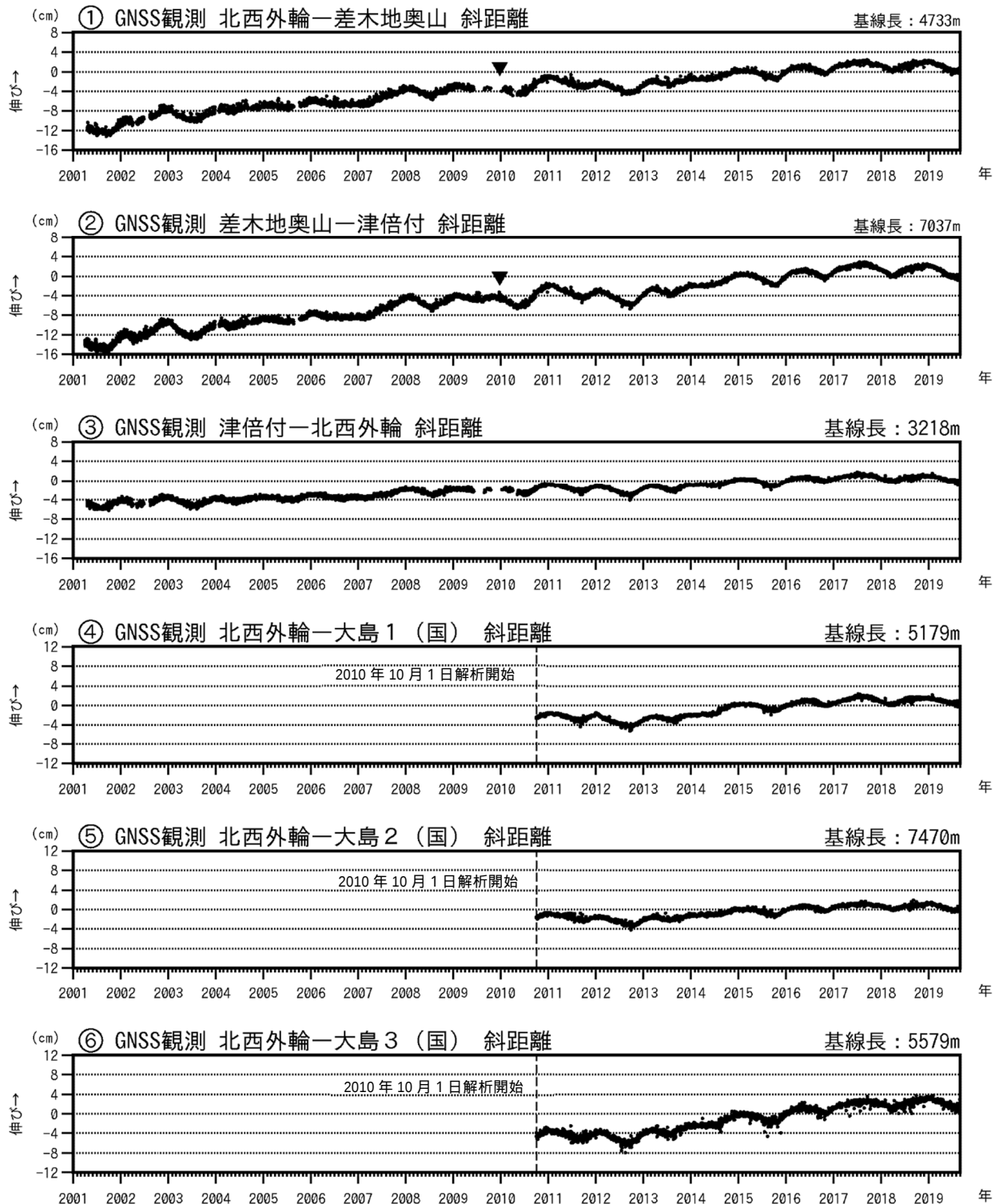
図 3 - 1 伊豆大島 GNSS 連続観測による基線長変化(2001 年 1 月～2019 年 8 月 31 日)
