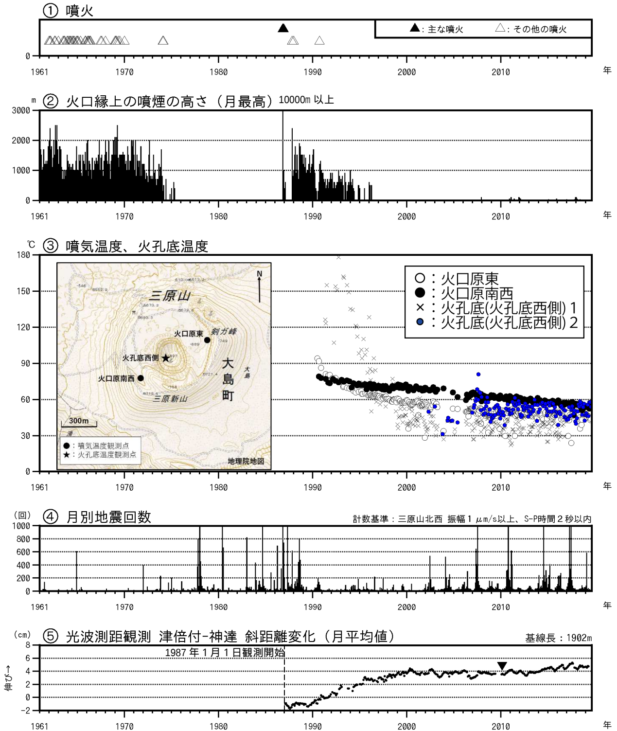
図 1 伊豆大島 長期間の火山活動経過図（1961 年 1 月～2019 年 8 月 31 日）
