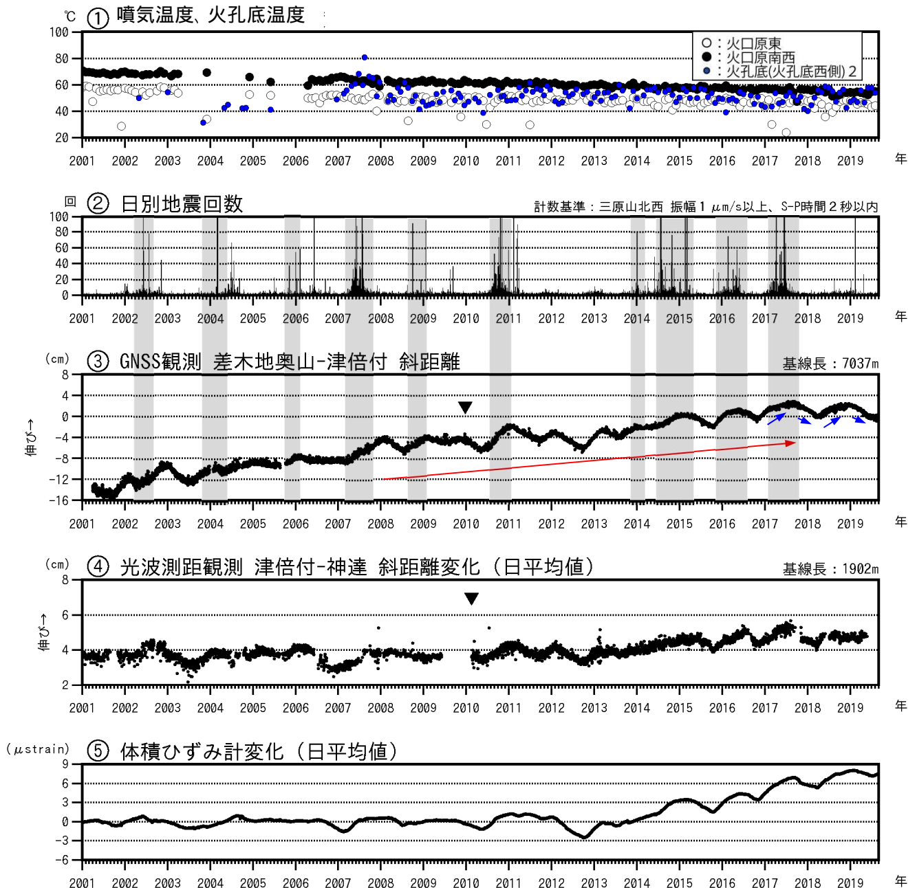
図2 伊豆大島 最近の火山活動経過図（2001年1月～2019年8月31日）
