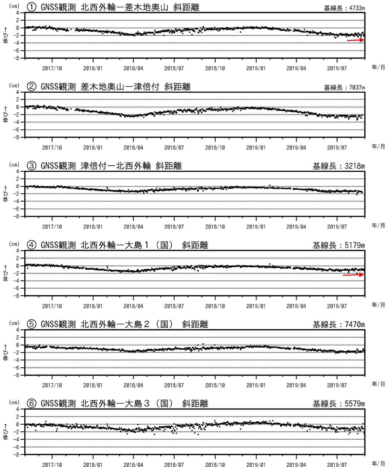
図 3 - 2 伊豆大島 GNSS 連続観測による基線長変化(2017 年 8 月～2019 年 8 月 31 日)
