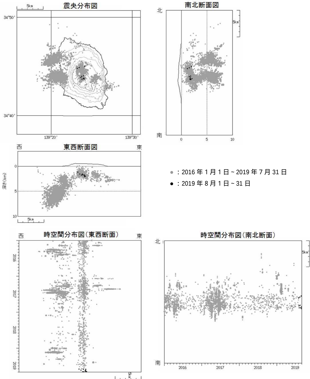
図 4 伊豆大島 震源分布図（2016 年 1 月 1 日～2019 年 8 月 31 日） ・長期的には、地震活動は活発な時期と静穏な時期を繰り返しています。 ・今期間、震源は三原山付近の深さ 1 ～ 2 km 付近に分布しました。
