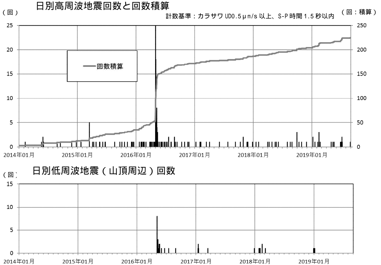
図6 新潟焼山 日別地震回数（2014年1月1日～2019年8月31日）
