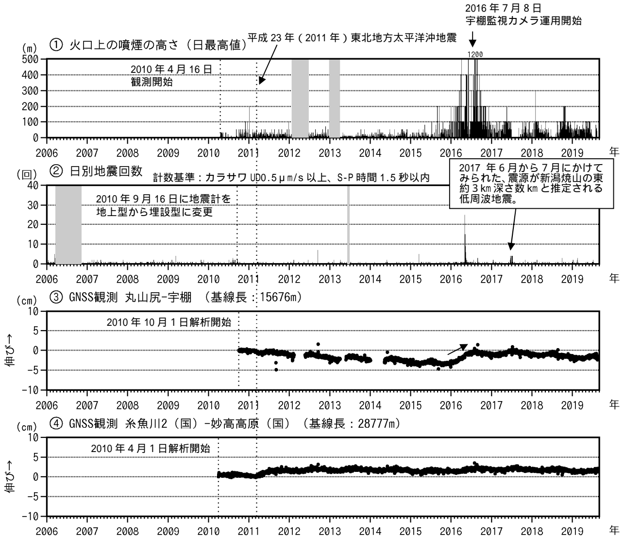
図3 新潟焼山 火山活動経過図（2006年1月1日～2019年8月31日）
