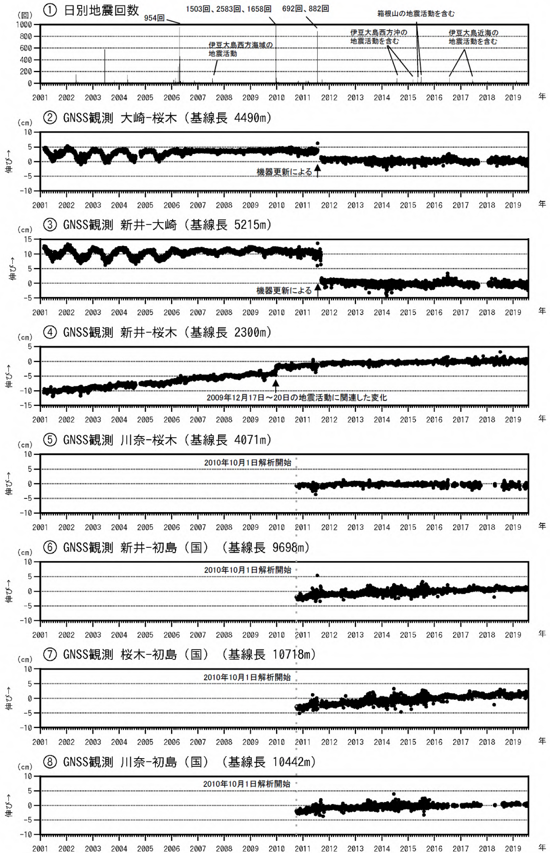
図3 伊豆東部火山群 火山活動経過図（2001年1月1日～2019年7月31日）
