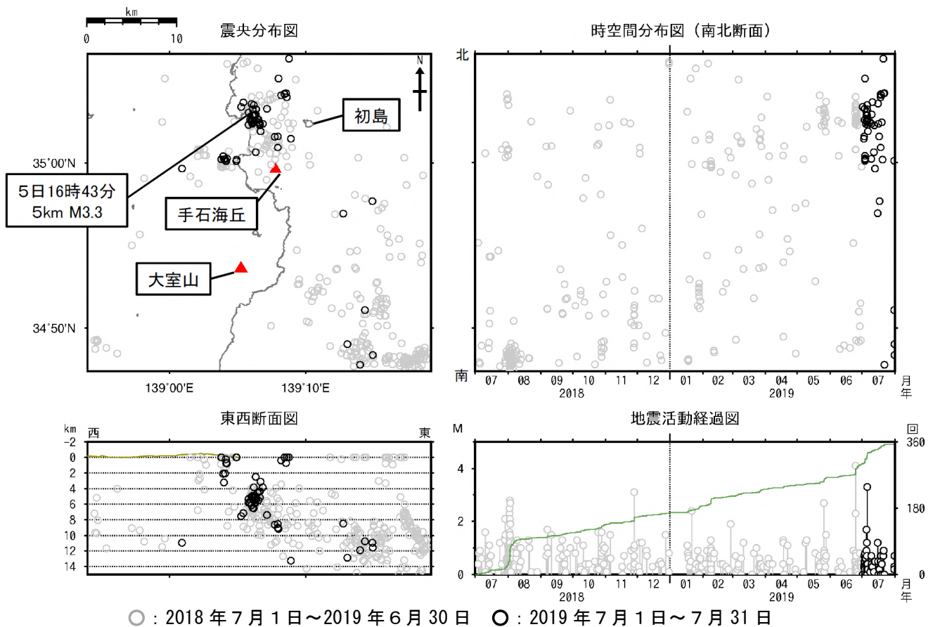
図2 伊豆東部火山群 広域地震観測網による震源分布図（2018年7月1日～2019年7月31日）
