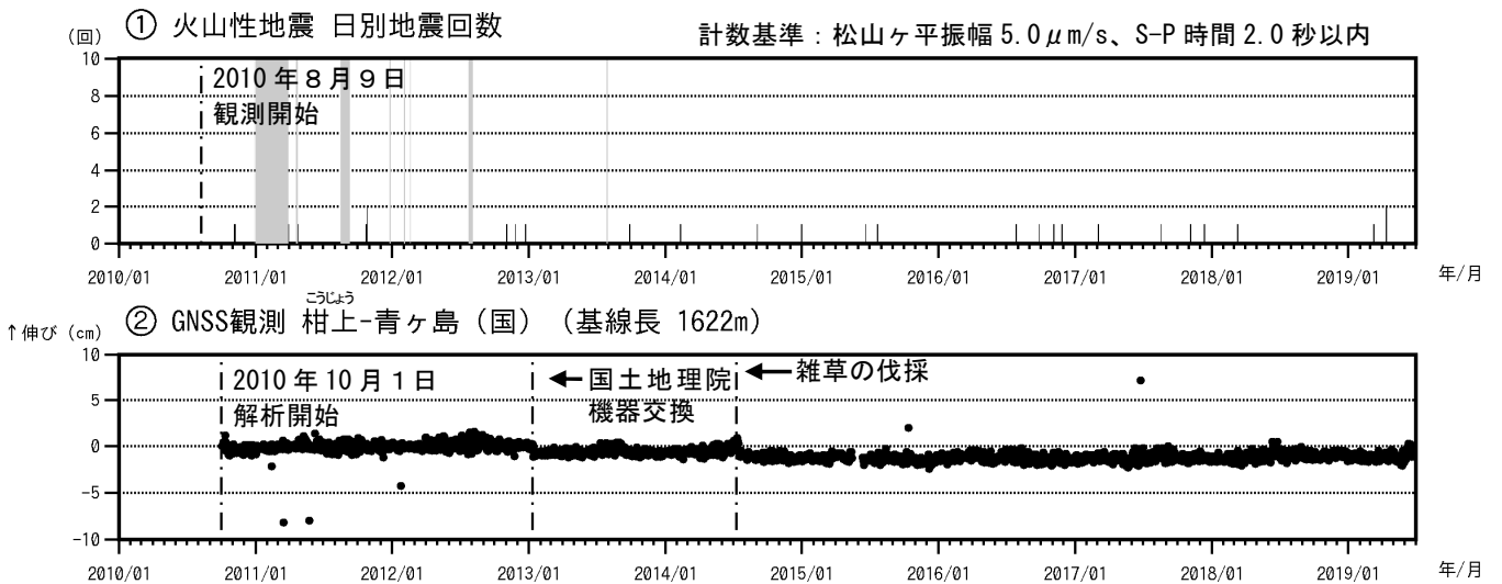
図3 青ヶ島 火山活動経過図（2010年8月9日～2019年6月30日）
