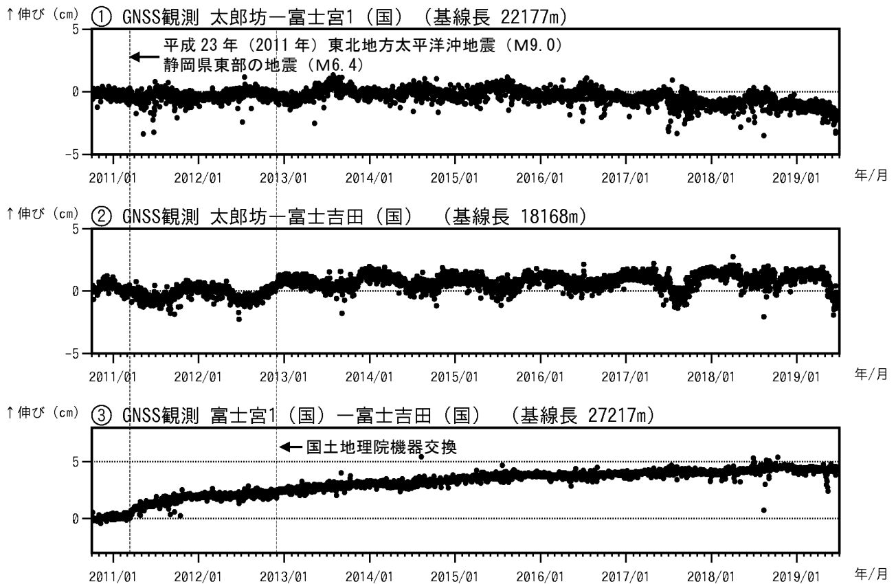
図4 富士山 GNSS 連続観測による基線長変化 (2010 年 10 月 1 日～2019 年 6 月 30 日)
