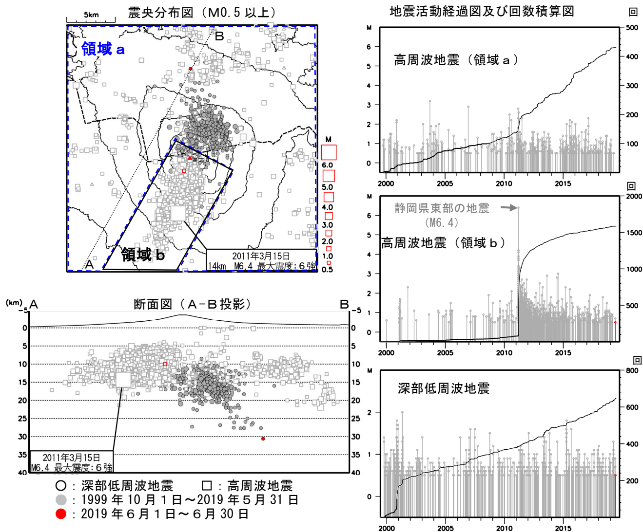
図3 富士山 広域地震観測網による山体及び周辺の地震活動（1999年10月1日～2019年6月30日）
