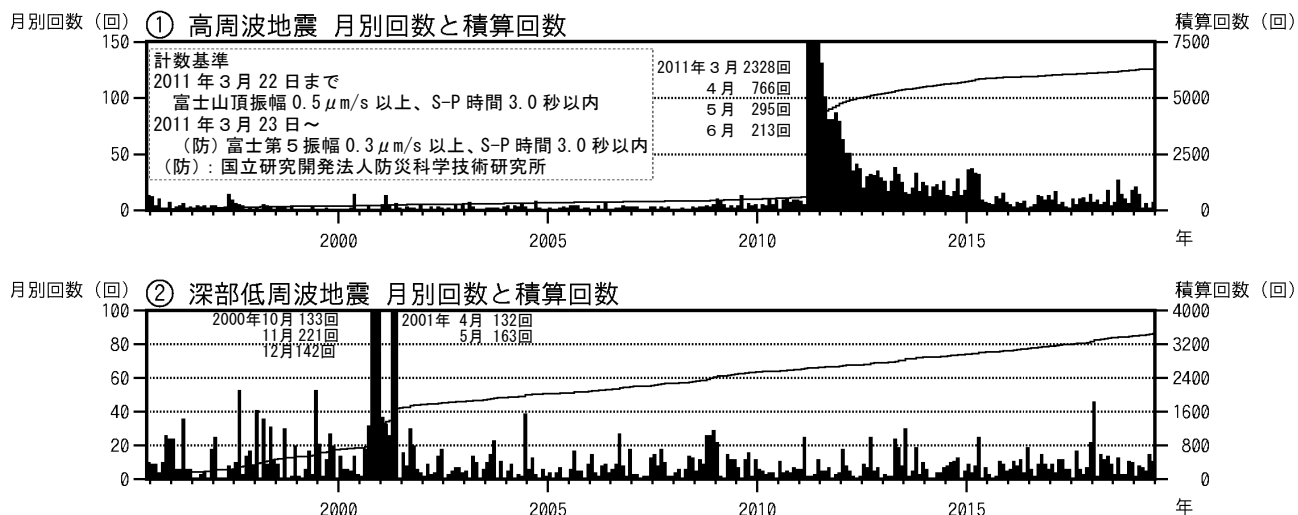
図2 富士山 月別地震回数（1995年6月1日～2019年6月30日）
