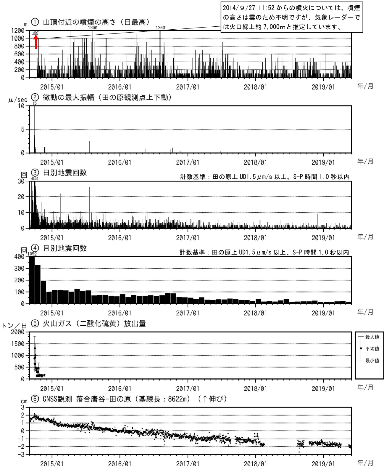
図4 御嶽山 最近の火山活動経過図（2014年9月1日～2019年5月31日）
