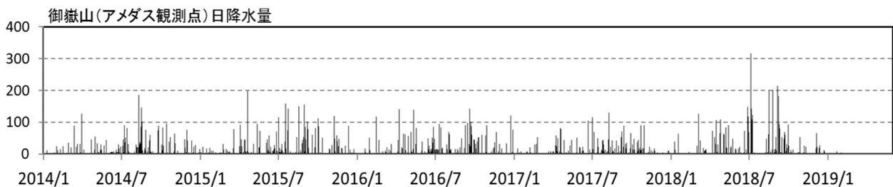
図7 御嶽山 田の原観測点の傾斜変動（2014年1月1日～2019年5月31日）
