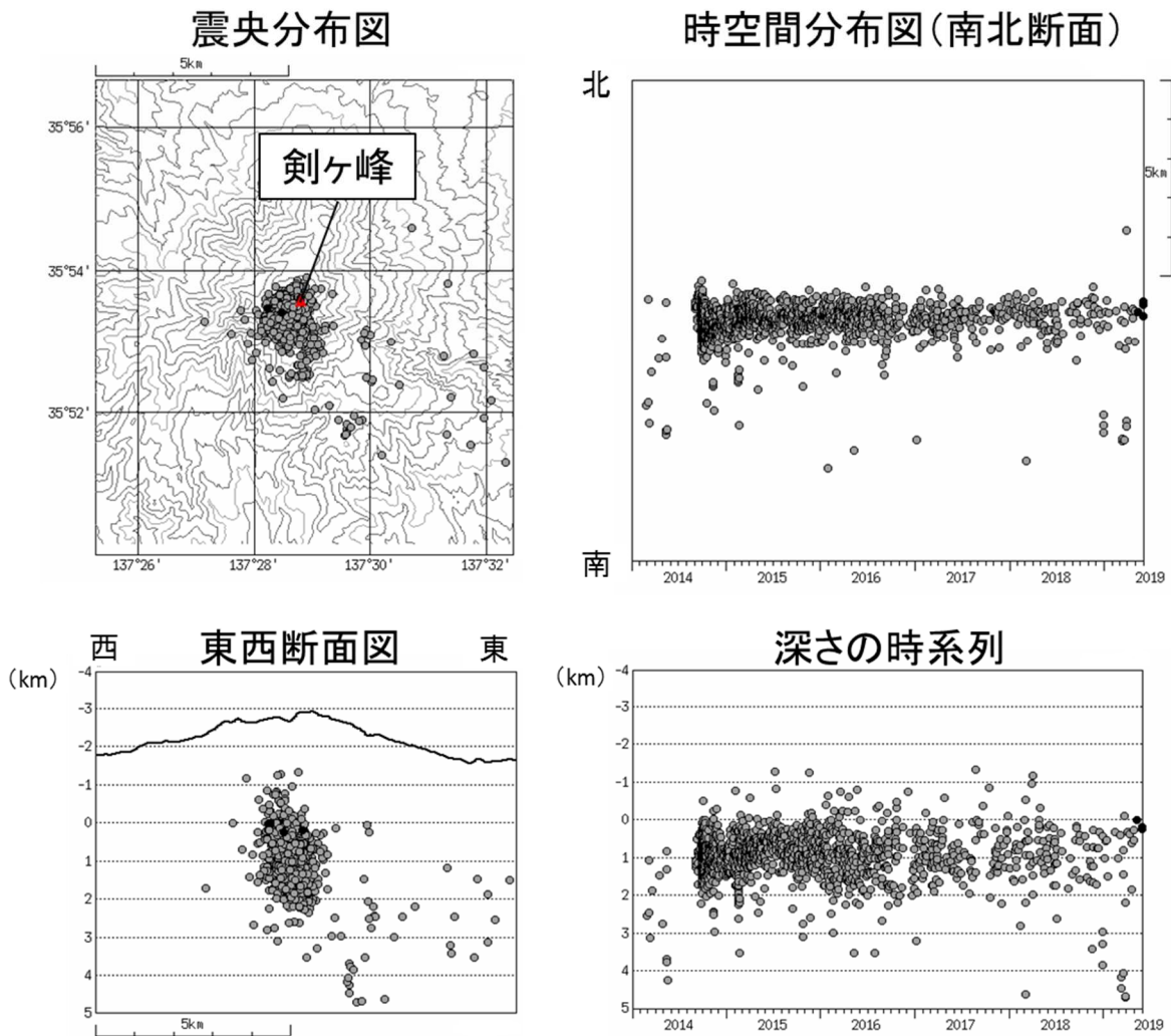
図2 御嶽山 震源分布図（2014年1月1日～2019年5月31日）
