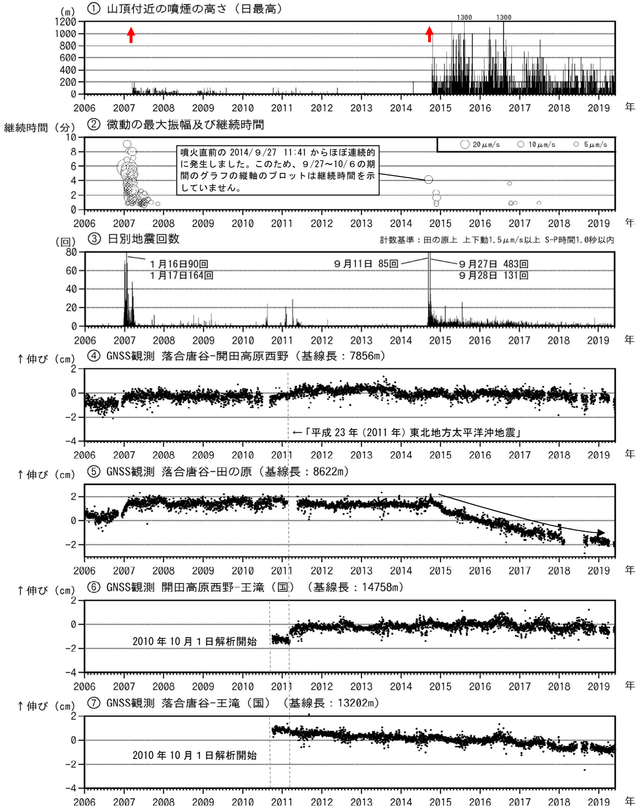
図5 御嶽山 長期間の火山活動経過図（2006年1月1日～2019年5月31日）
