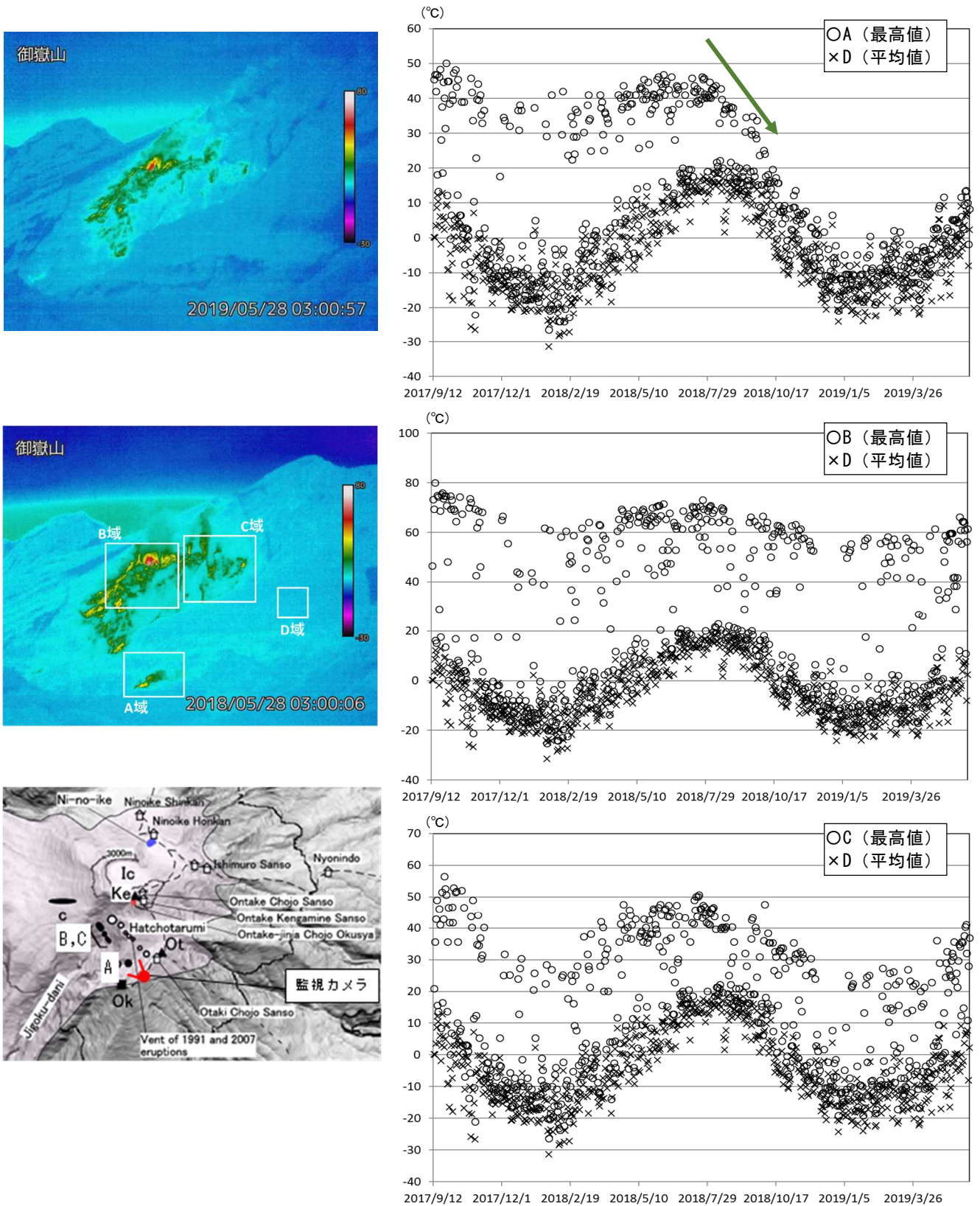
図3 御嶽山 奥の院赤外熱映像カメラによる剣ヶ峰南西側における最高温度の推移
