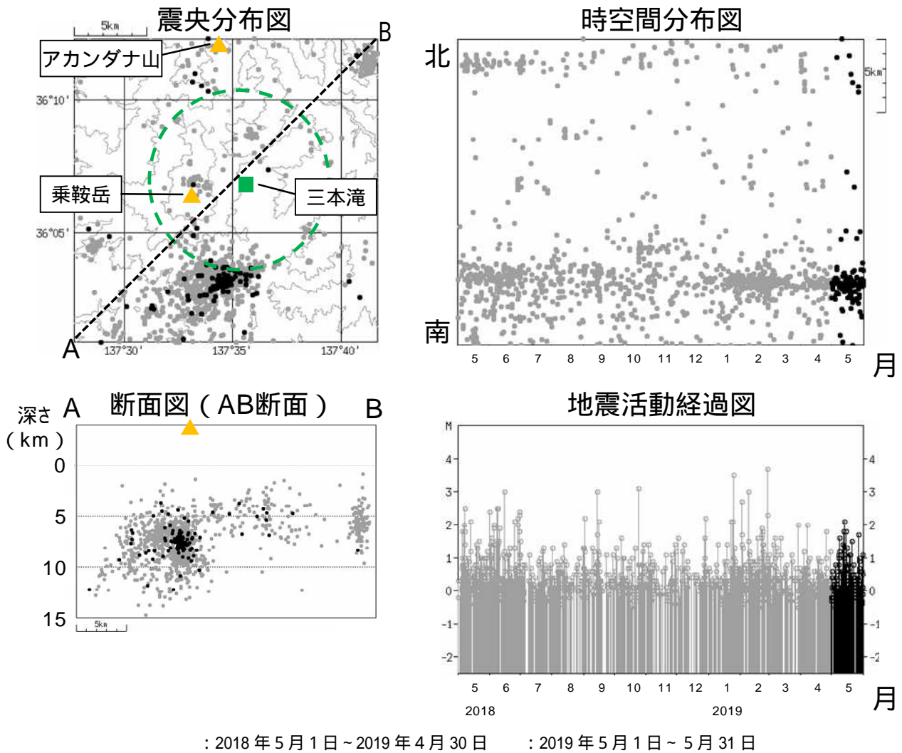
図3 乗鞍岳 広域地震観測網による山体・周辺の地震活動(2018年5月1日～2019年5月31日) 広域地震観測網により震源決定したもので、深さは全て海面以下として決定しています。M（マグニチュード）は地震の規模を表します。図中の震源要素は一部暫定値が含まれており、後日変更することがあります。 震央分布図中の緑点線円は、図2 で計数される地震のおおよその範囲を示します。 ・乗鞍岳付近の地震活動は、低調に経過しています。 ・乗鞍岳から南方へ約6 km離れたところでまとまった地震活動がみられますが、乗鞍岳の火山活動とは関係ないとみています。
