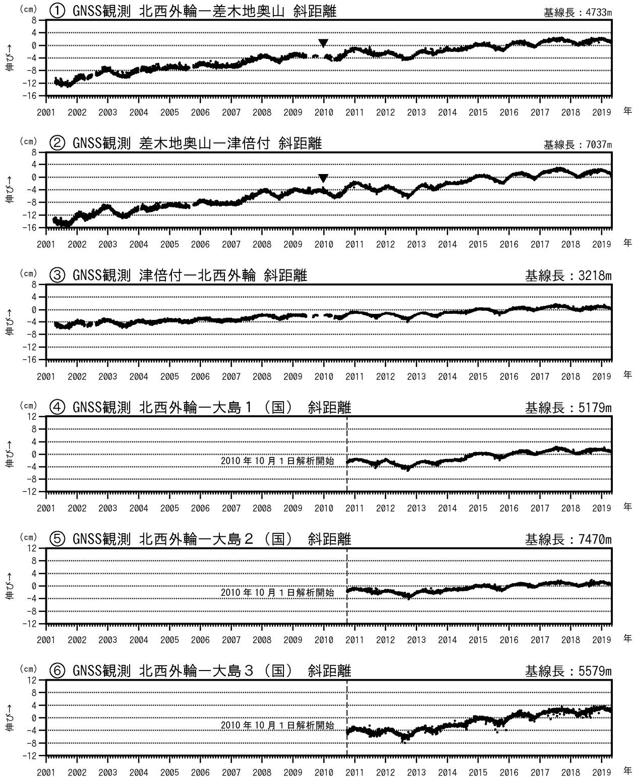
図3 伊豆大島 GNSS 連続観測による基線長変化 (2001 年 1 月～2019 年 4 月 30 日)
