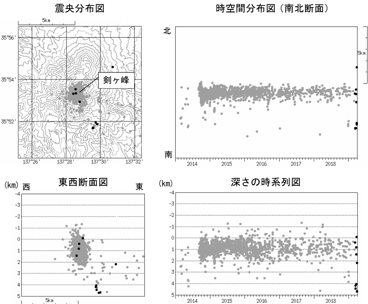
図 2 御嶽山 震源分布図（2014 年 1 月 1 日～2019 年 3 月 31 日）
