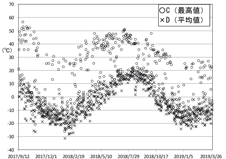
図3 御嶽山 奥の院赤外熱映像カメラによる剣ヶ峰南西側における最高温度の推移（2017年9月13日～2019年3月31日）と同カメラの位置（Oikawa et al., 2016 に加筆）
