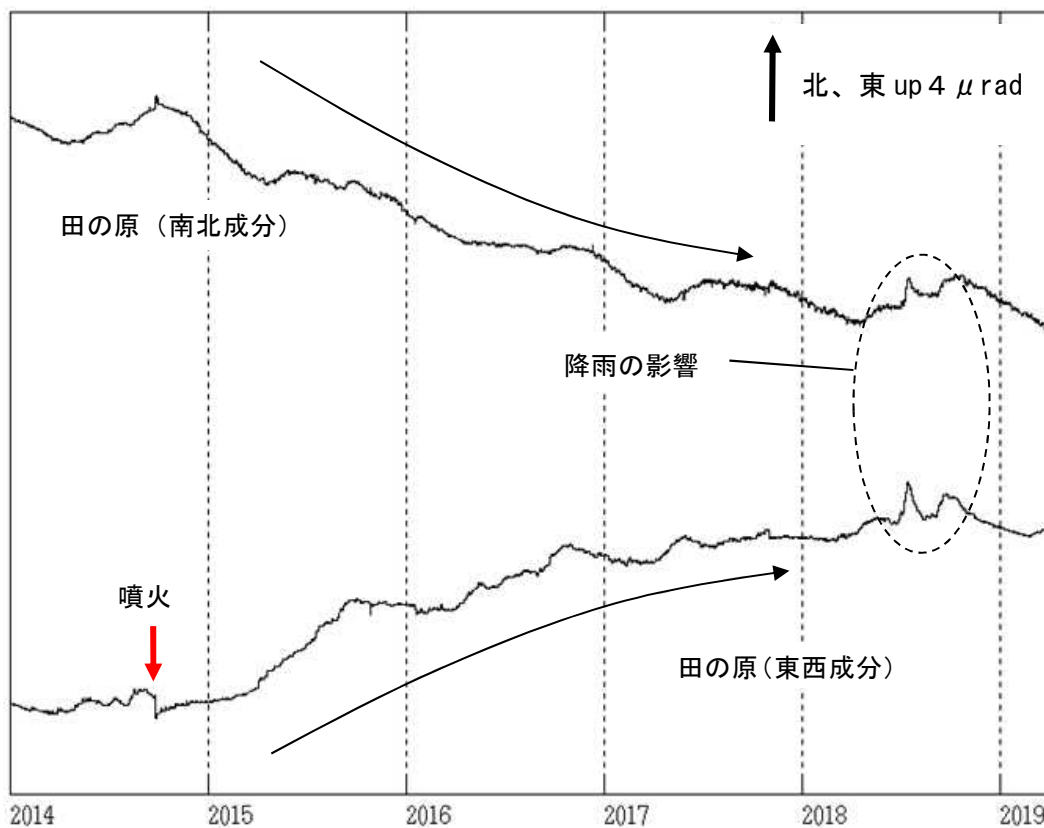
図 7 御嶽山 田の原観測点の傾斜変動（2014 年 1 月 1 日～2019 年 3 月 31 日）
