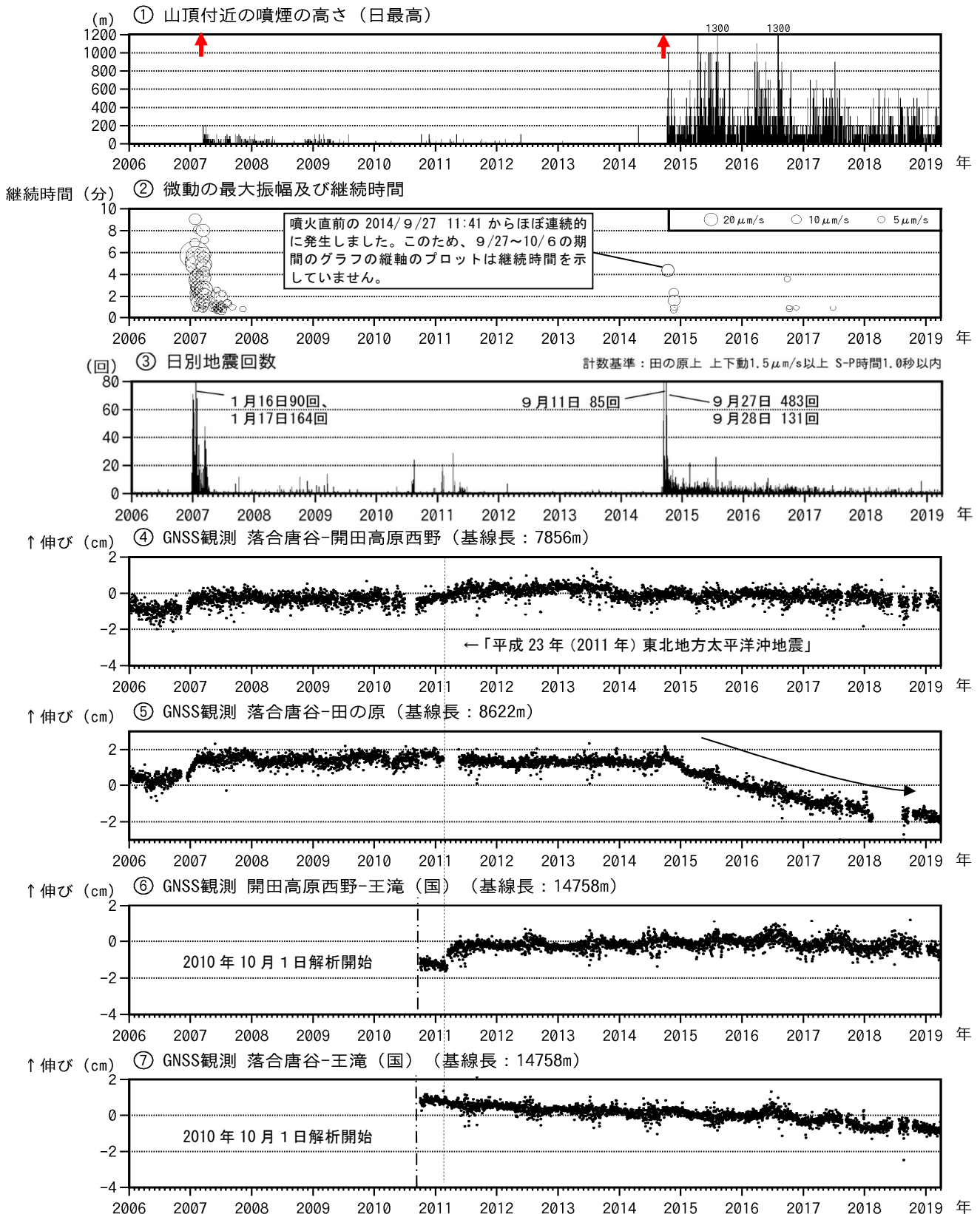
図5 御嶽山 長期間の火山活動経過図（2006年1月1日～2019年3月31日）
