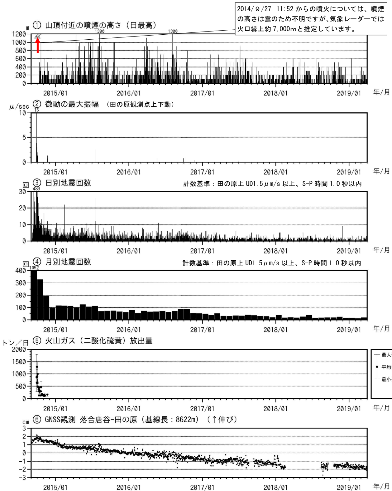
図4 御嶽山 最近の火山活動経過図（2014年9月1日～2019年3月31日）
