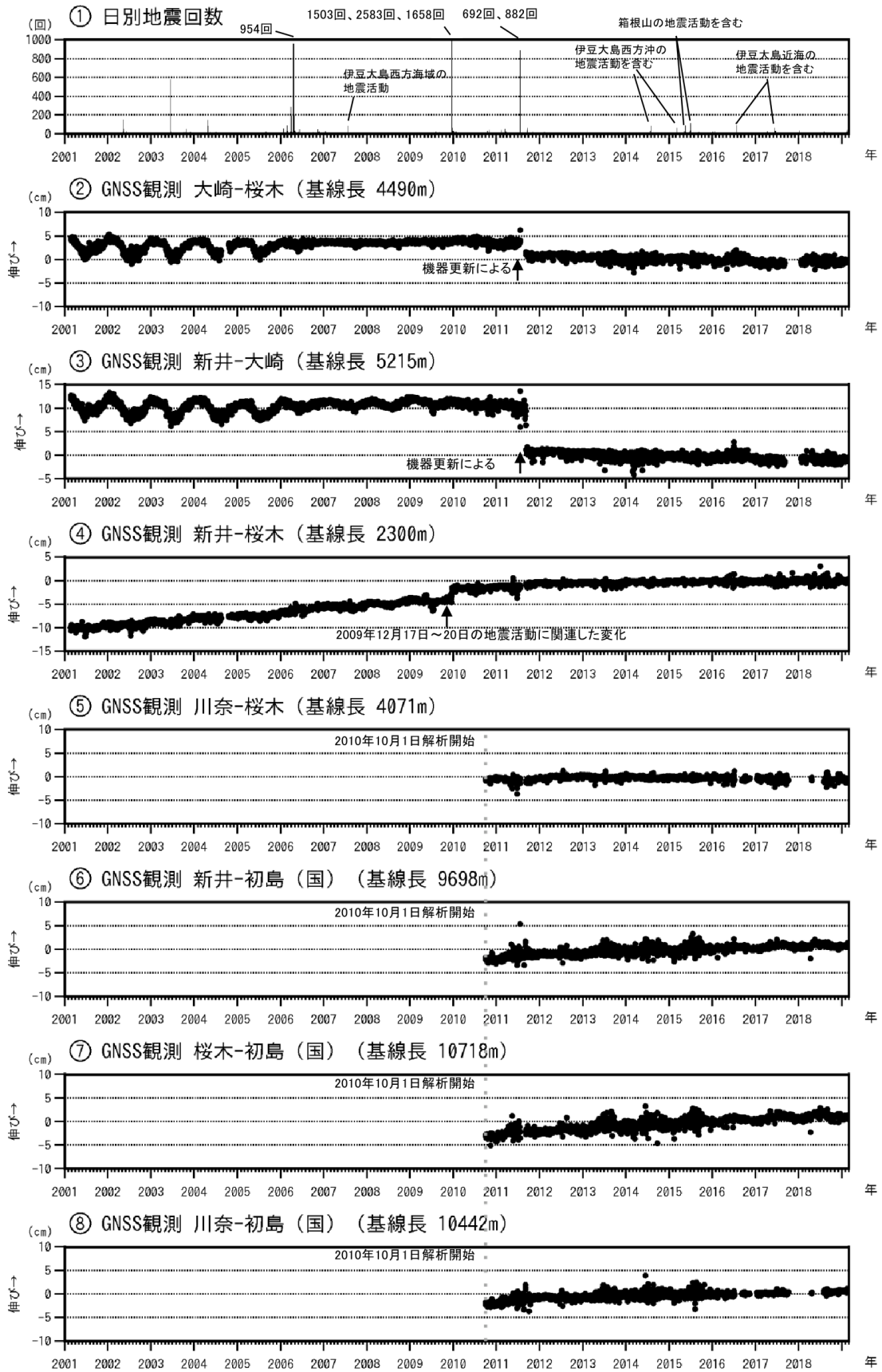
図 3 伊豆東部火山群 火山活動経過図（2001 年 1 月 1 日～2019 年 2 月 28 日）
