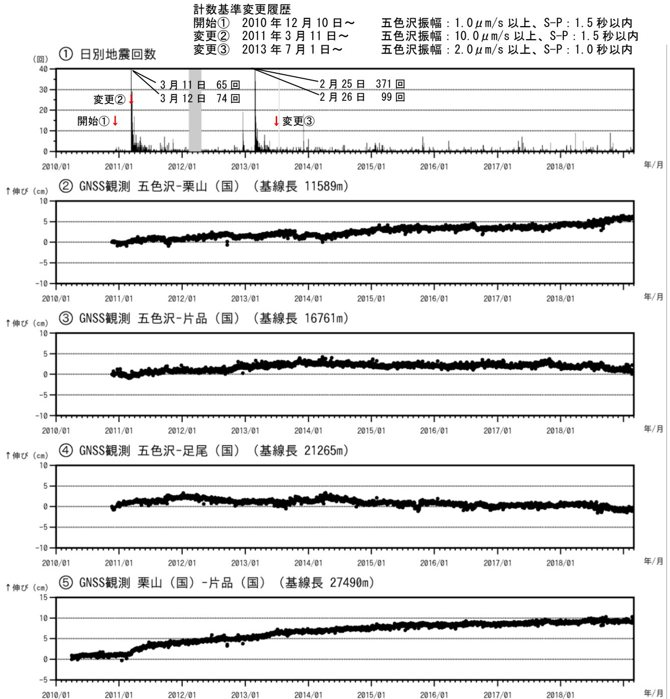
図2 日光白根山 火山活動経過図（2010 年 11 月 20 日～2019 年 2 月 28 日）
