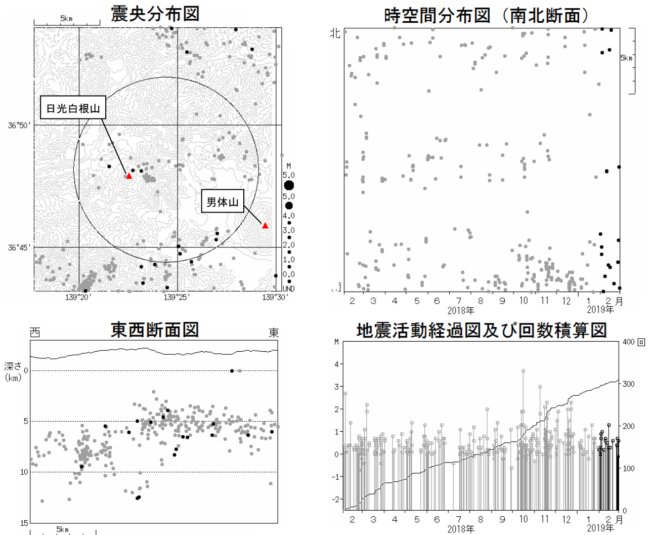
図 3 日光白根山 広域地震観測網による山体・周辺の地震活動 (2018 年 2 月 1 日～2019 年 2 月 28 日)
