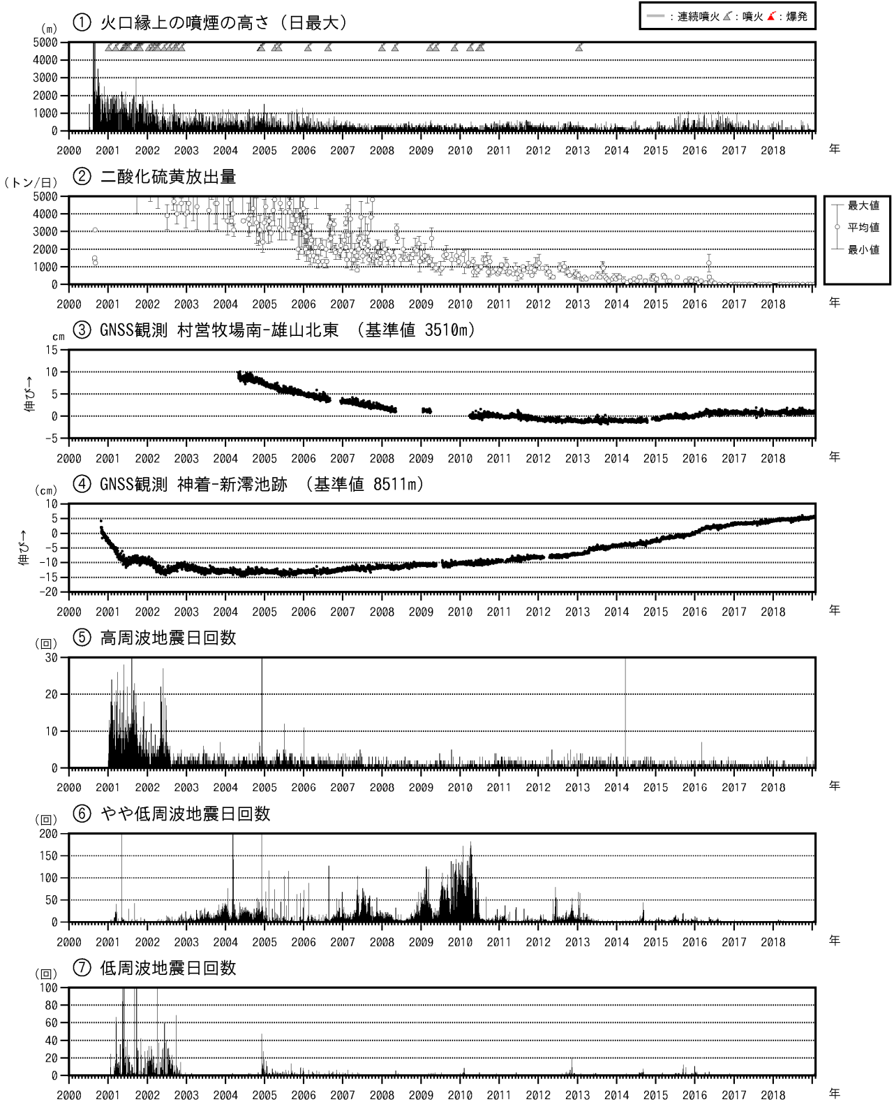
図5 三宅島 火山活動長期経過図（2000年1月1日～2019年1月31日）
