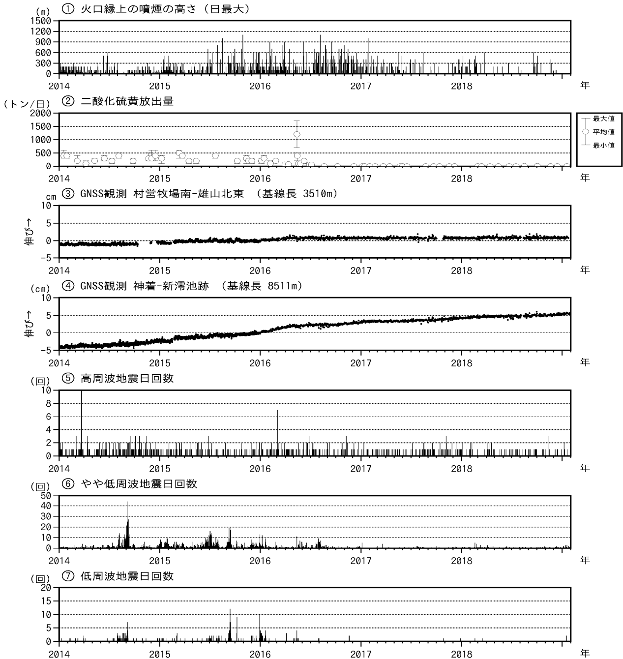
図6 三宅島 火山活動短期経過図(2014年1月1日~2019年1月31日)
