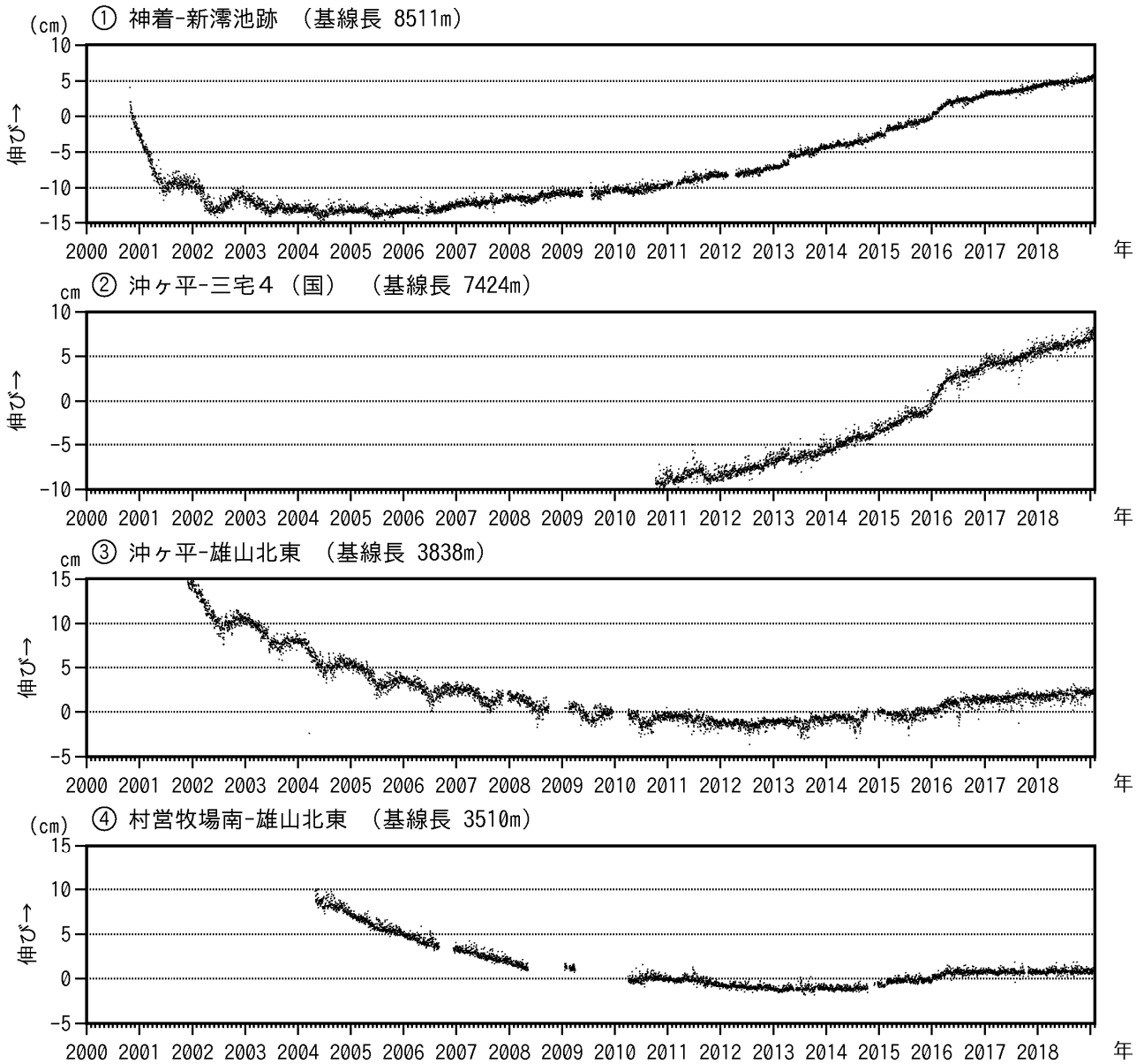
図7 三宅島 GNSS 連続観測結果 (2000年10月26日~2019年1月31日)
