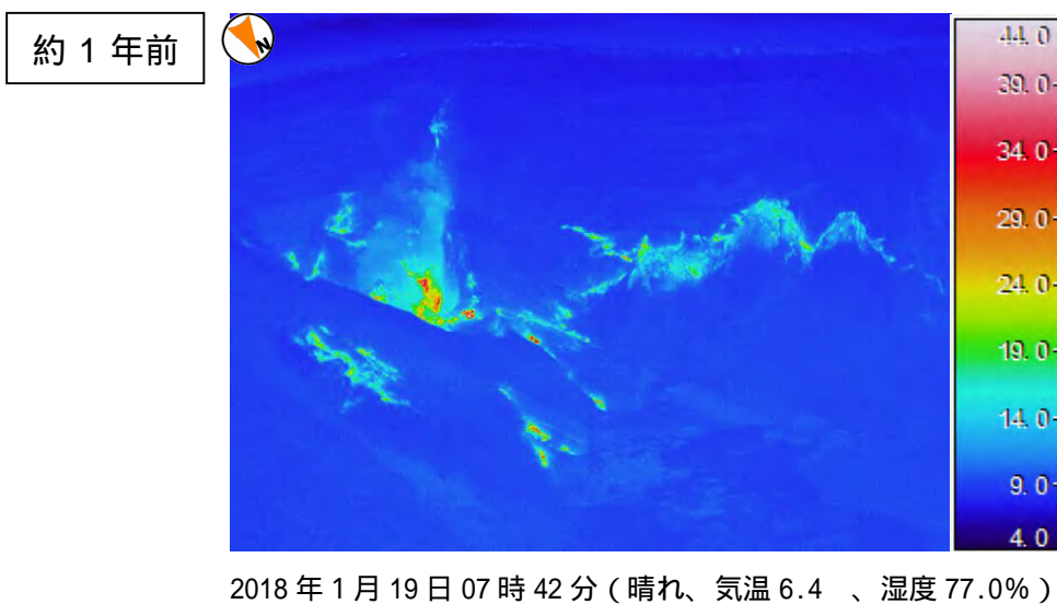
図4 三宅島 赤外熱映像装置による山頂火口内の地表面温度分布 10日に実施した現地調査では、2018年12月や昨年と同様に主火孔内及びその周辺で引き続き高温領域が認められました。高温領域の分布に特段の変化は認められません。
