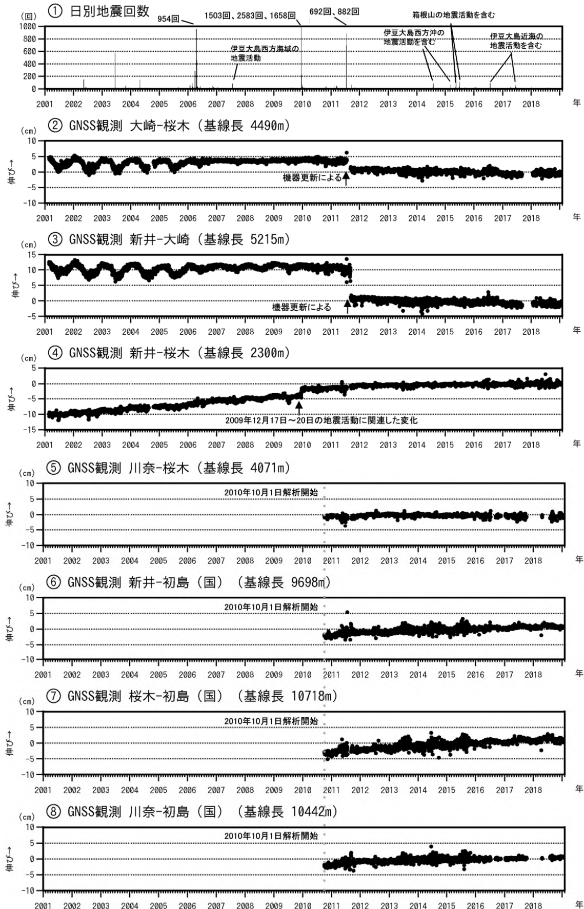
図3 伊豆東部火山群 火山活動経過図(2001年1月1日~2019年1月31日) : 2012年7月23日までは鎌田2、それ以降は鎌田3地震観測点による。 ~ (国): 国土地理院。図4のGNSS基線 ~ に対応。グラフの空白部分は欠測。 2010年10月及び2016年1月以降のデータについては、解析方法を変更しています。 基線長変化に見られる周期的な変動は季節変動と考えられます。
