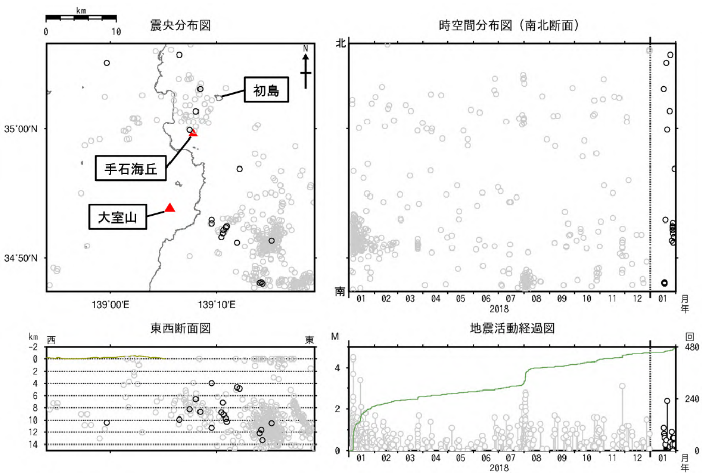
図2 伊豆東部火山群 広域地震観測網による震源分布図(2018年1月1日～2019年1月31日)
