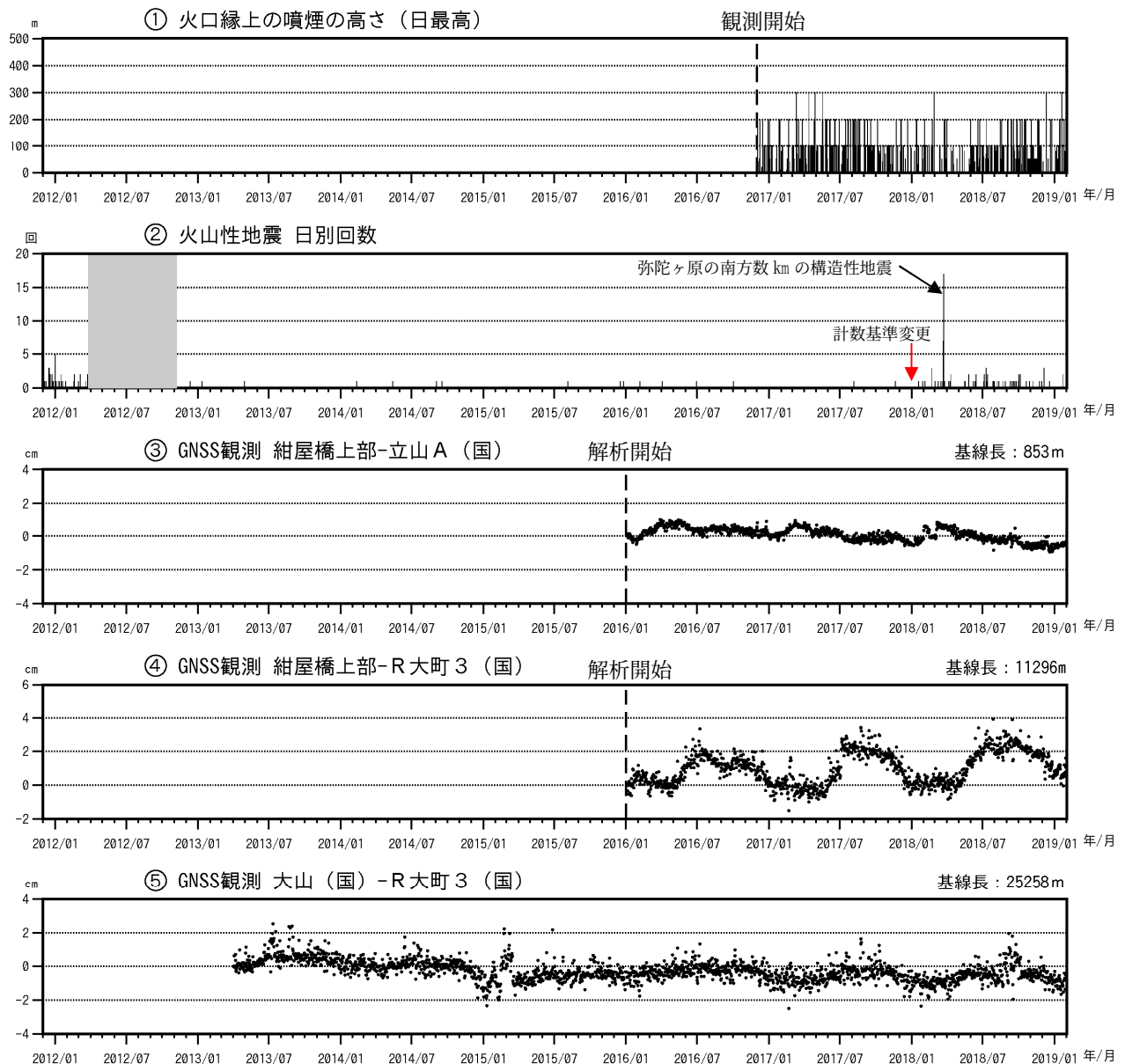
図3 弥陀ヶ原 火山活動経過図（2011 年 12 月 1 日～2019 年 1 月 31 日）
