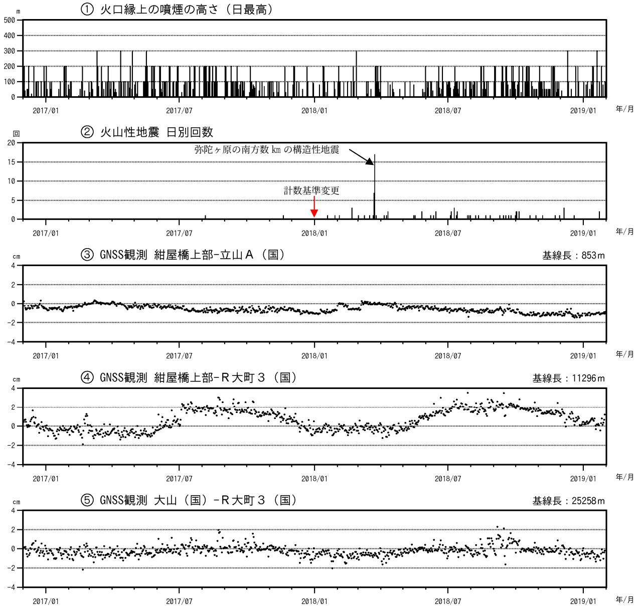
図 4 弥陀ヶ原 最近の火山活動経過図（2016 年 12 月 1 日～2019 年 1 月 31 日）
