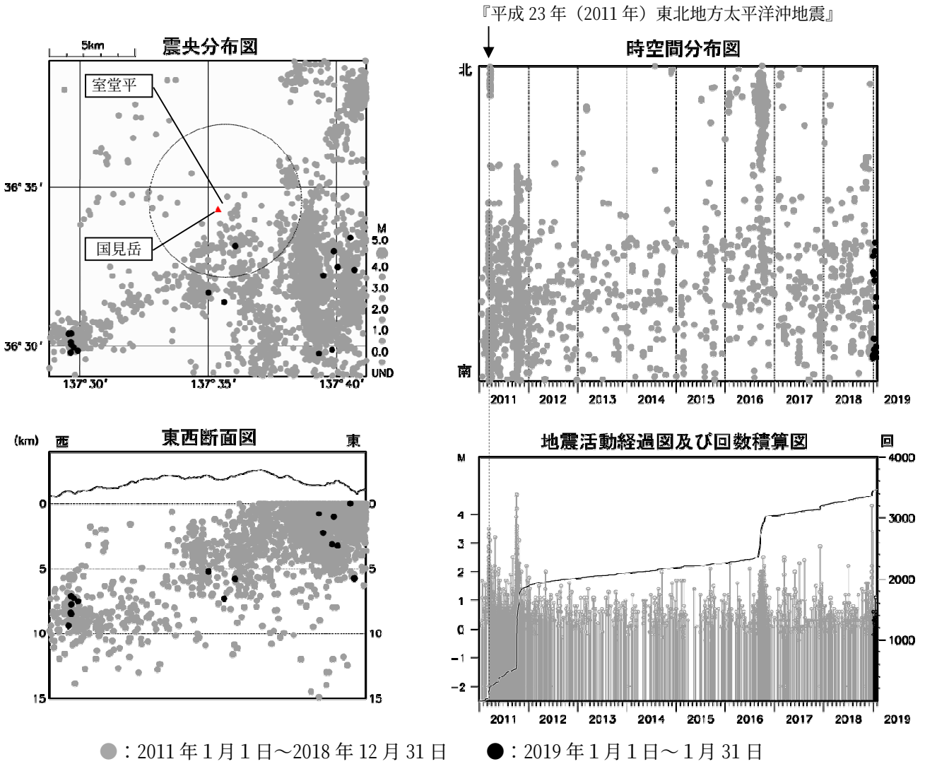
図2 弥陀ヶ原 広域地震観測網による山体・周辺の地震活動（2011 年 1 月 1 日～2019 年 1 月 31 日）
