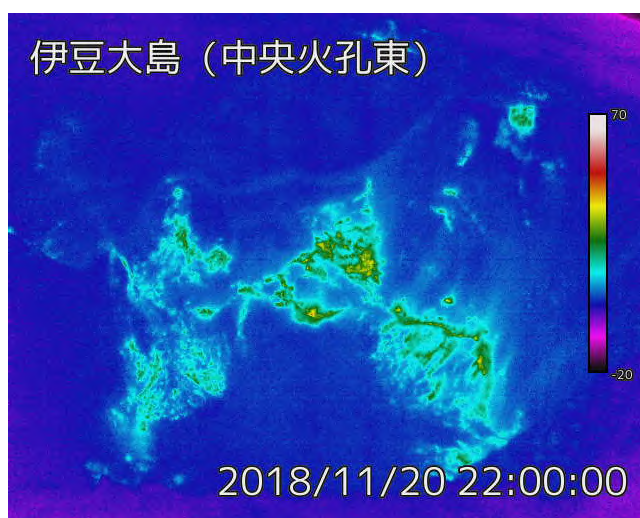
2018 年 11 月 20 日、中央火孔東監視カメラによる
