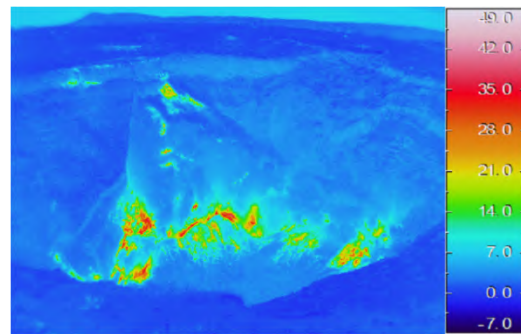
2018 年 12 月 25 日 04 時 53 分 気温：2℃、晴れ
