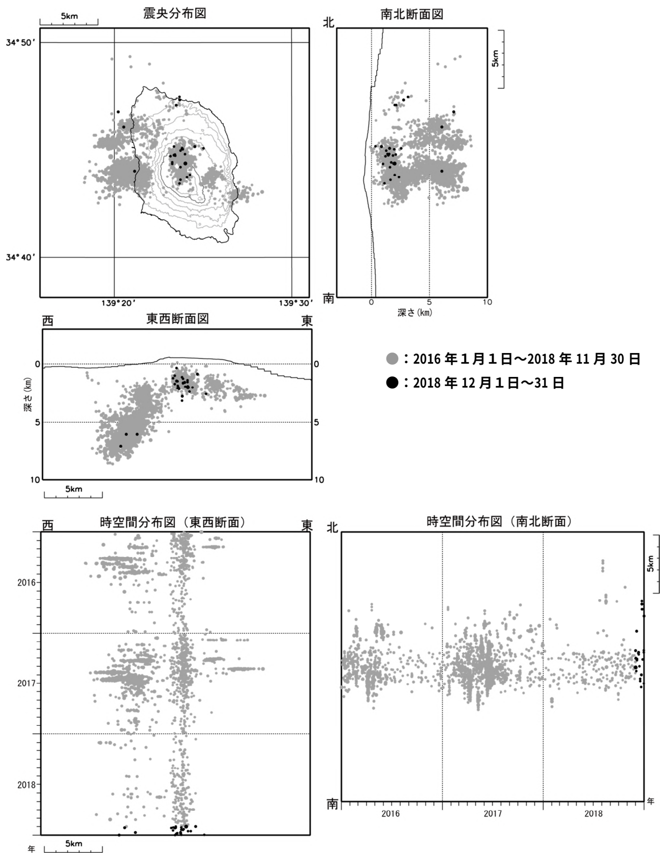
図 4 伊豆大島 震源分布図（2016 年 1 月 1 日～2018 年 12 月 31 日）
