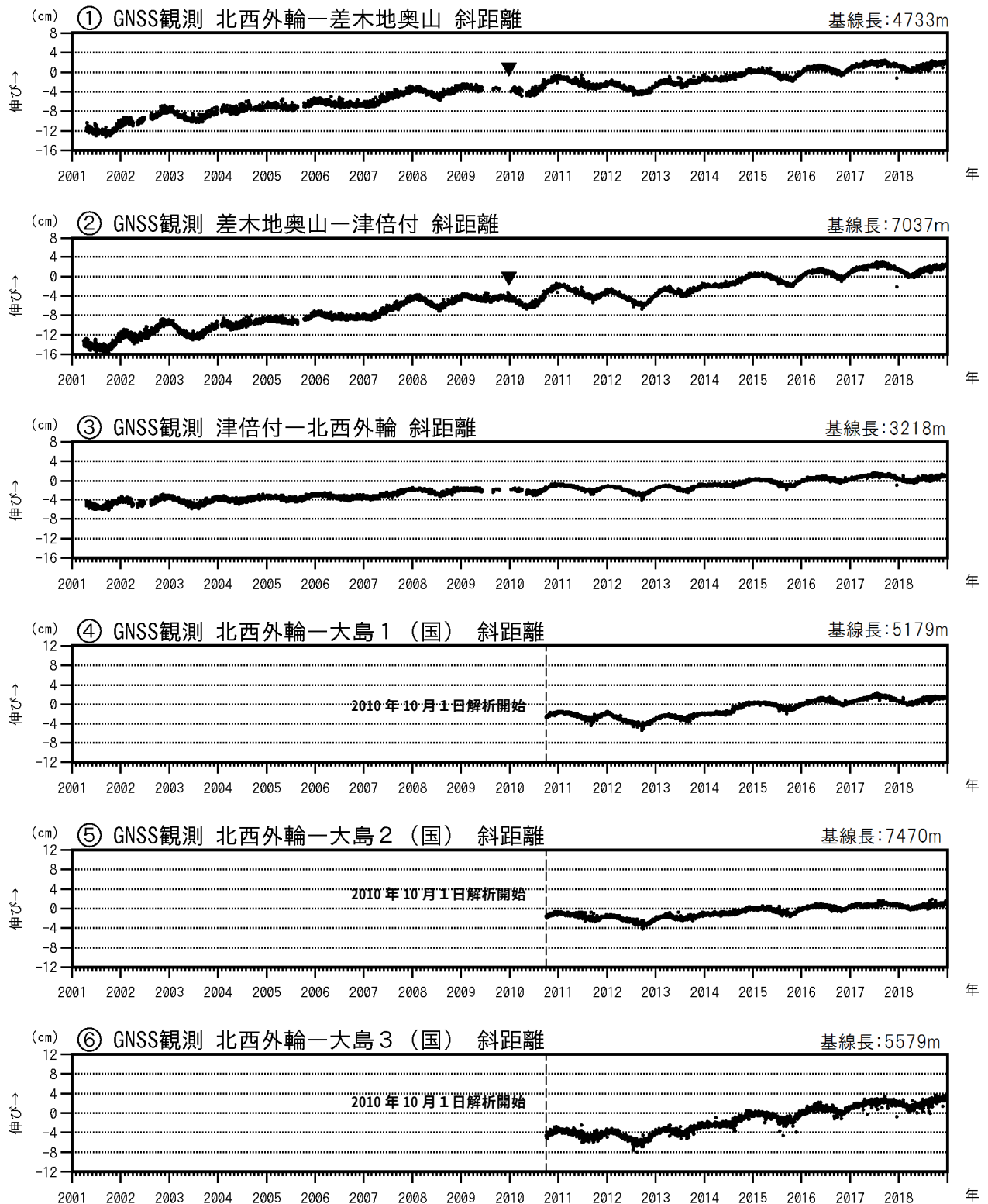
図3 伊豆大島 GNSS 連続観測による基線長変化(2001 年 1 月～2018 年 12 月 31 日)
