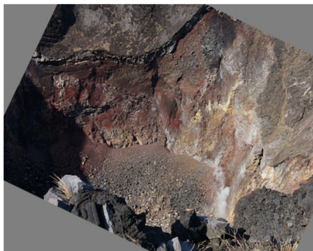
中央火孔東監視カメラの撮影領域（可視）
