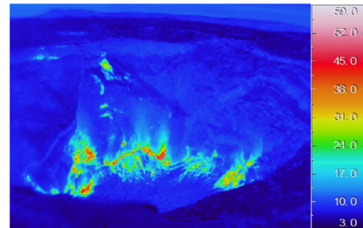
2018 年 11 月 21 日 04 時 57 分 気温：8℃、晴れ
