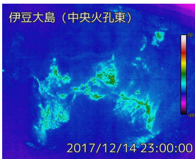
2017 年 12 月 14 日、中央火孔東監視カメラによる
