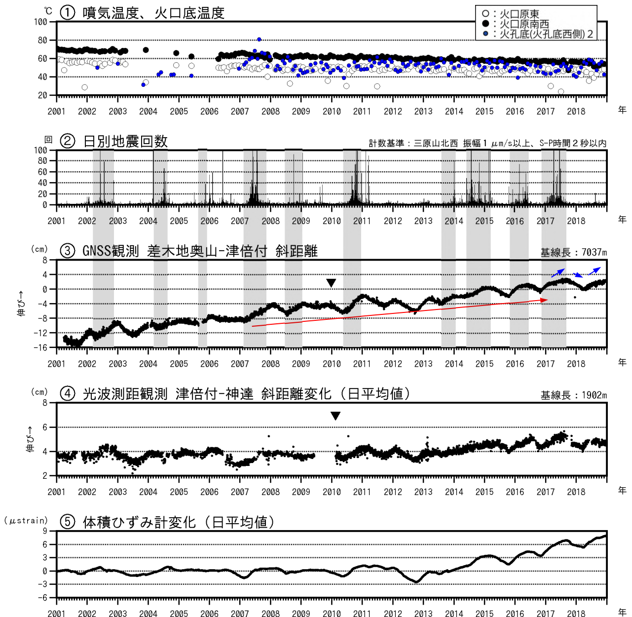
図2 伊豆大島 最近の火山活動経過図（2001年1月～2018年12月31日）
