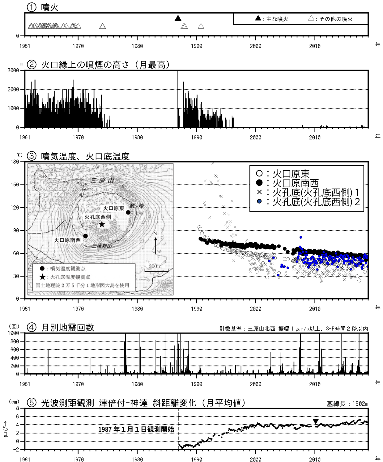
図 1 伊豆大島 長期間の火山活動経過図（1961 年 1 月～2018 年 12 月 31 日）
