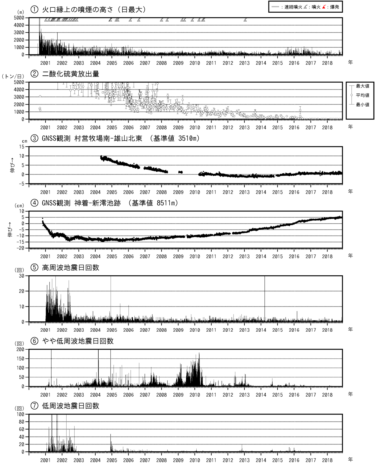
図5 三宅島 火山活動長期経過図（2000年1月1日～2018年11月30日）
