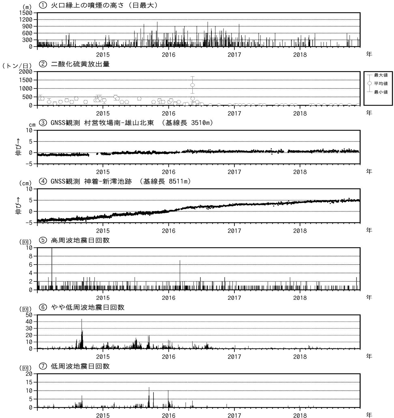
図6 三宅島 火山活動短期経過図(2014年1月1日~2018年11月30日)
