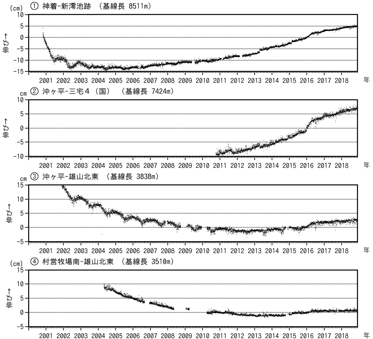
図7 三宅島 GNSS 連続観測結果（2000年10月26日～2018年11月30日）
