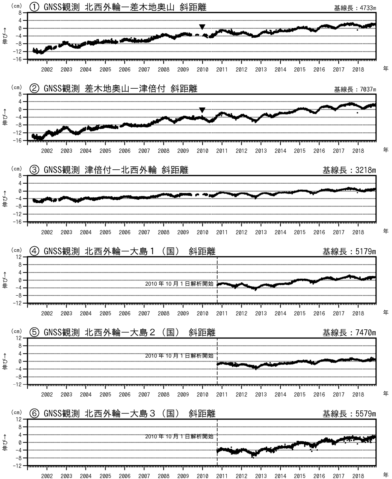
図3 伊豆大島 GNSS 連続観測による基線長変化(2001年1月~2018年11月30日)
