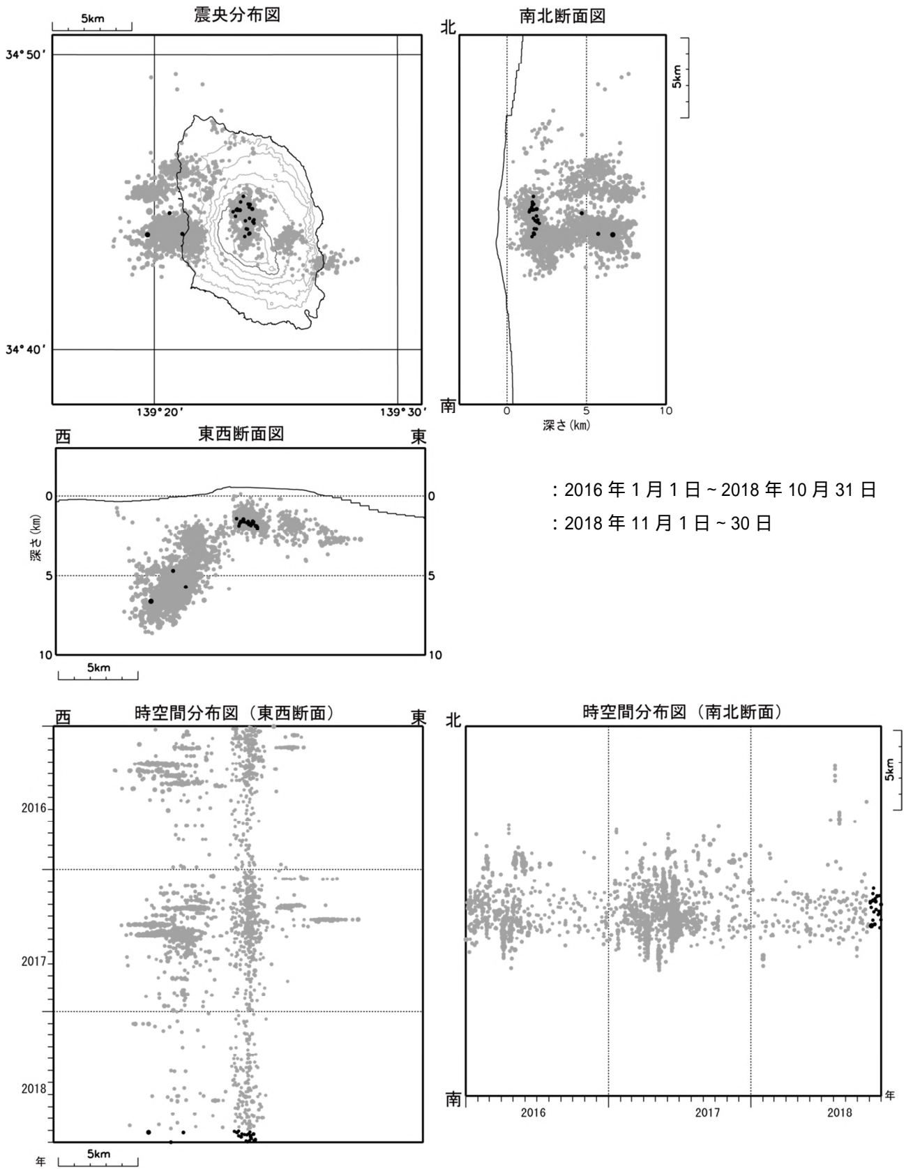
図4 伊豆大島 震源分布図（2016年1月1日～2018年11月30日）
