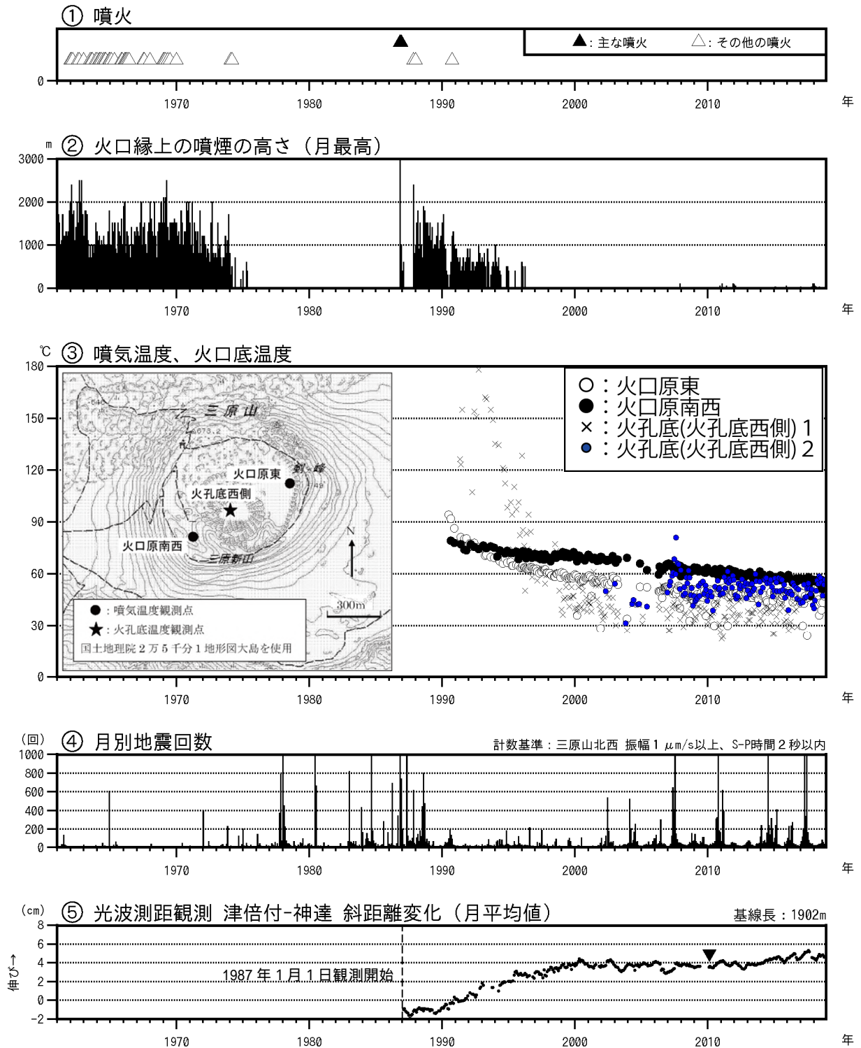
図1 伊豆大島 長期間の火山活動経過図（1961年1月～2018年11月30日）
