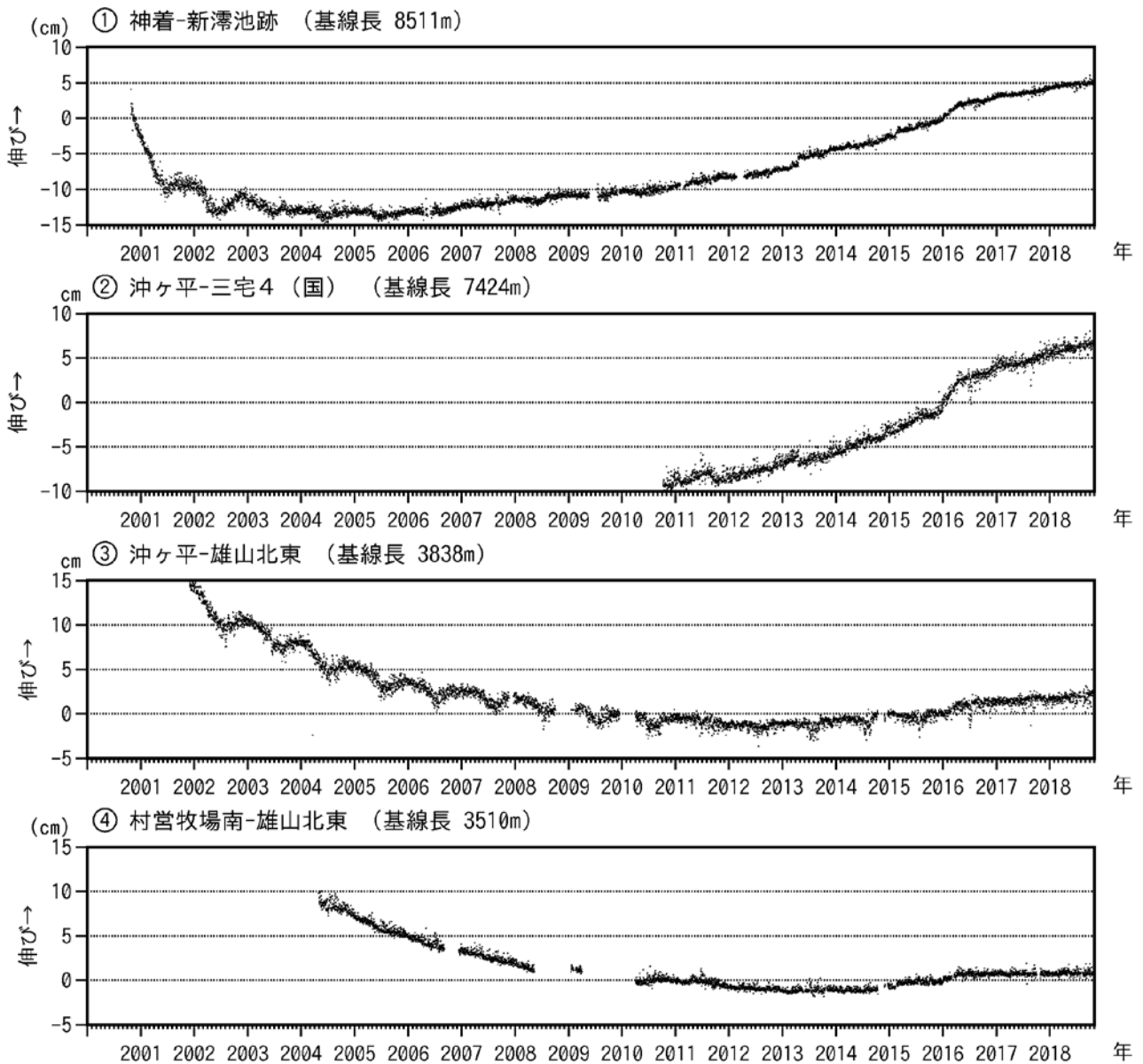
図7 三宅島 GNSS 連続観測結果（2000年10月26日～2018年10月31日）
