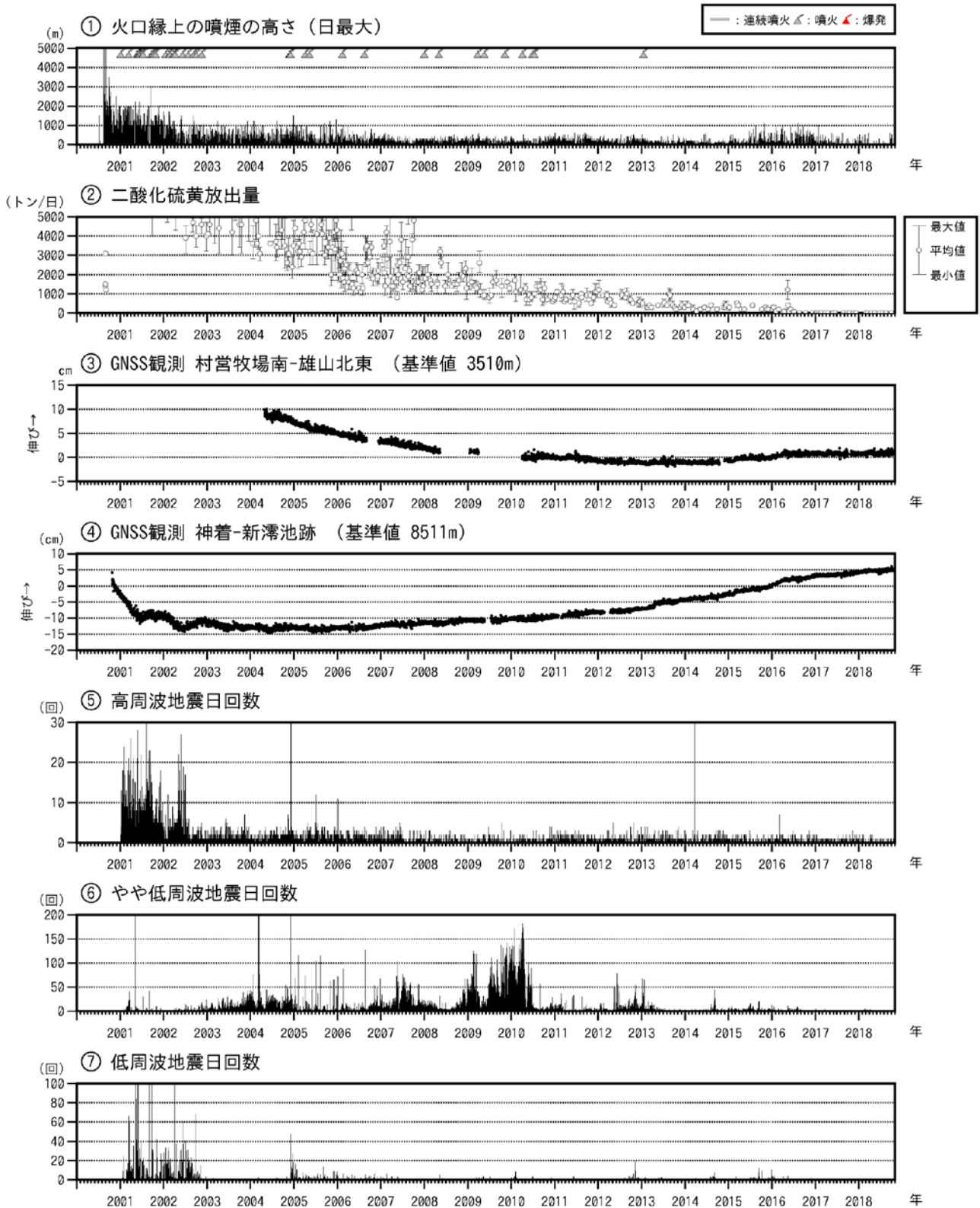
図5 三宅島 火山活動長期経過図（2000年1月1日～2018年10月31日） ※図5の説明は次ページに掲載しています。
