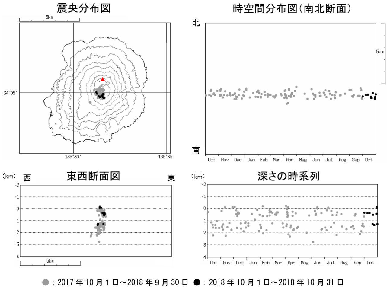
図 8 三宅島 震源分布図（2017 年 10 月 1 日～2018 年 10 月 31 日） 震源は山頂火口直下に分布しており、これまでと比べて特段の変化は認められません。
