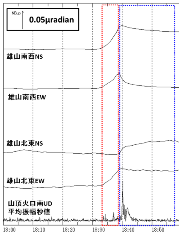
図9 三宅島 14日18時台の火山性微動と傾斜計の変動
