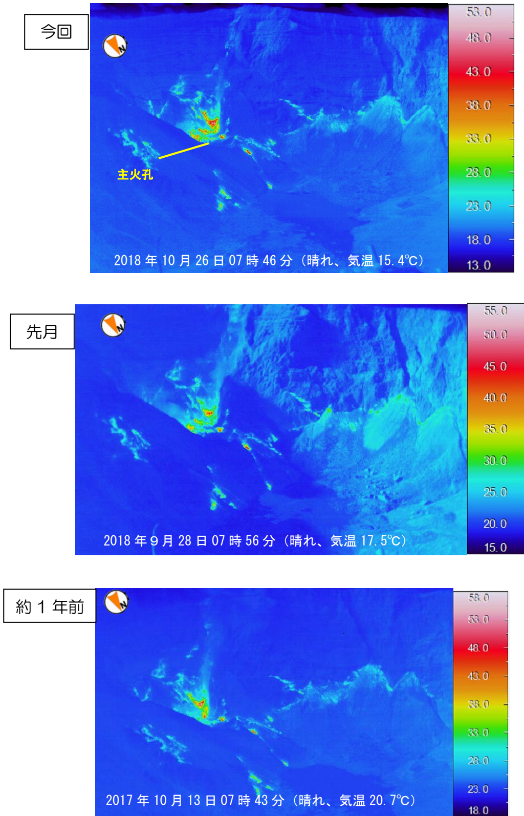
図 4 三宅島 赤外熱映像装置による山頂火口内の地表面温度分布 26 日に実施した現地調査では、9 月や昨年と同様に主火孔内及びその周辺で引き続き高温領域が認められました。高温領域の分布に特段の変化は認められません。
