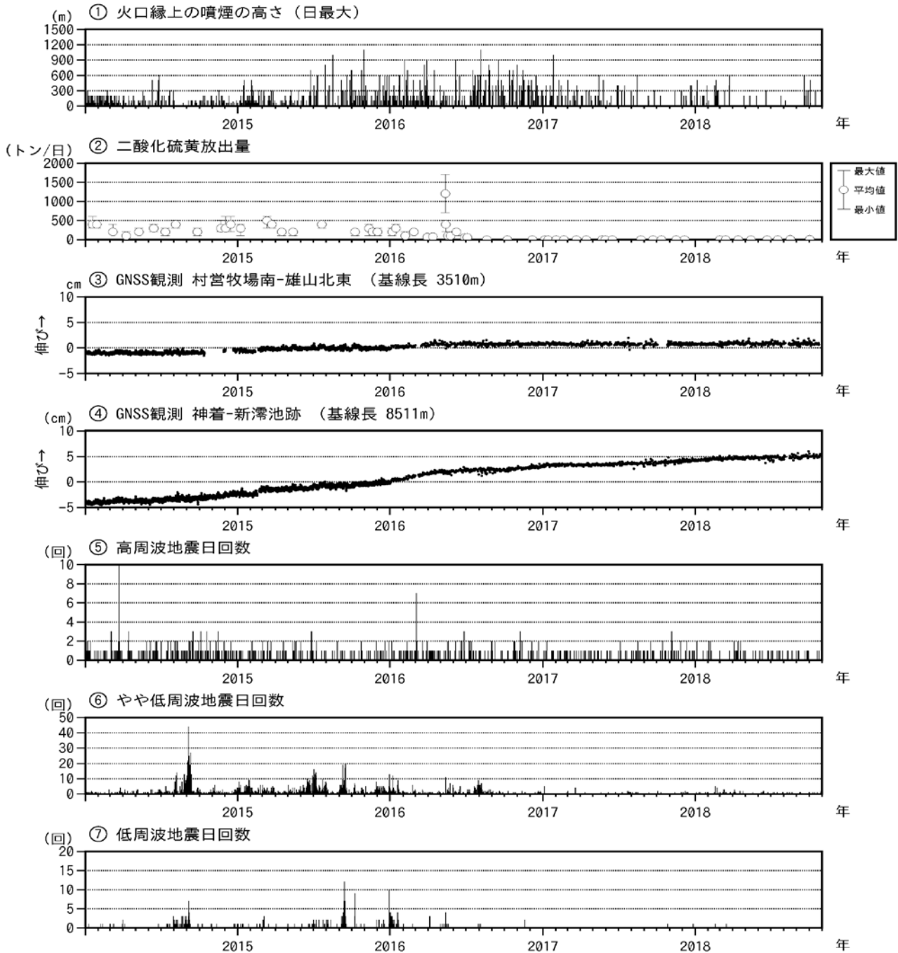
図6 三宅島 火山活動短期経過図（2014年1月1日～2018年10月31日）
