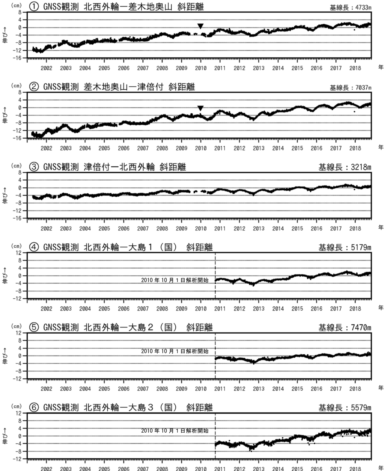
図3 伊豆大島 GNSS連続観測による基線長変化(2001年1月～2018年10月31日)
