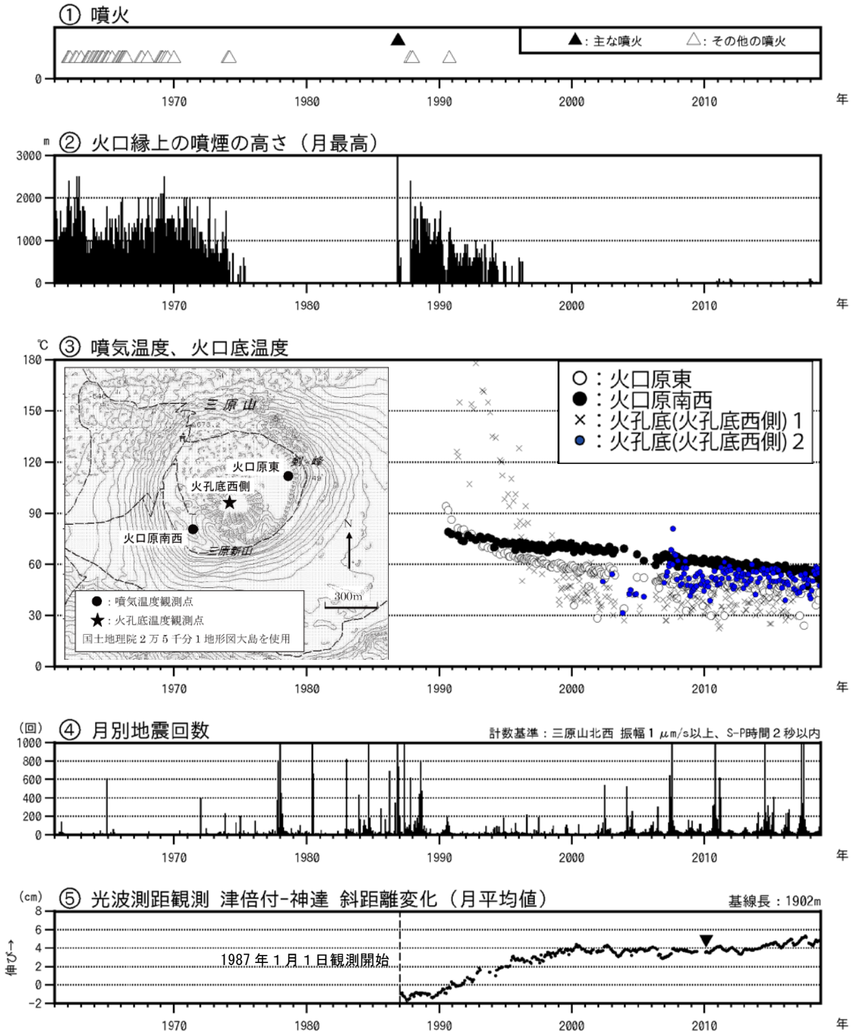
図1 伊豆大島 長期間の火山活動経過図（1961年1月～2018年10月31日）
