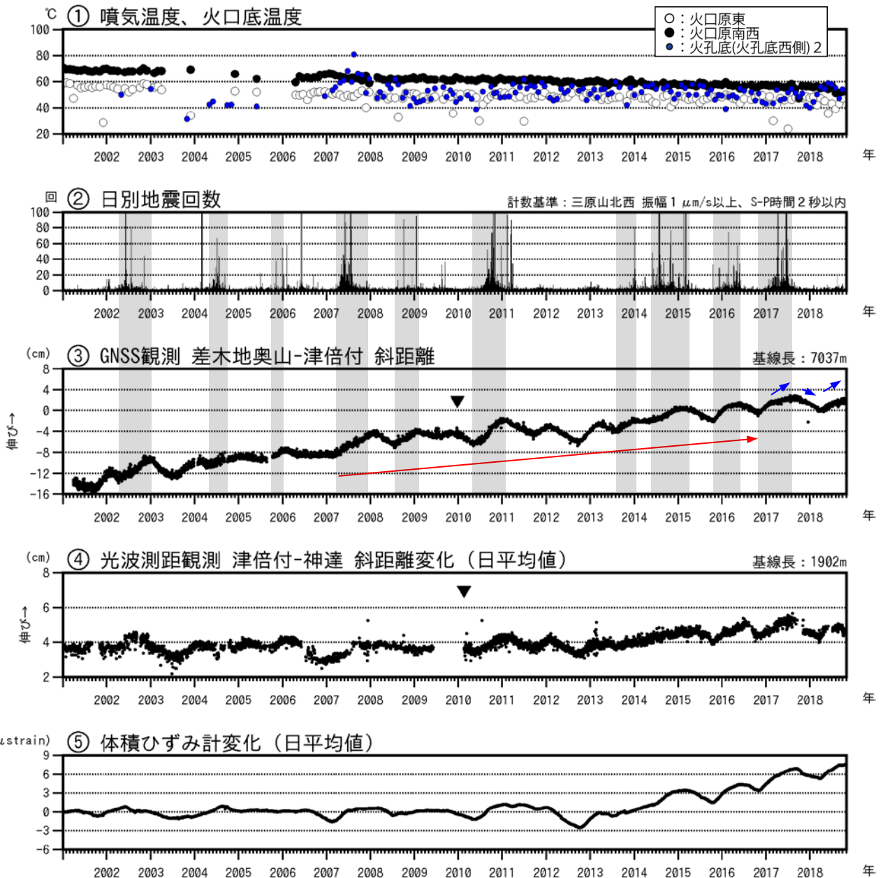
図 2 伊豆大島 最近の火山活動経過図（2001 年 1 月～2018 年 10 月 31 日）
