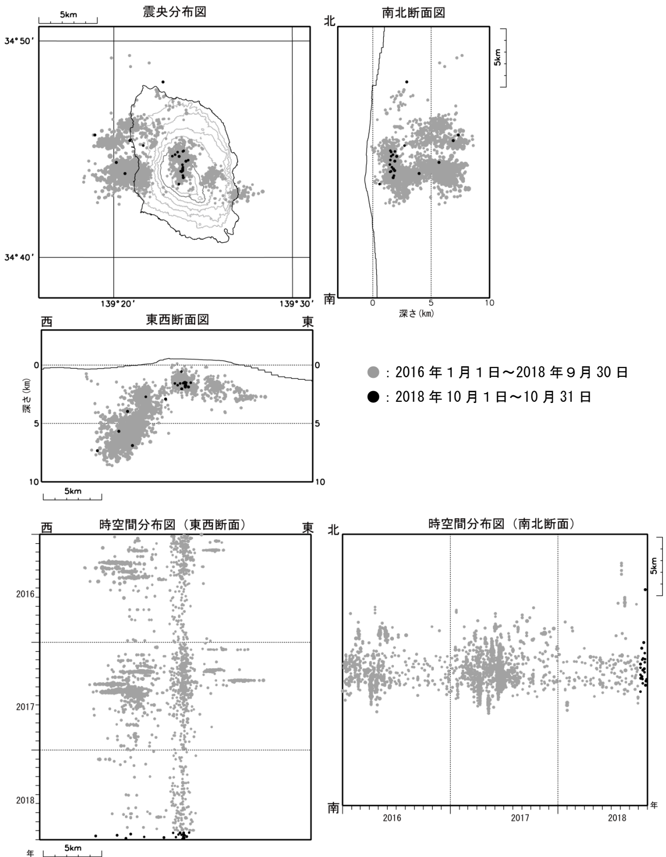
図4 伊豆大島 震源分布図（2016年1月1日～2018年10月31日）
