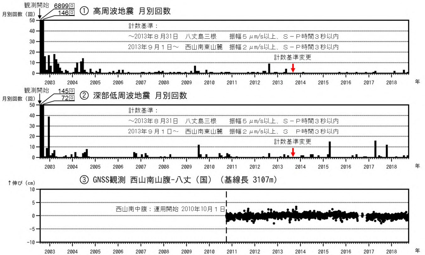
図2 八丈島 火山活動経過図(2002年8月13日~2018年9月30日)
