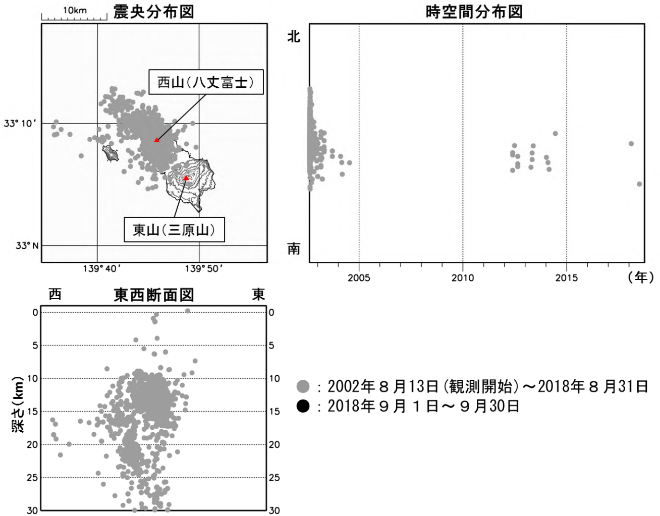
図3 八丈島 震源分布図(2002年8月13日~2018年9月30日) ・今期間、震源が求まる地震はありませんでした。
