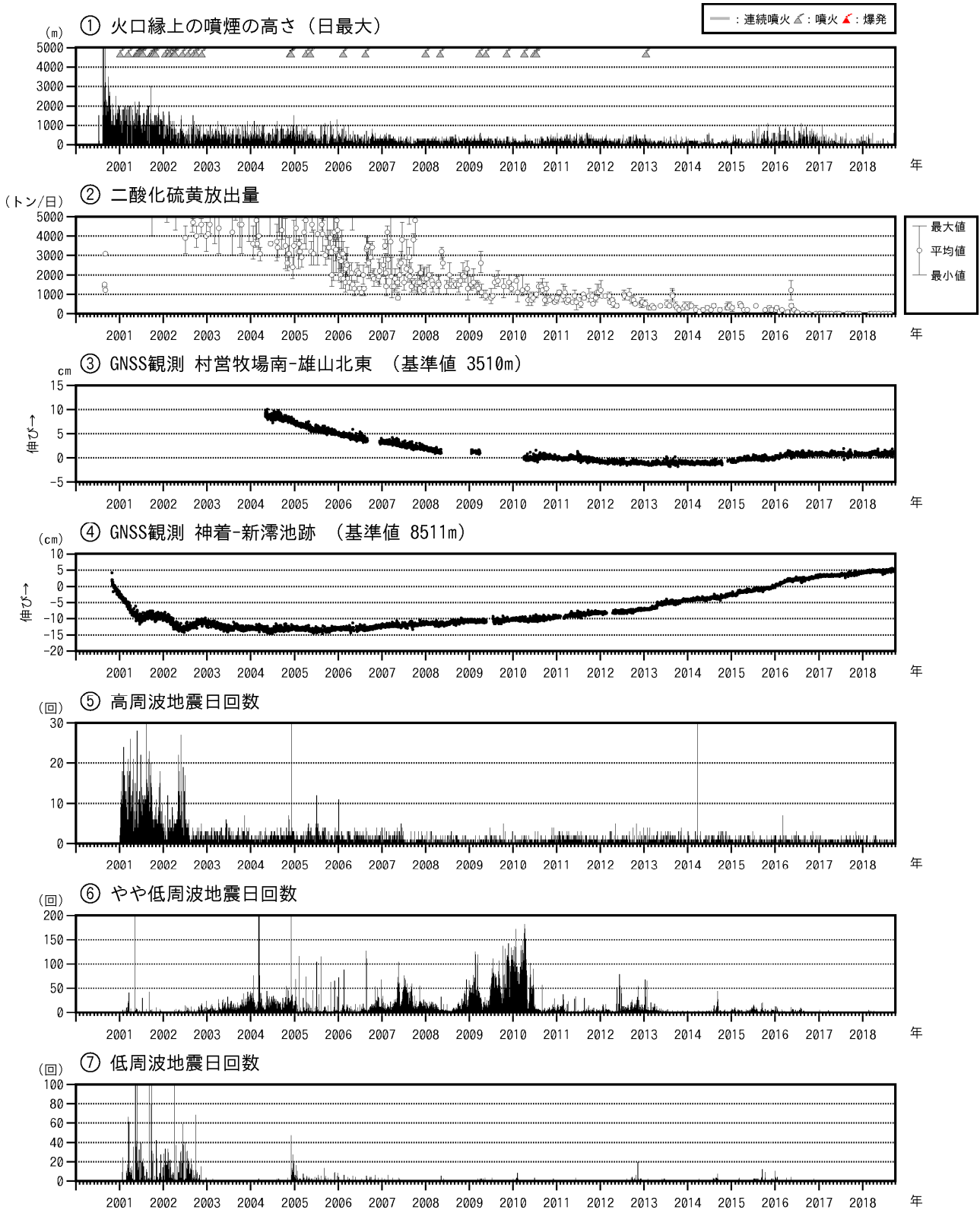
図5 三宅島 火山活動長期経過図（2000年1月1日～2018年9月30日）
