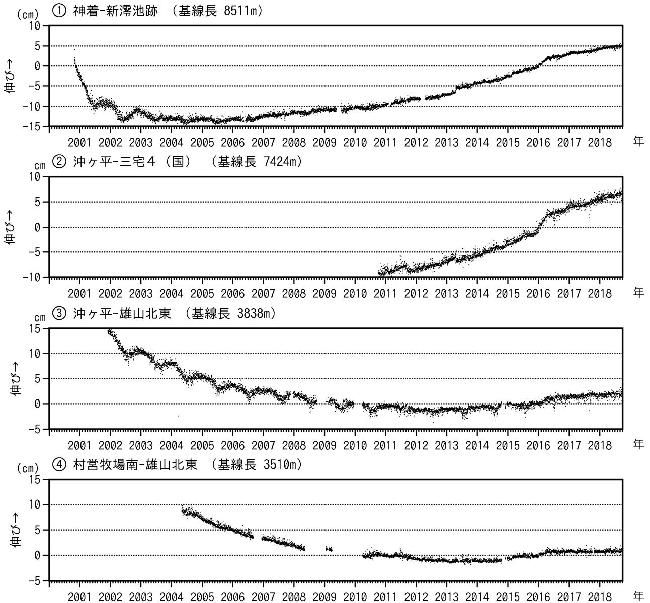
図7 三宅島 GNSS 連続観測結果 (2000年10月26日~2018年9月30日)
