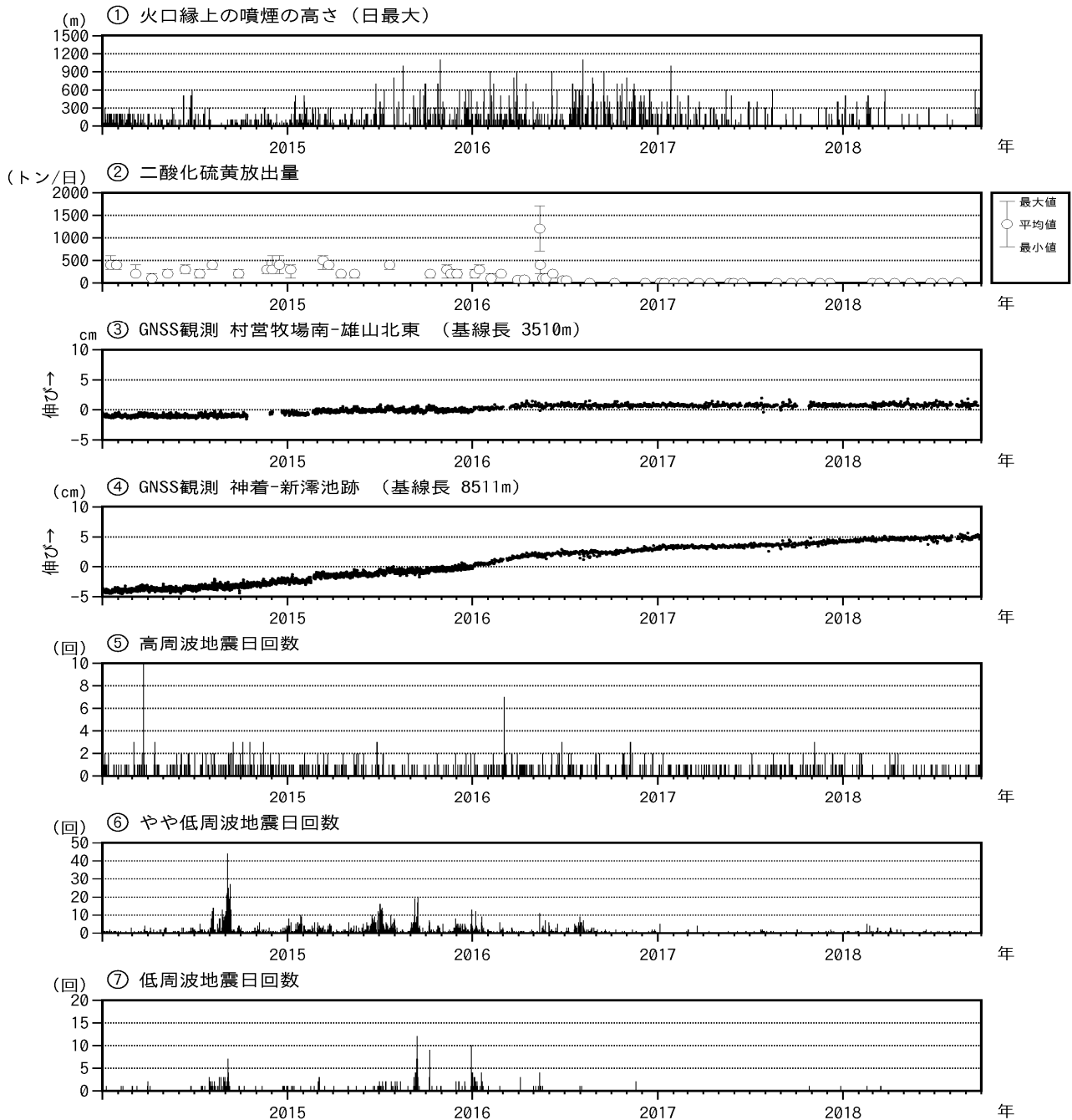
図6 三宅島 火山活動短期経過図(2014年1月1日~2018年9月30日)
