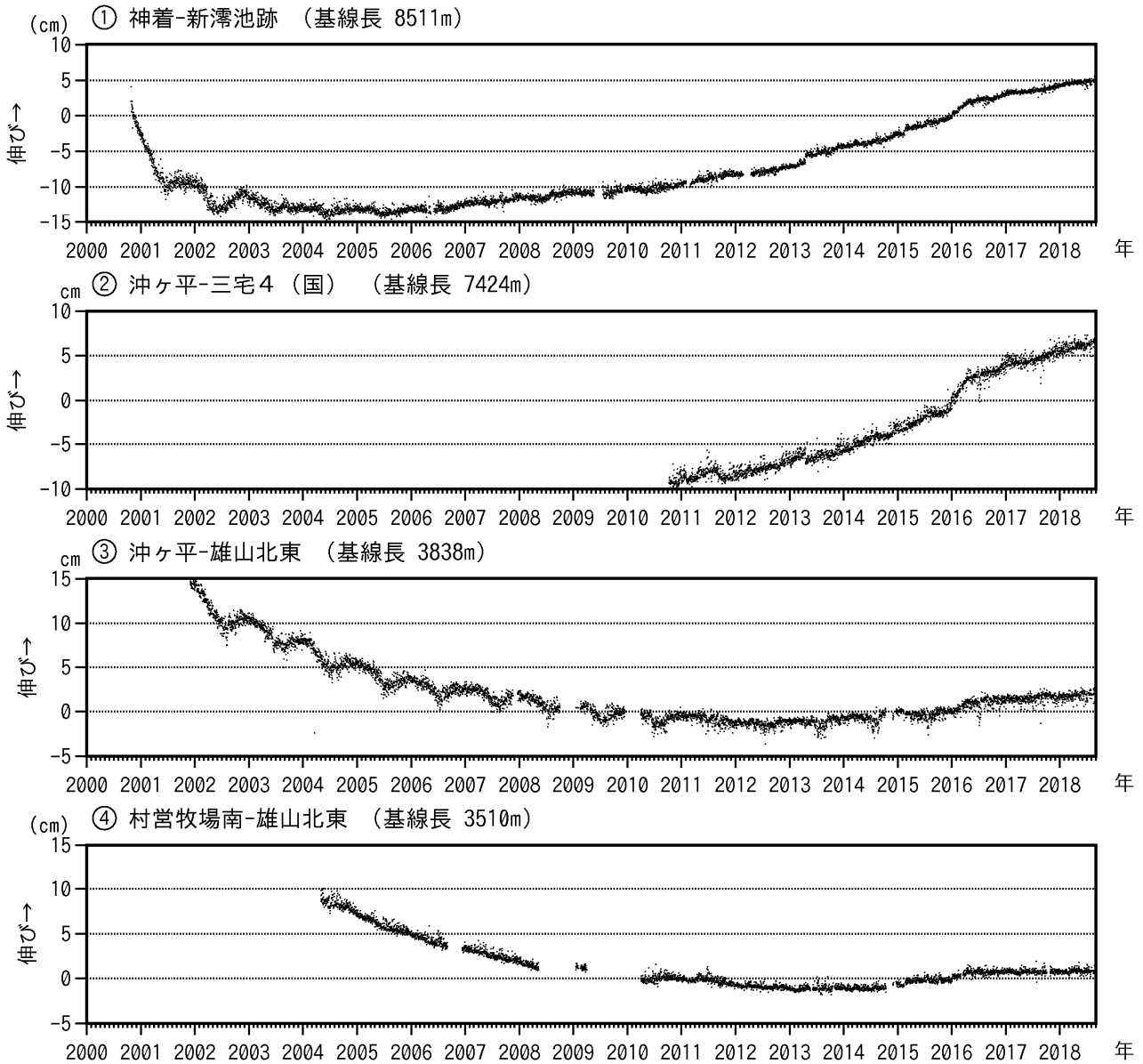
図7 三宅島 GNSS 連続観測結果 (2000年10月26日~2018年8月31日)
