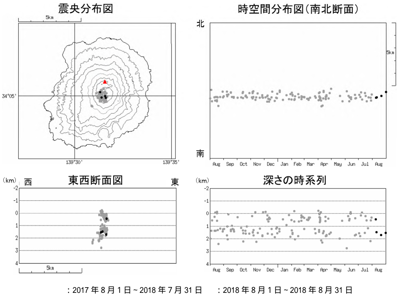
図8 三宅島 震源分布図(2017年8月1日~2018年8月31日) 震源は山頂火口直下に分布しており、これまでと比べて特段の変化は認められません。
