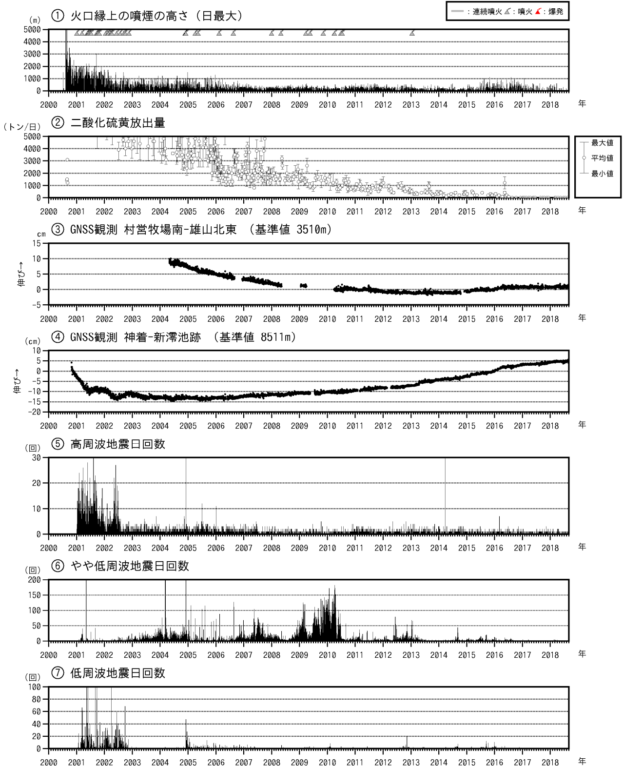
図5 三宅島 火山活動長期経過図（2000年1月1日～2018年8月31日） 図5の説明は次ページに掲載しています。
