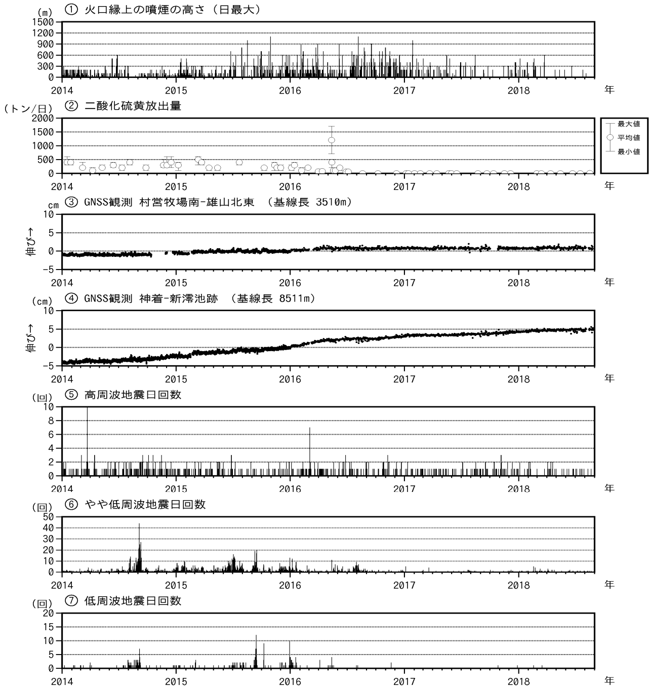
図6 三宅島 火山活動短期経過図(2014年1月1日~2018年8月31日)
