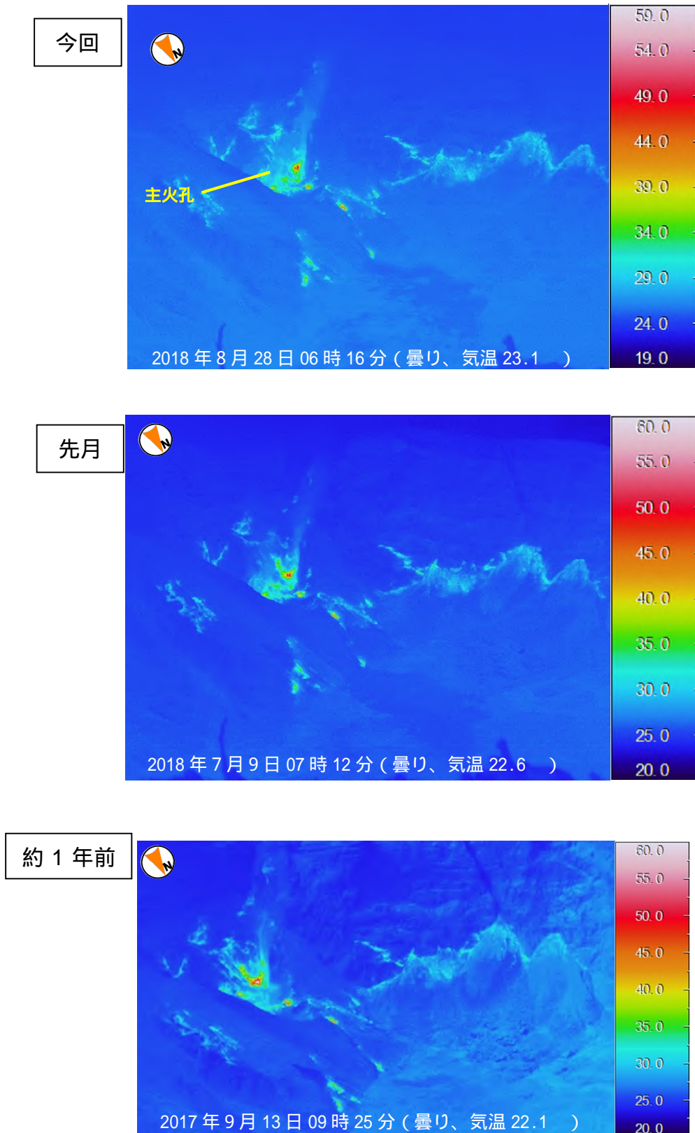
図 4 三宅島 赤外熱映像装置による山頂火口内の地表面温度分布 28 日に実施した現地調査では、7 月や昨年と同様に主火口内及びその周辺で引き続き高温領域が認められました。高温領域の分布に特段の変化は認められません。
