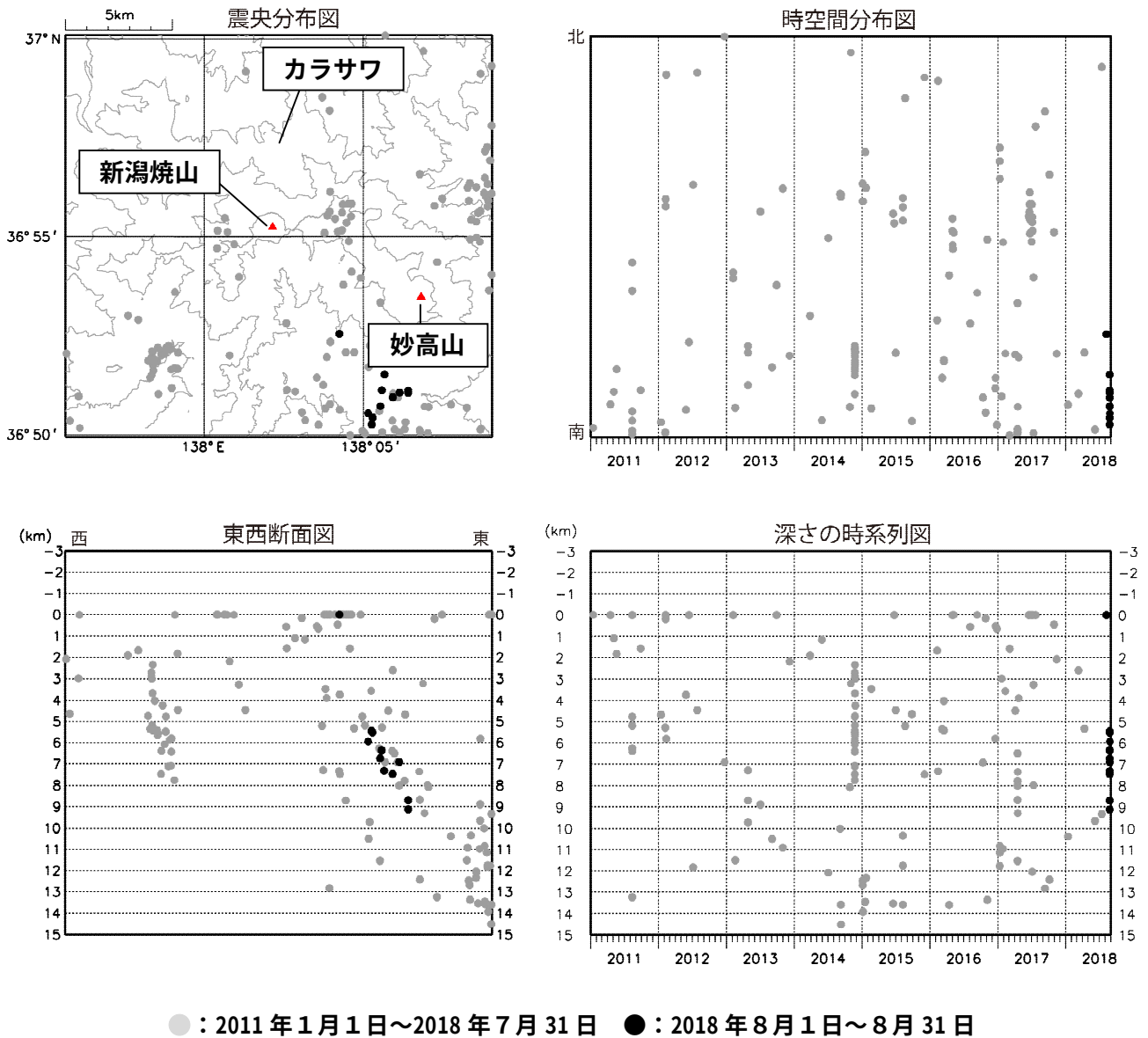
図 8 新潟焼山 広域地震観測網による山体・周辺の地震活動（2011 年 1 月 1 日～2018 年 8 月 31 日）
