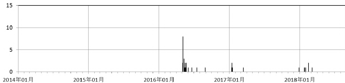
図 6 新潟焼山 日別地震回数（2014 年 1 月 1 日～2018 年 8 月 31 日）
