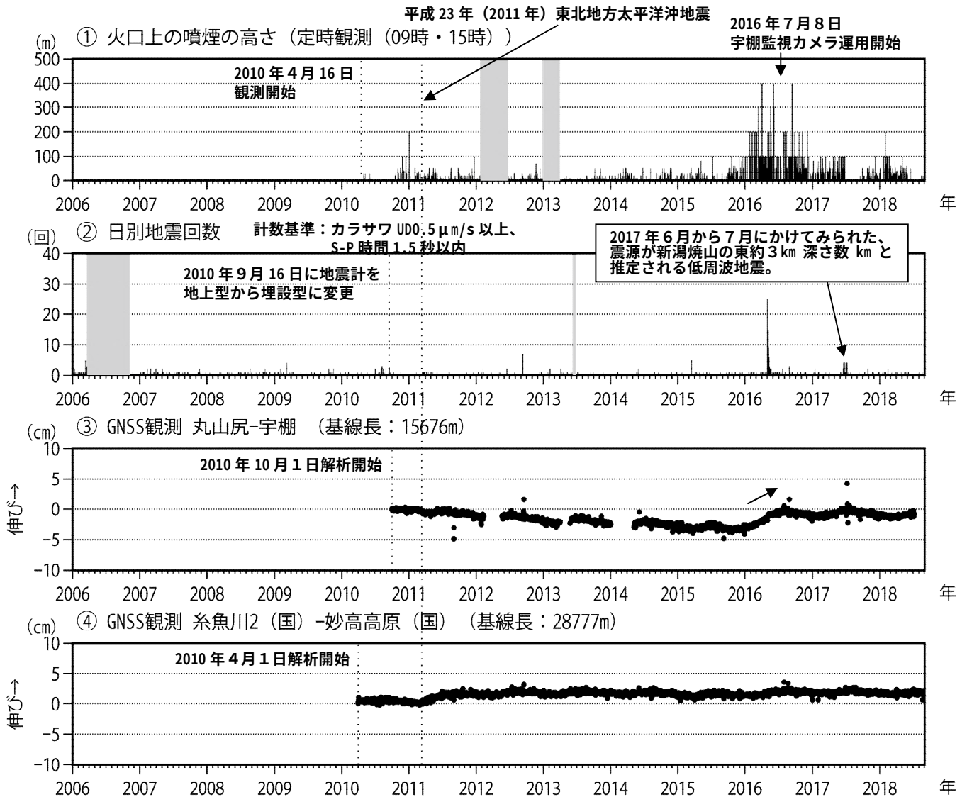
図 3 新潟焼山 火山活動経過図（2006 年 1 月 1 日～2018 年 8 月 31 日）
