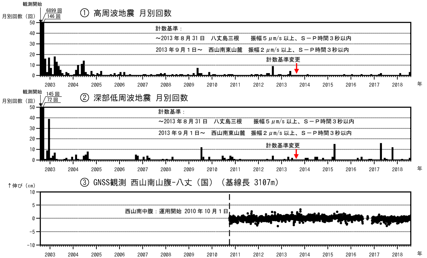
図2 八丈島 火山活動経過図 (2002年8月13日~2018年7月31日)
