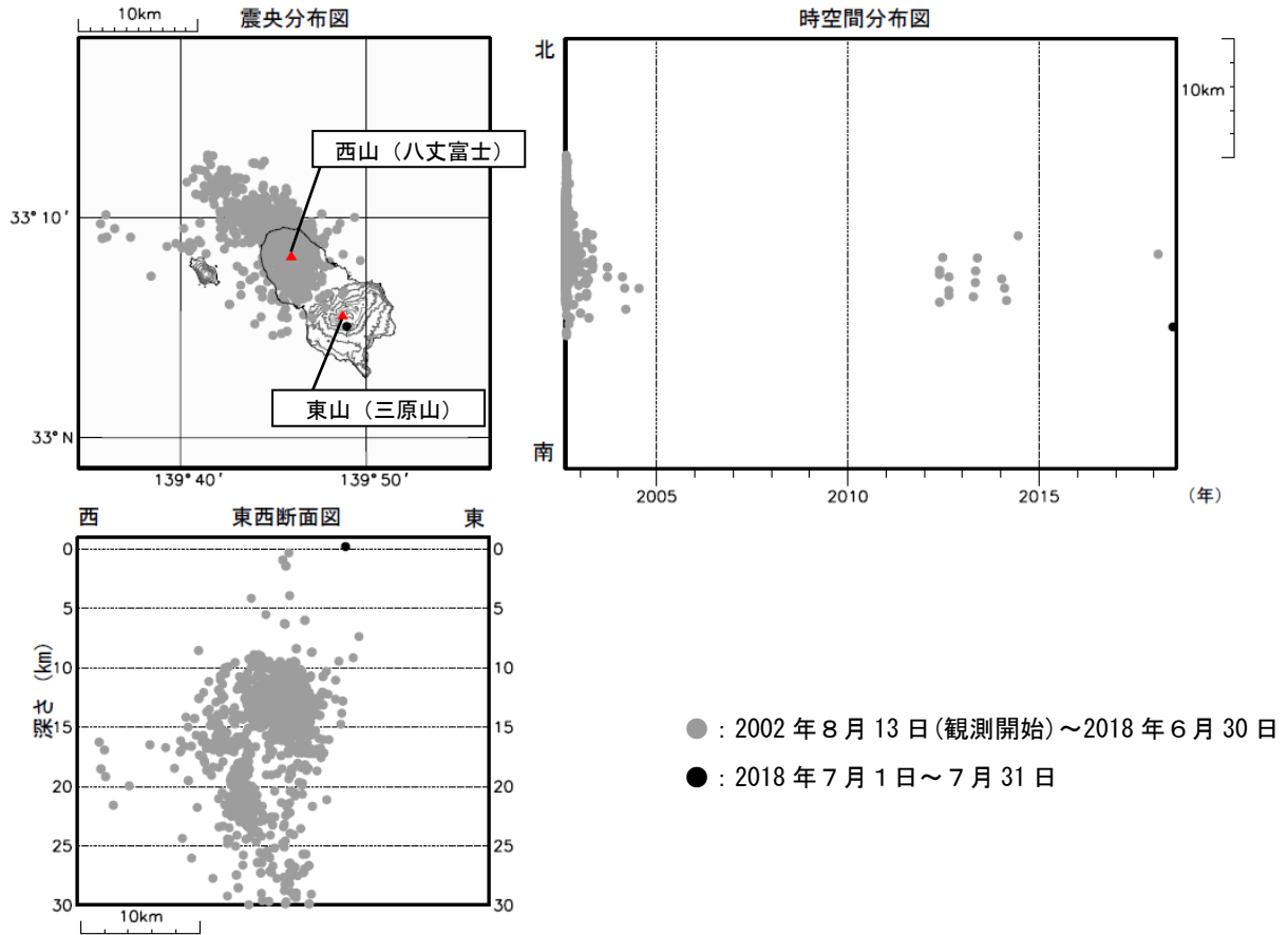
図3 八丈島 震源分布図（2002年8月13日～2018年7月31日）
