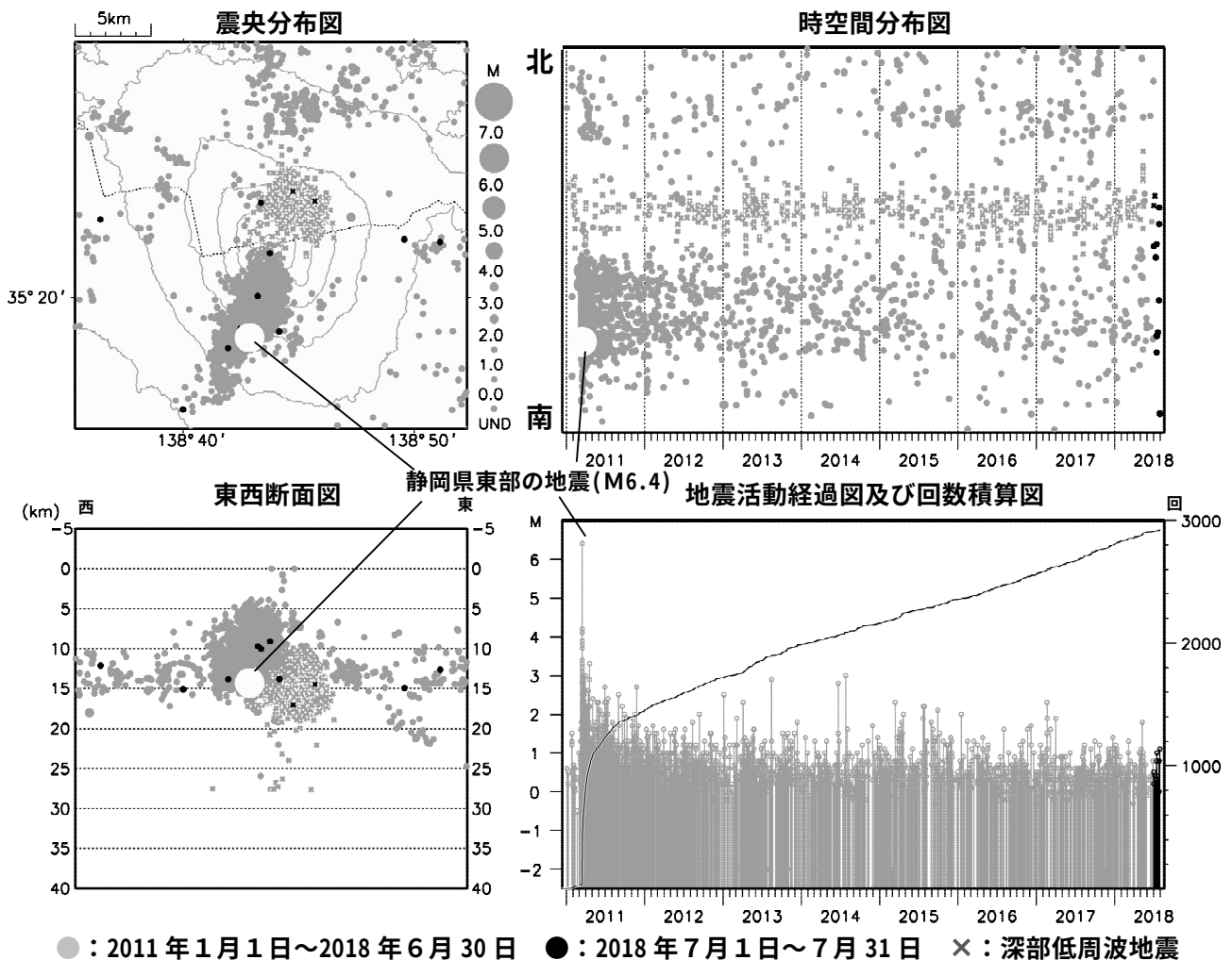
図3 富士山 広域地震観測網による山体・周辺の地震活動（2011年1月1日～2018年7月31日）
