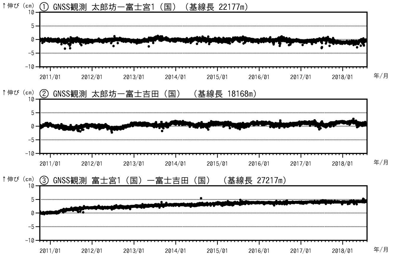
図4 富士山 GNSS 連続観測による基線長変化 (2010 年 10 月 1 日～2018 年 7 月 31 日)
