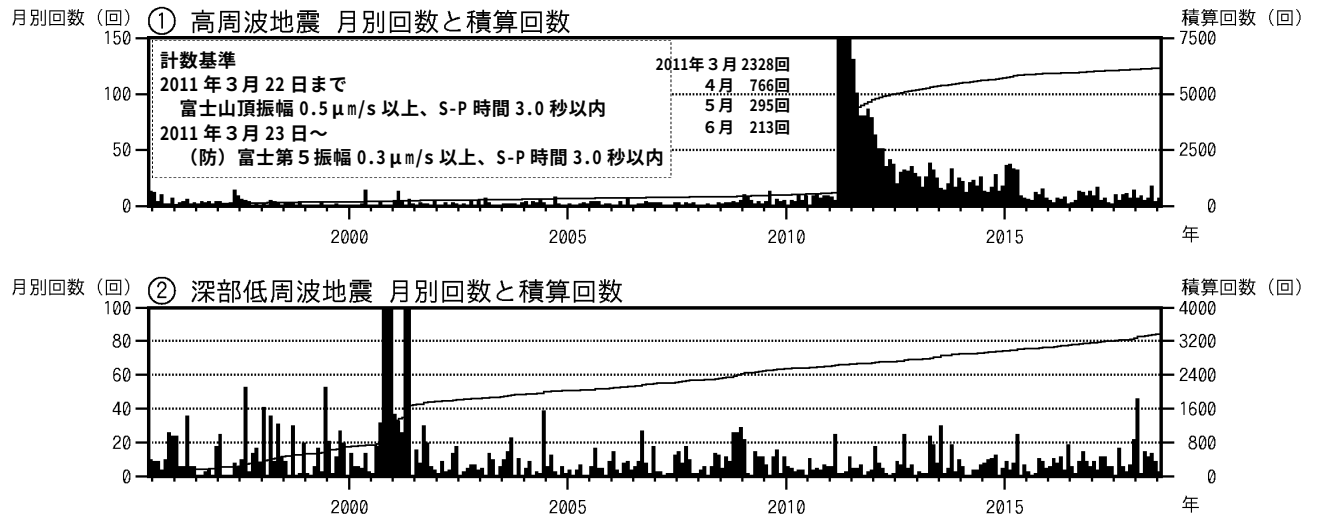
図2 富士山 月別地震回数（1995年6月1日～2018年7月31日）
