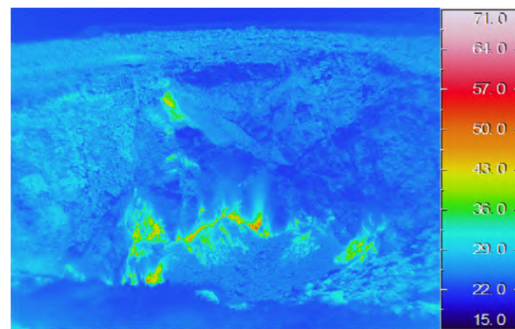
2018年6月22日11時15分 気温:25、曇り
