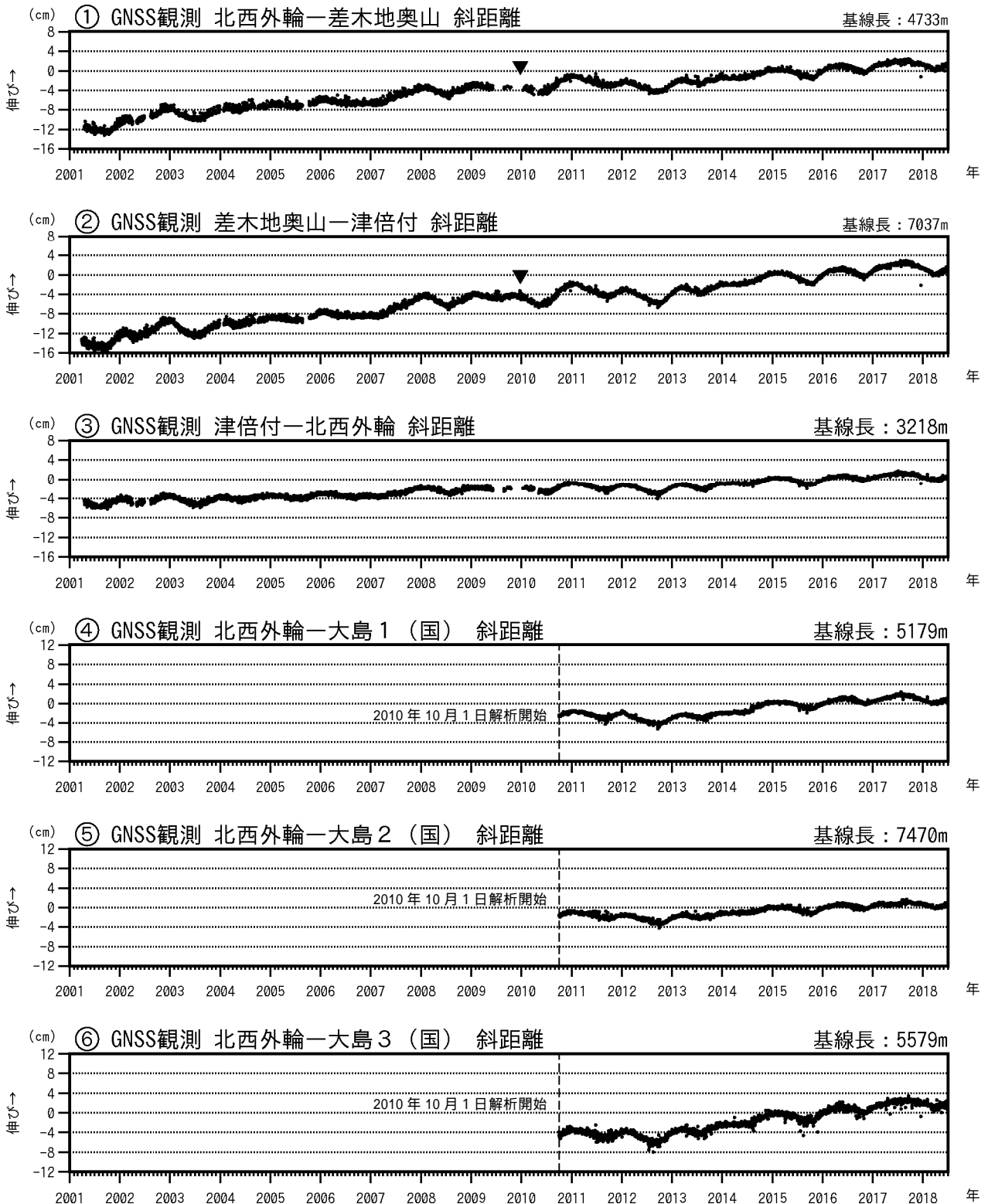
図3 伊豆大島 GNSS連続観測による基線長変化(2001年1月～2018年6月30日) (国): 国土地理院、～は図8のGNSS基線～に対応、グラフの空白部分は欠測。 2010年10月及び2016年1月以降のデータについては、解析方法を変更しています。 ～は差木地奥山観測点の支柱工事を実施。
