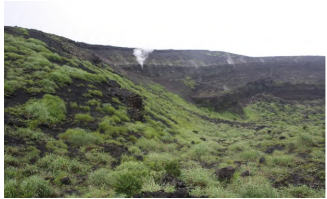
剣ガ峰付近(6月22日、撮影方向は図7参照)
