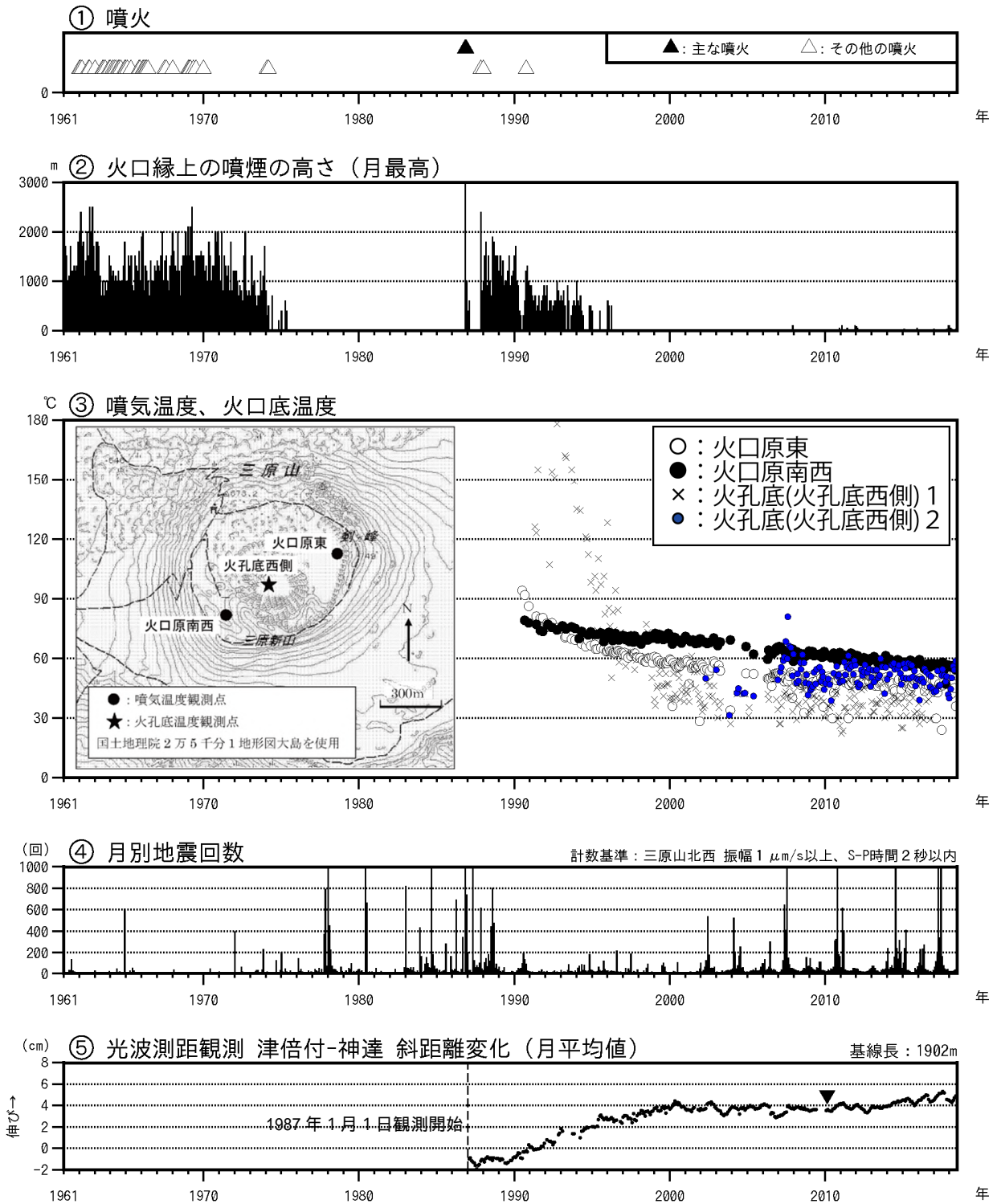
図1 伊豆大島 長期間の火山活動経過図(1961年1月~2018年6月30日)
