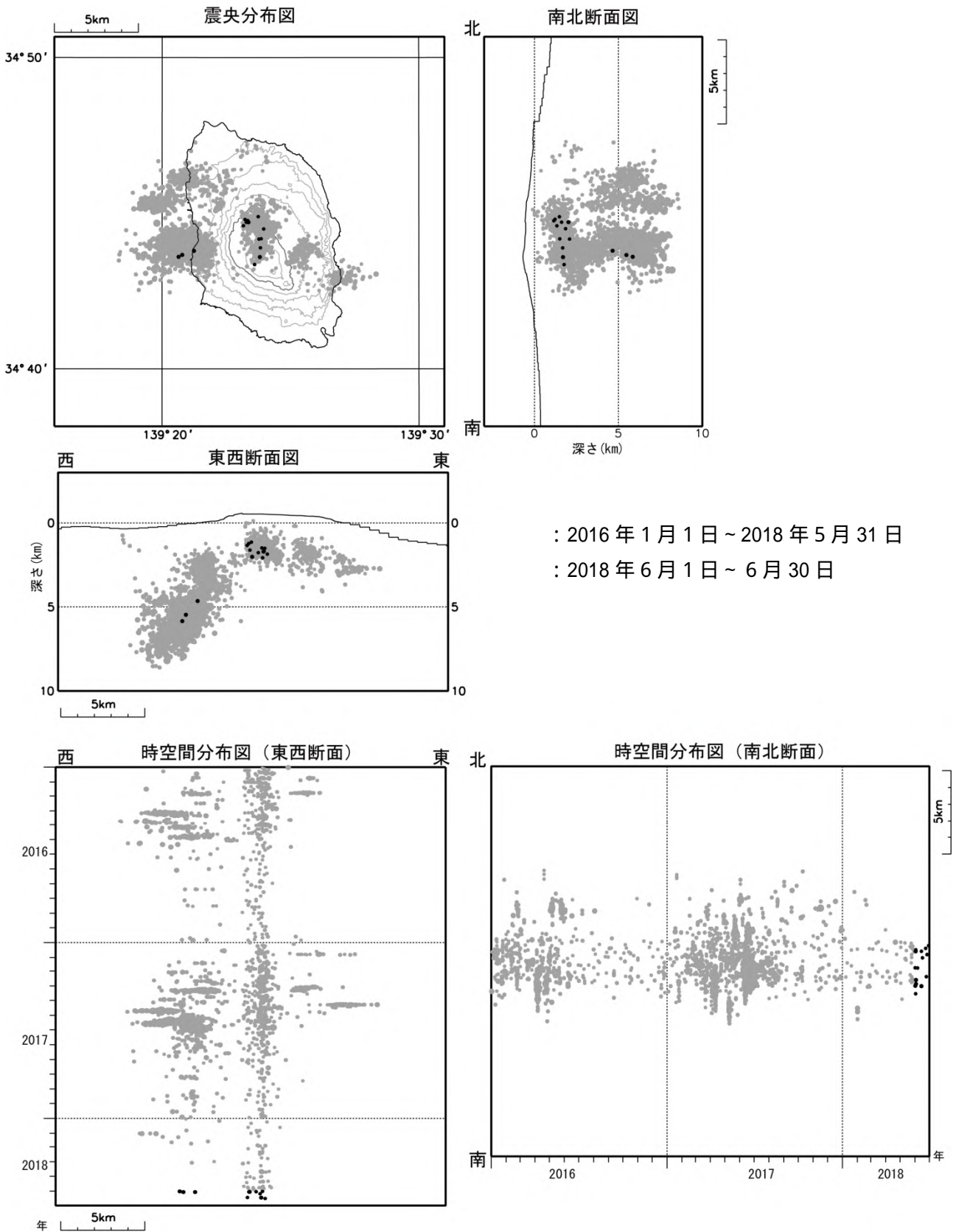
図4 伊豆大島 震源分布図(2016年1月1日～2018年6月30日)
