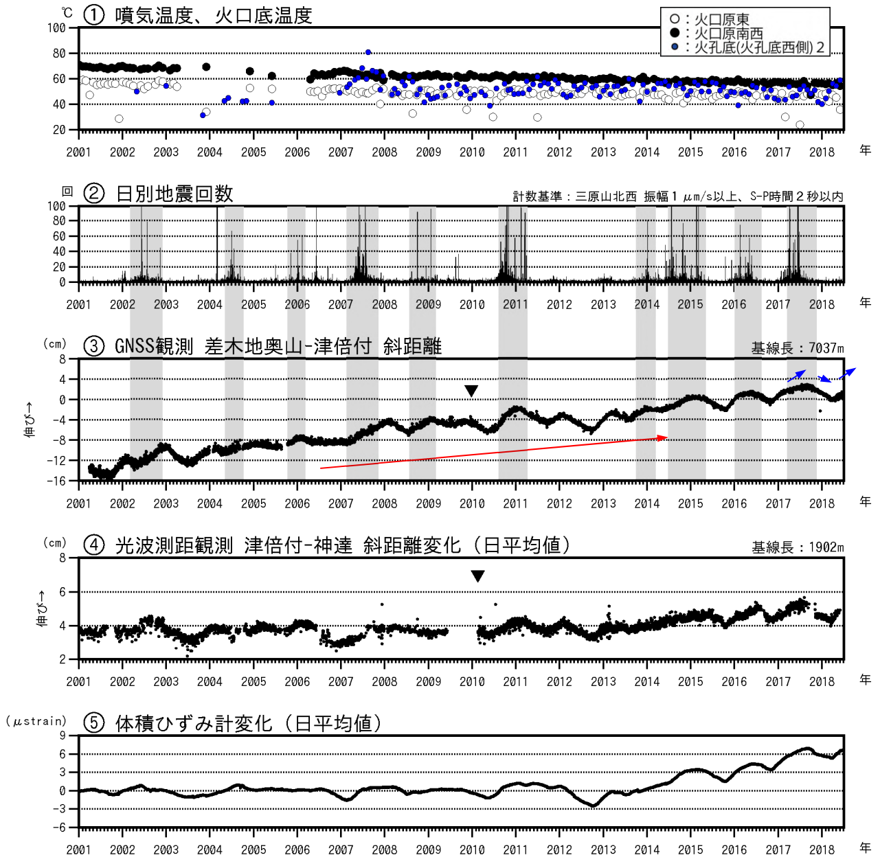
図2 伊豆大島 最近の火山活動経過図(2001年1月~2018年6月30日)
