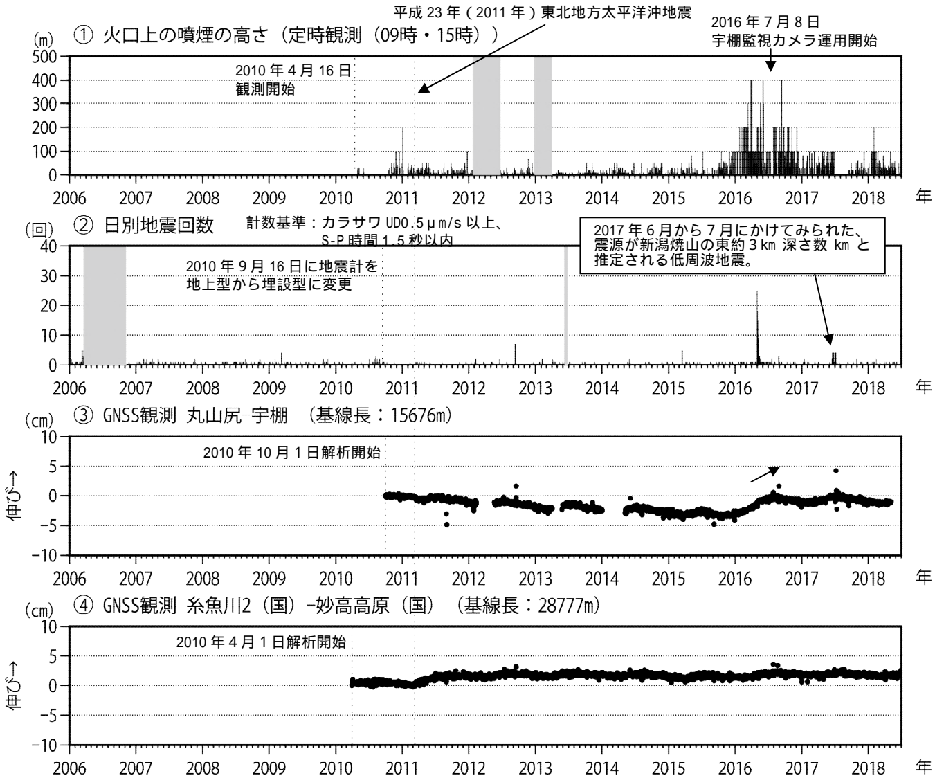
図3 新潟焼山 火山活動経過図(2006年1月1日~2018年6月30日)
