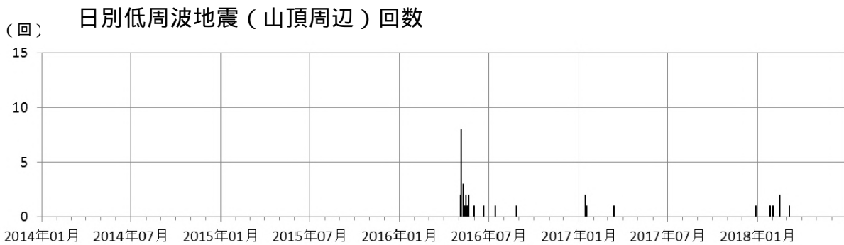
図6 新潟焼山 日別地震回数(2014年1月1日~2018年6月30日)
