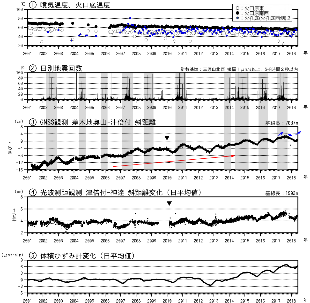
図2 伊豆大島 最近の火山活動経過図(2001年1月~2018年5月31日)
