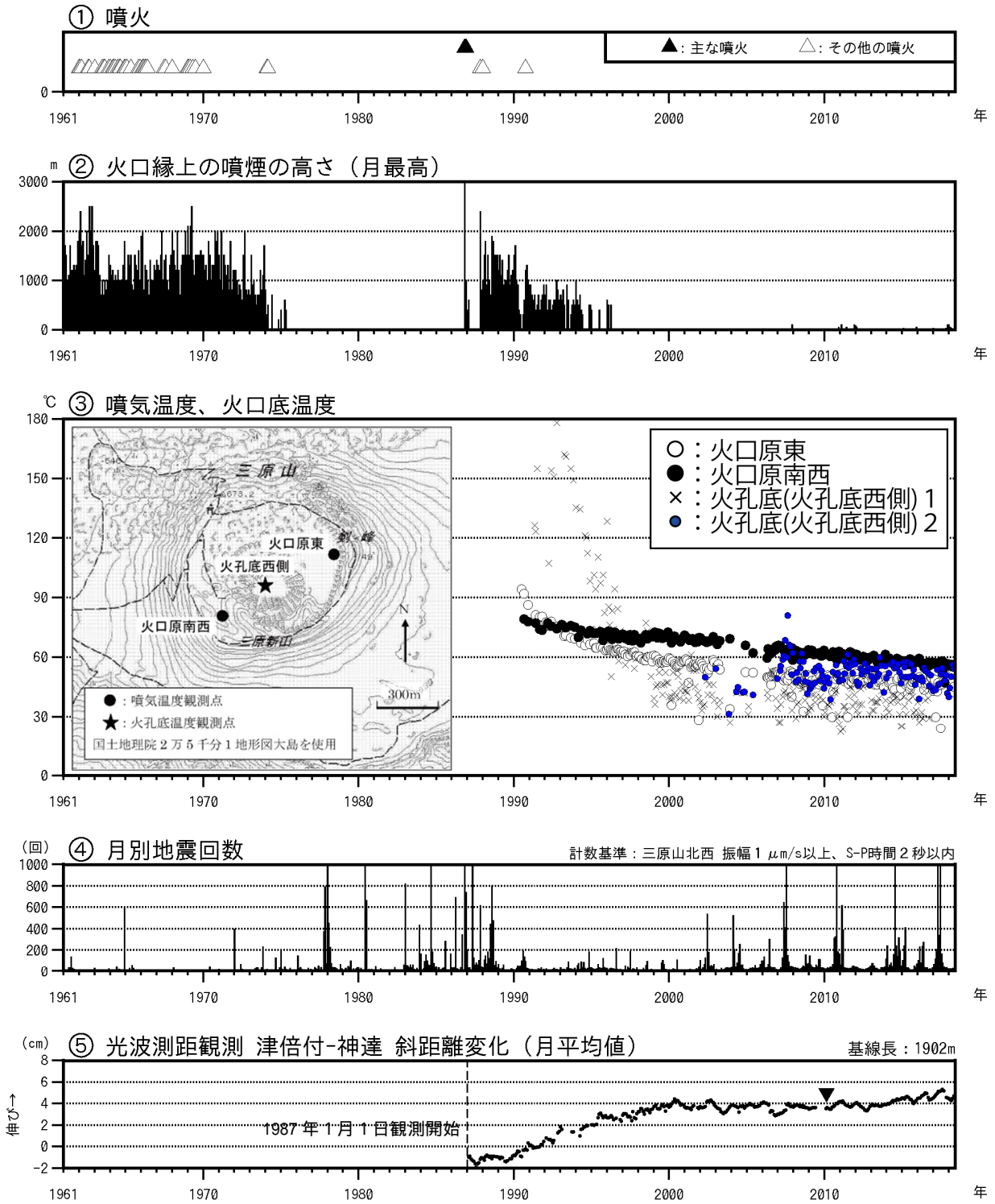
図1 伊豆大島 長期間の火山活動経過図(1961年1月~2018年5月31日)
