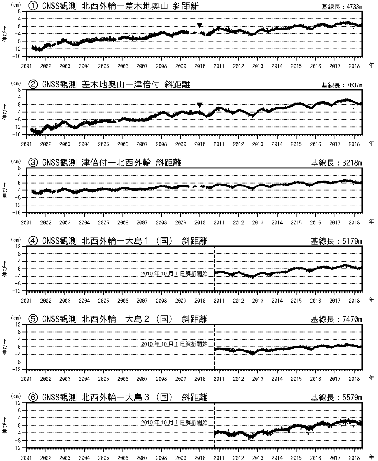
図3 伊豆大島 GNSS 連続観測による基線長変化(2001年1月~2018年5月31日) (国): 国土地理院、~ は図8のGNSS基線 ~ に対応、グラフの空白部分は欠測。 2010年10月及び2016年1月以降のデータについては、解析方法を変更しています。 は差木地奥山観測点の支柱工事を実施。
