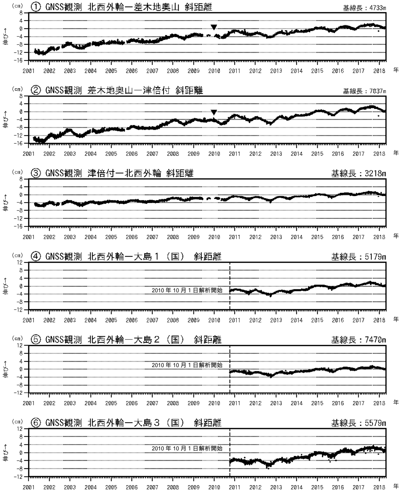
図3 伊豆大島 GNSS連続観測による基線長変化(2001年1月~2018年4月30日)
