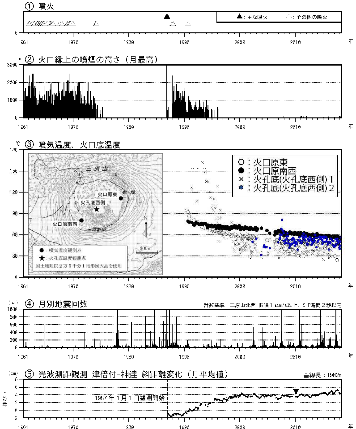
図1 伊豆大島 長期間の火山活動経過図(1961年1月~2018年4月30日)
