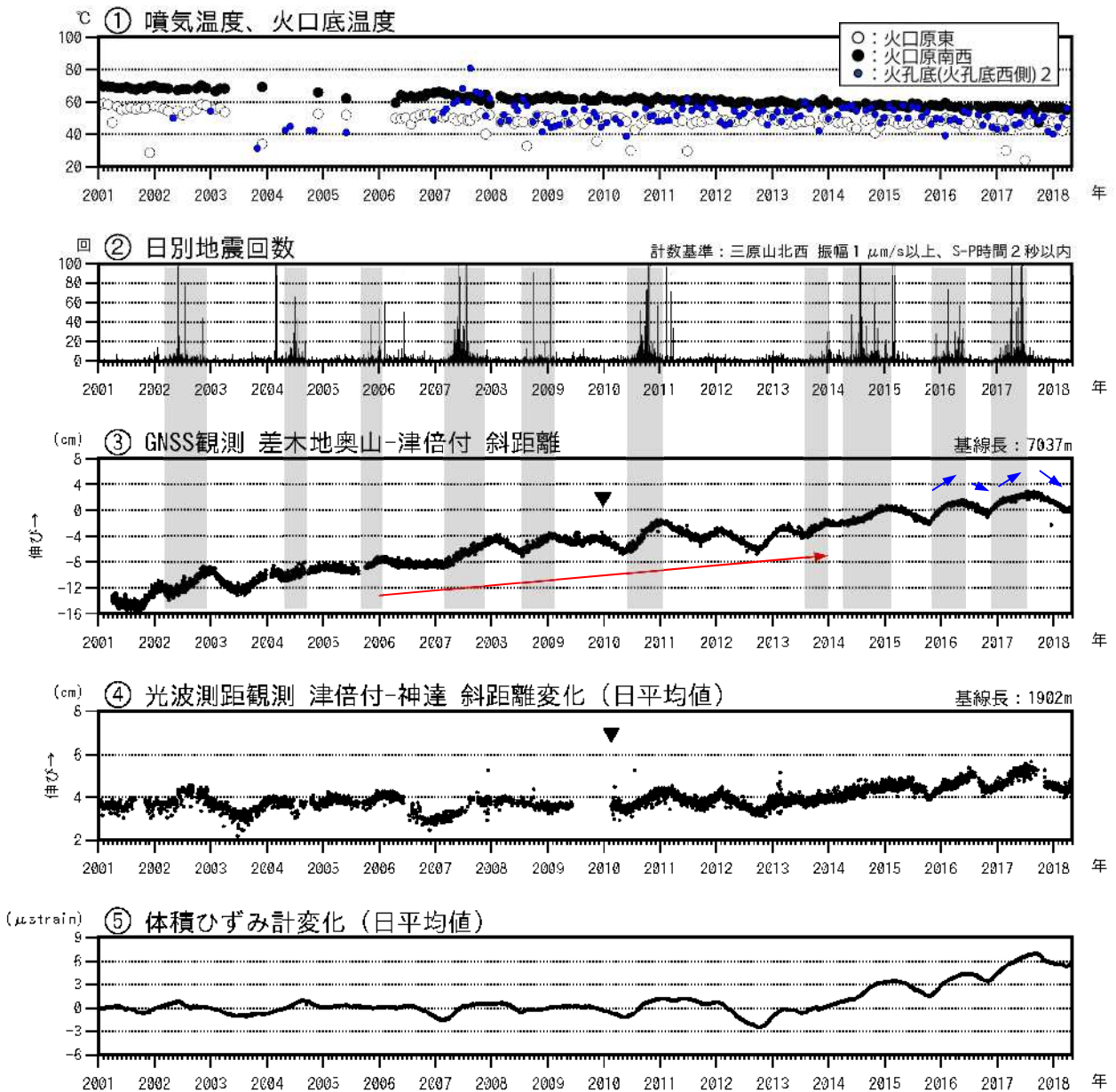
図 2 伊豆大島 最近の火山活動経過図（2001 年 1 月～2018 年 4 月 30 日）
