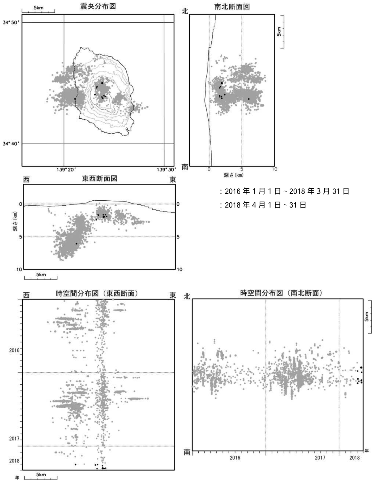
図4 伊豆大島 震源分布図(2016年1月1日～2018年4月30日)
