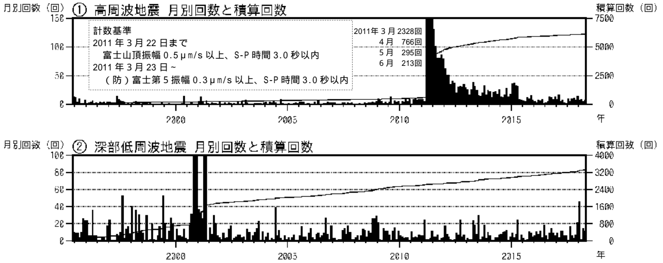
図2 富士山 月別地震回数(1995年6月1日～2018年4月30日)
