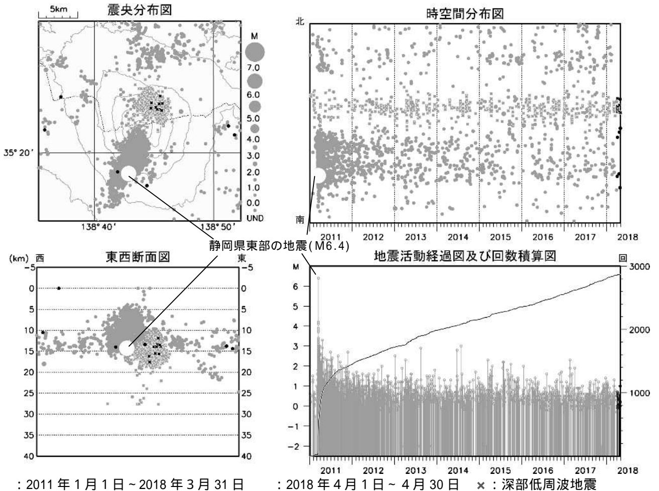
図3 富士山 広域地震観測網による山体・周辺の地震活動(2011年1月1日～2018年4月30日)
