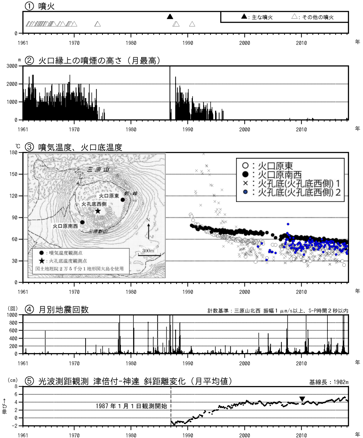
図 1 伊豆大島 長期間の火山活動経過図（1961 年 1 月～2018 年 3 月 31 日）
