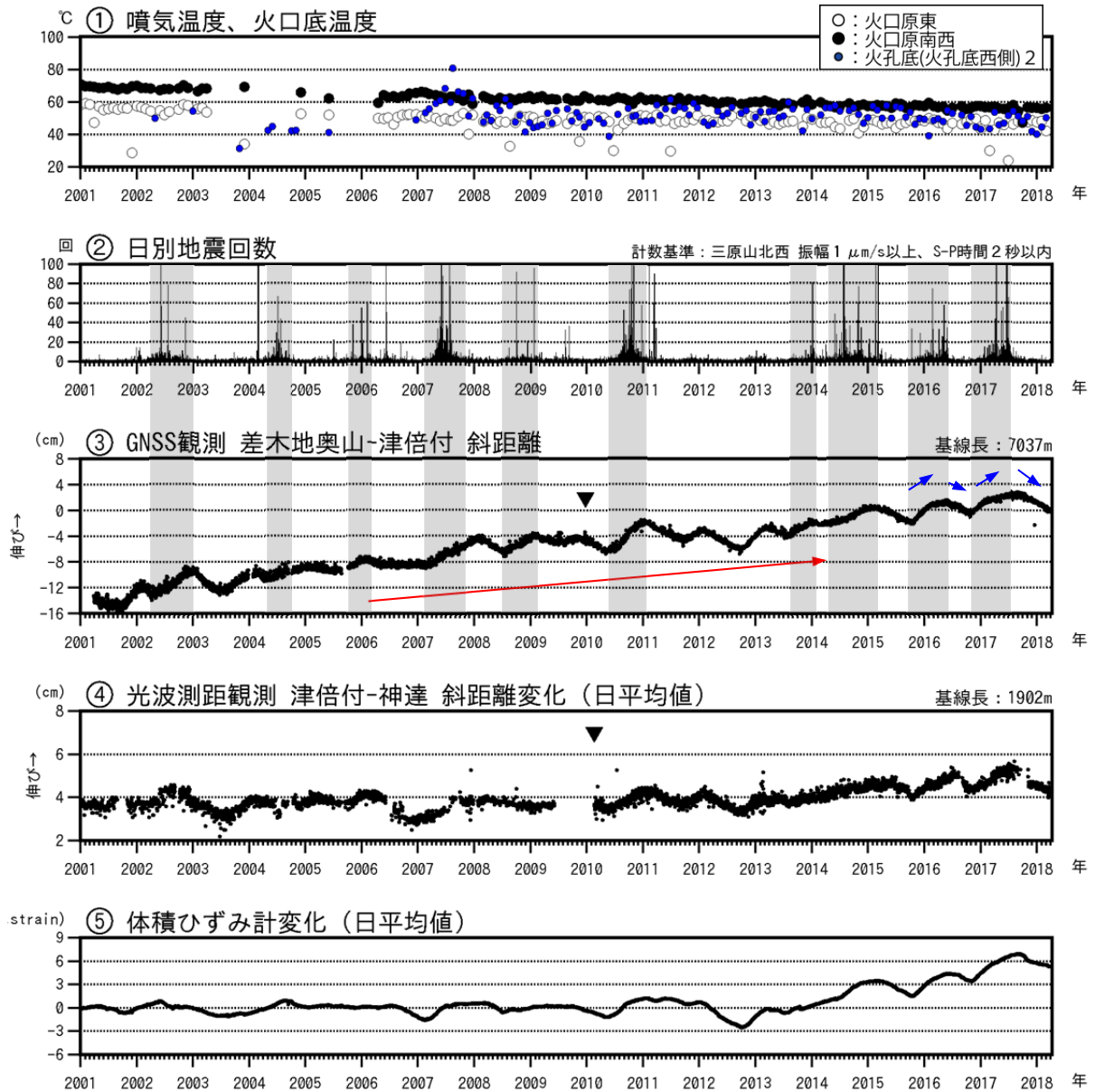
図 2 伊豆大島 最近の火山活動経過図（2001 年 1 月～2018 年 3 月 31 日）
