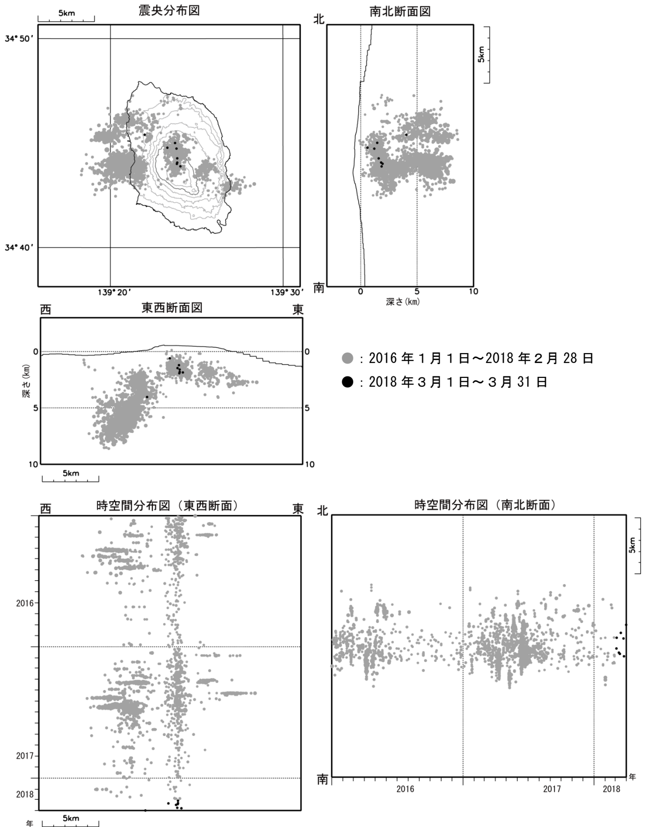
図4 伊豆大島 震源分布図（2016年1月1日～2018年3月31日）
