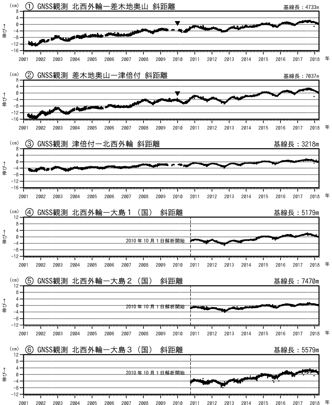
図3 伊豆大島 GNSS連続観測による基線長変化(2001年1月～2018年3月31日)
