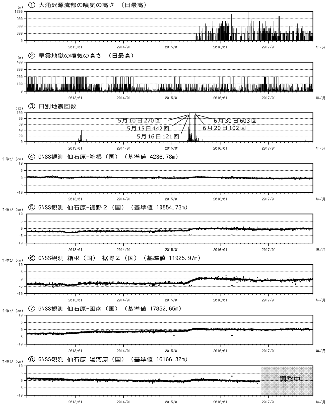
図5 箱根山 火山活動経過図（2012年1月1日～2017年11月30日）
