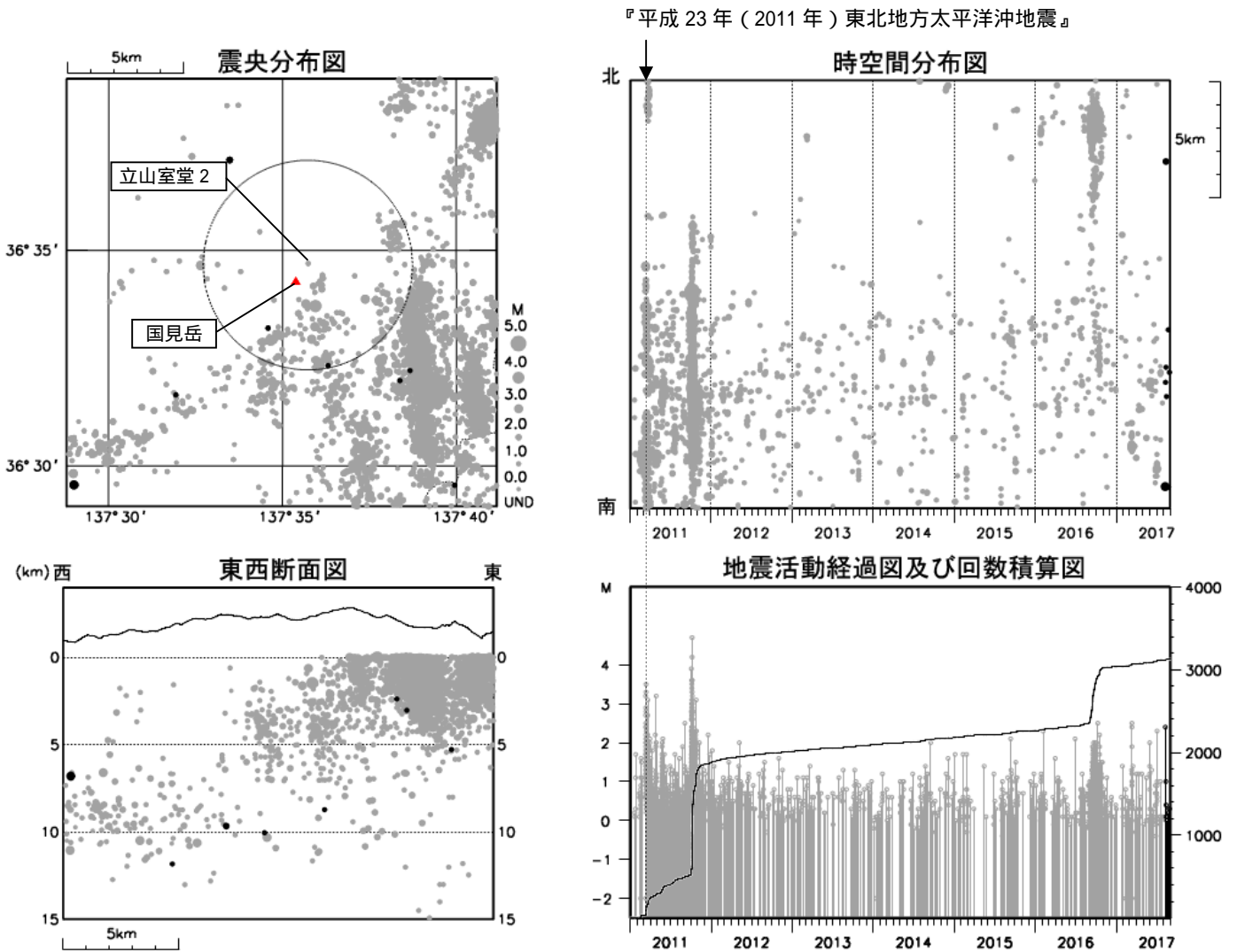
図 2 弥陀ヶ原 広域地震観測網による山体・周辺の地震活動 (2011 年 1 月 1 日 ~ 2017 年 8 月 31 日) : 2011 年 1 月 1 日 ~ 2017 年 7 月 31 日 : 2017 年 8 月 1 日 ~ 8 月 31 日
