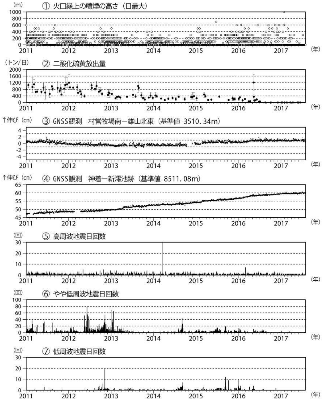
図6 三宅島 火山活動短期経過図(2011年1月1日~2017年7月31日)
