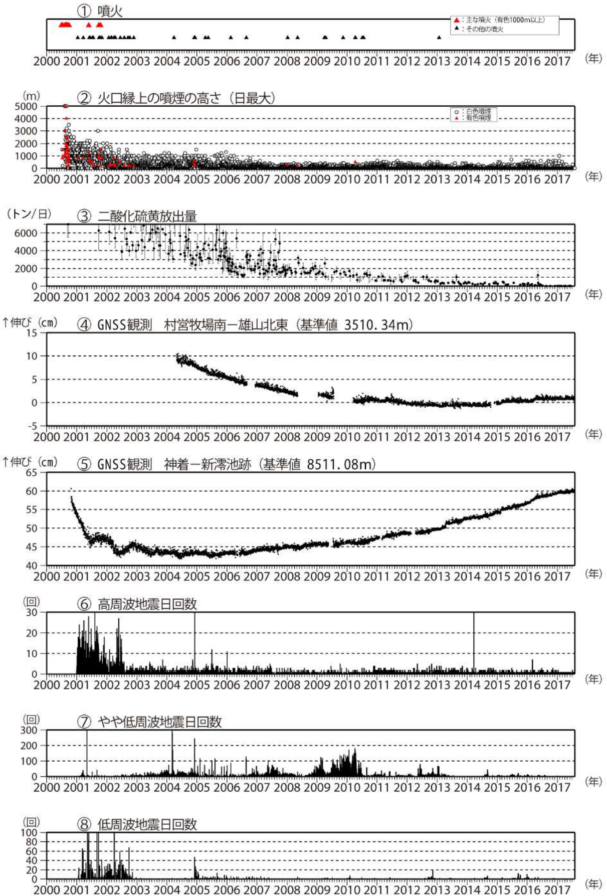
図5 三宅島 火山活動長期経過図（2000年1月1日～2017年7月31日）
