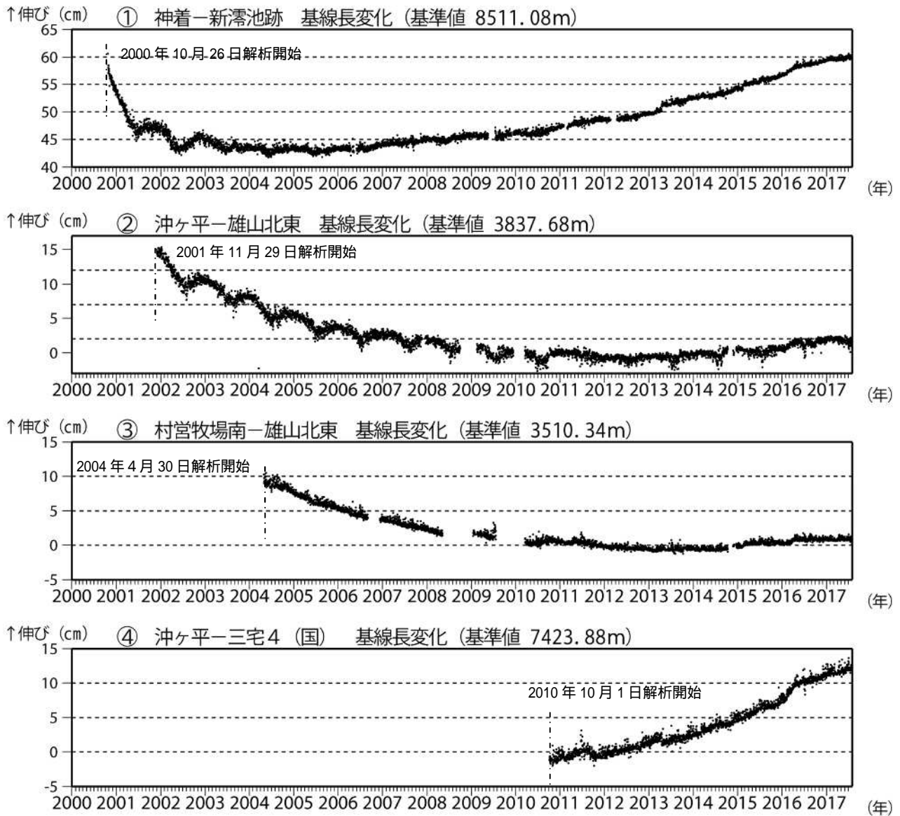
図7 三宅島 GNSS 連続観測結果 (2000 年 10 月 26 日 ~ 2017 年 7 月 31 日) (国): 国土地理院
