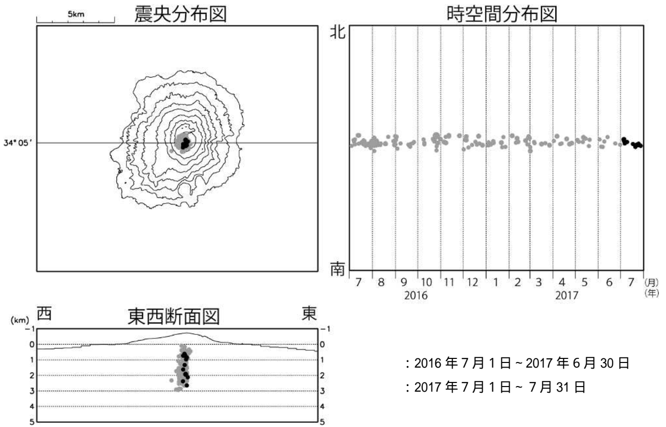
図 8 三宅島 震源分布図(2016 年 7 月 1 日 ~ 2017 年 7 月 31 日) ・震源は山頂火口直下に分布しており、これまでと比べて特段の変化は認められません。
