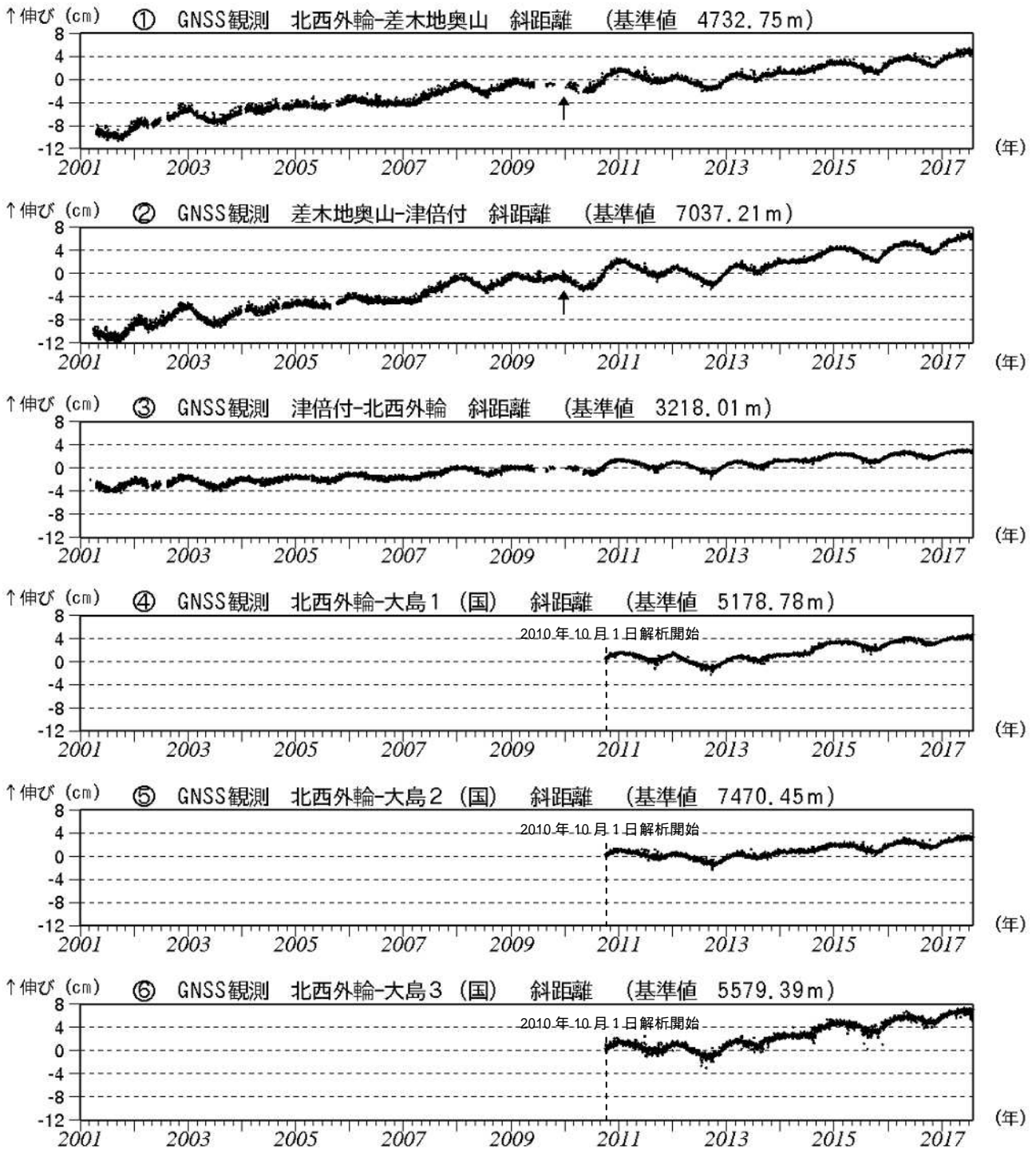
図3 伊豆大島 GNSS連続観測による基線長変化(2001年1月~2017年7月31日)
