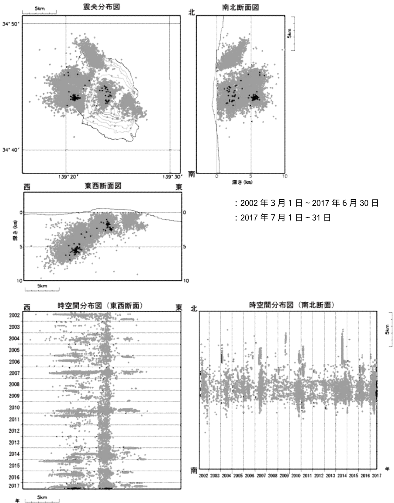
図4 伊豆大島 震源分布図(2002年3月1日~2017年7月31日)
