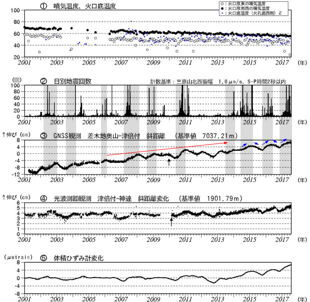
図2 伊豆大島 最近の火山活動経過図(2001年1月~2017年7月31日)
