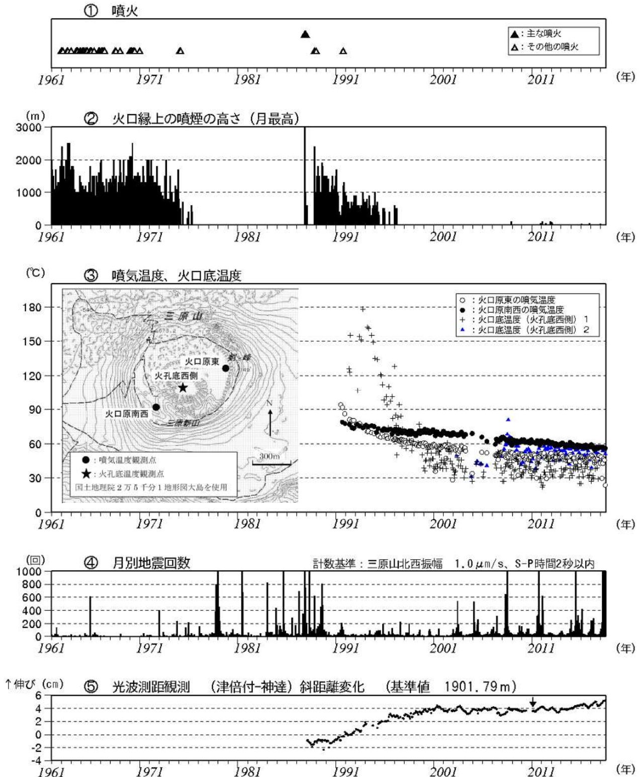
図 1 伊豆大島 長期間の火山活動経過図 (1961 年 1 月 ~ 2017 年 7 月 31 日)
