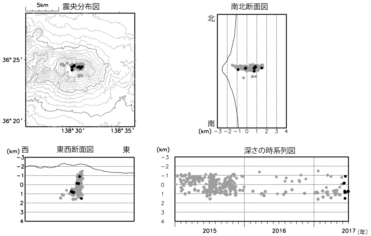
図5 浅間山 震源分布図（2015 年 1 月 1 日～2017 年 7 月 31 日）
