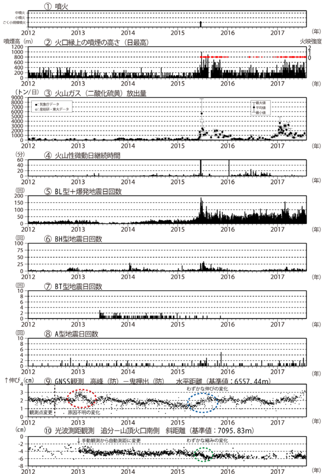
図4 浅間山 最近の火山活動経過図 (2012年1月1日～2017年7月31日)
