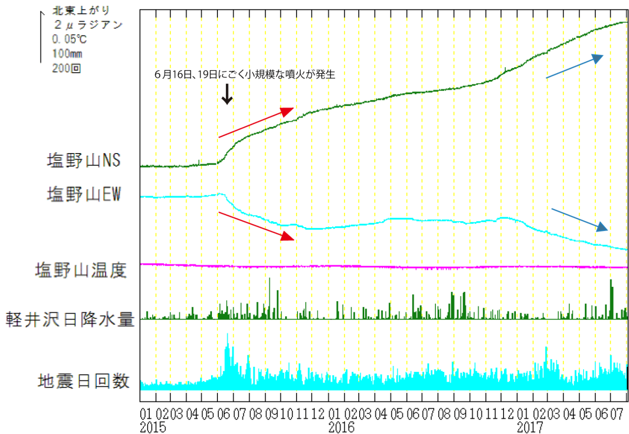
図8 浅間山 塩野山観測点における傾斜データ（2015 年 1 月 1 日～2017 年 7 月 31 日）
