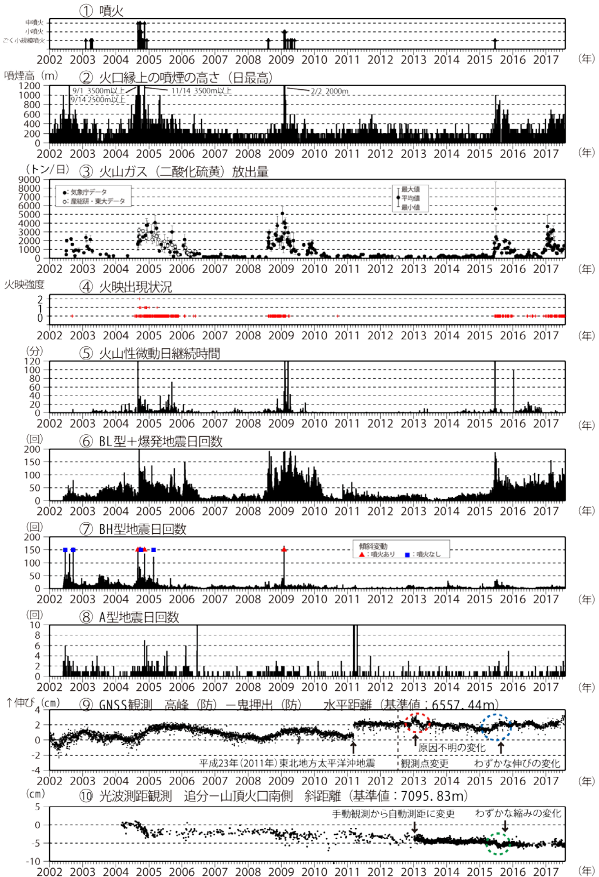
図3 浅間山 火山活動経過図 (2002年1月1日～2017年7月31日)
