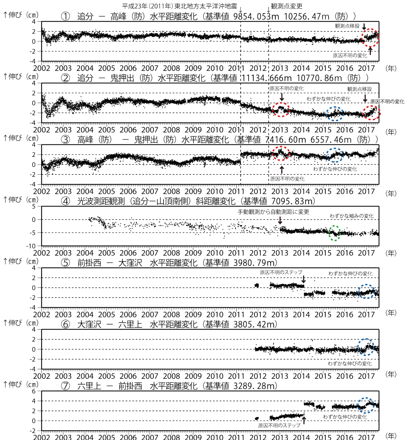
図6 浅間山 GNSS 連続観測及び光波測距観測の結果(2002 年 1 月 1 日～2017 年 7 月 31 日)
