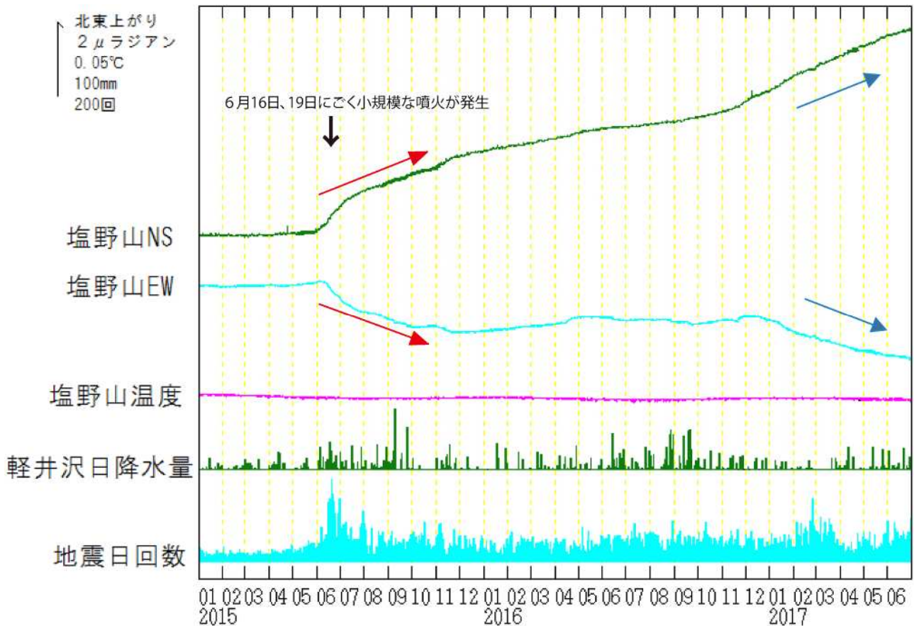
図8 浅間山 塩野山観測点における傾斜データ（2015 年 1 月 1 日～2017 年 6 月 30 日）
