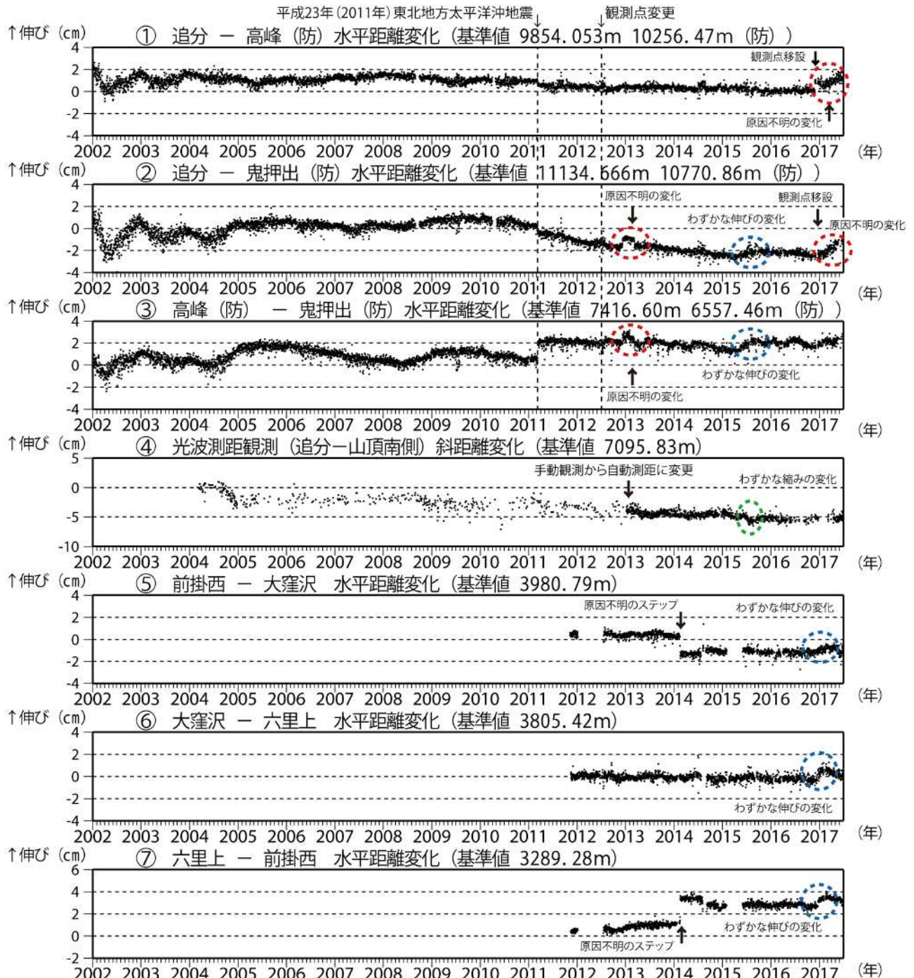
図6 浅間山 GNSS 連続観測及び光波測距観測の結果(2002 年 1 月 1 日～2017 年 6 月 30 日)
