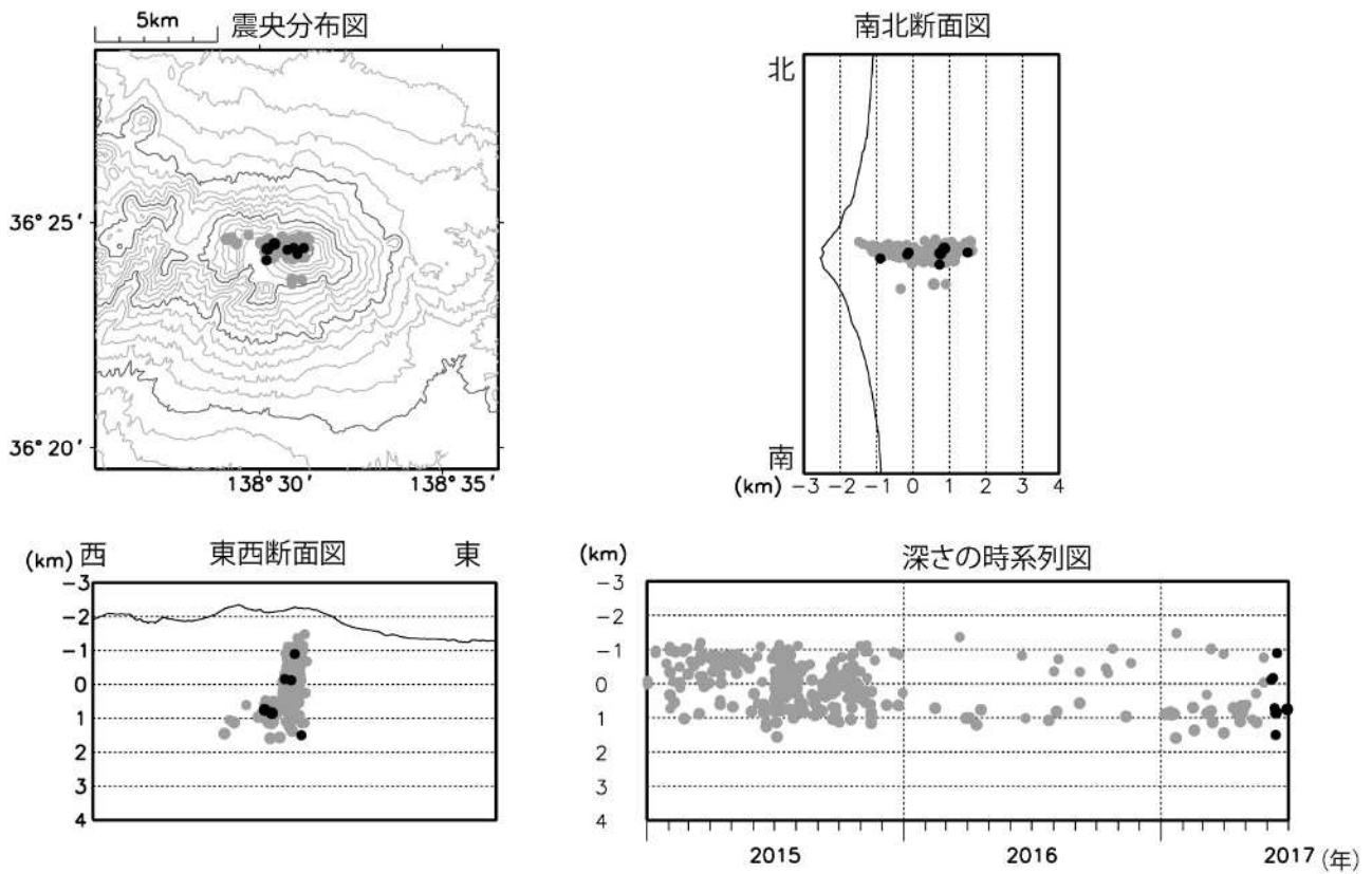
図5 浅間山 震源分布図（2015 年 1 月 1 日～2017 年 6 月 30 日）
