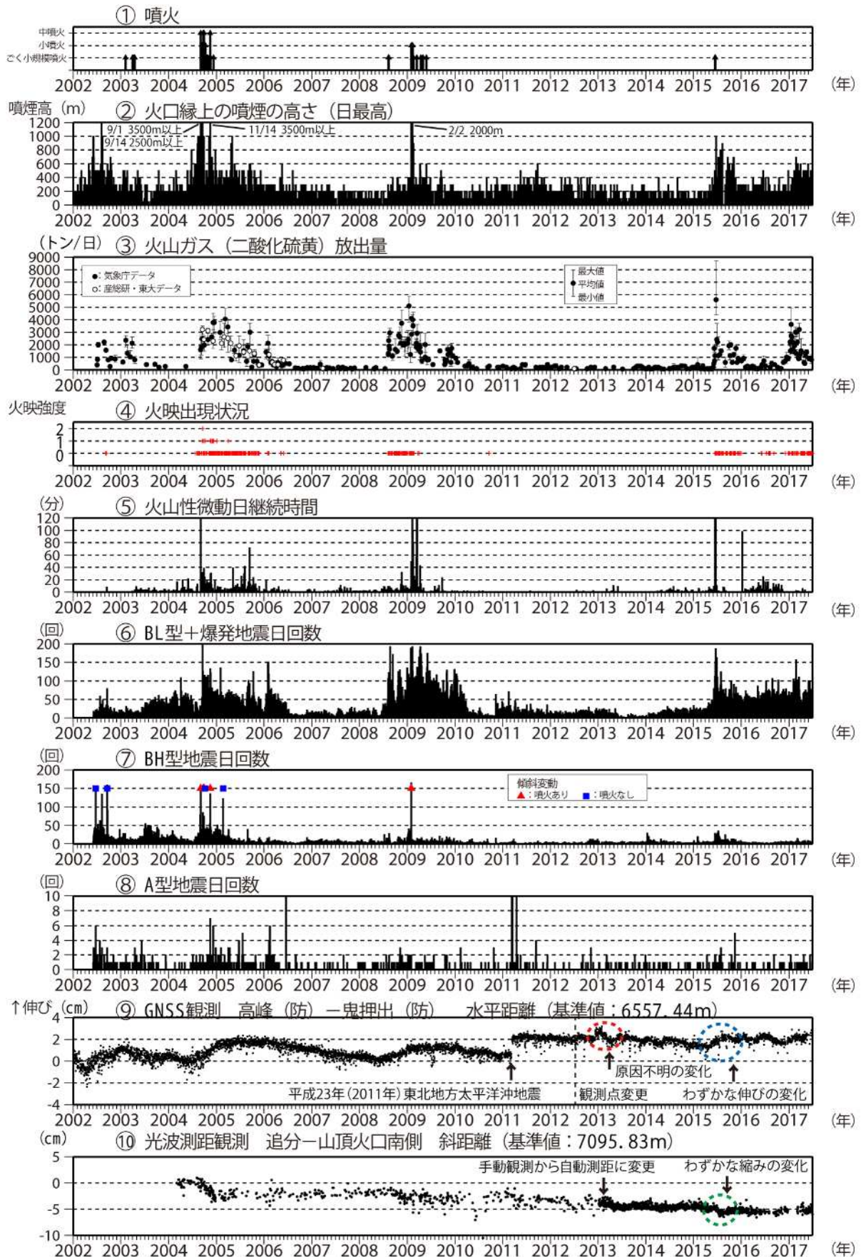
図3 浅間山 火山活動経過図 (2002年1月1日～2017年6月30日)
