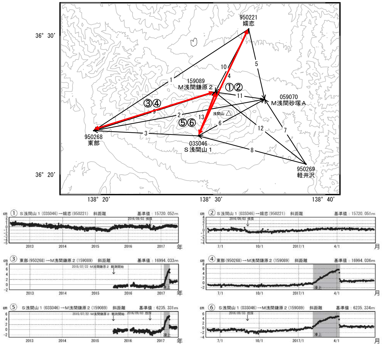
図 9 浅間山 国土地理院による地殻変動観測結果 6)
