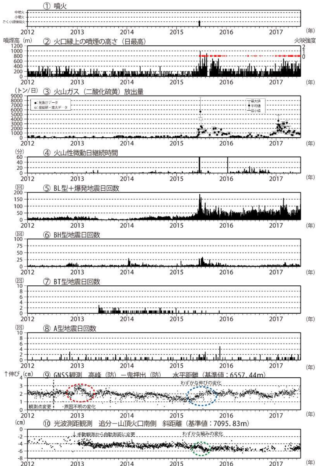
図4 浅間山 最近の火山活動経過図（2012年1月1日～2017年6月30日）
