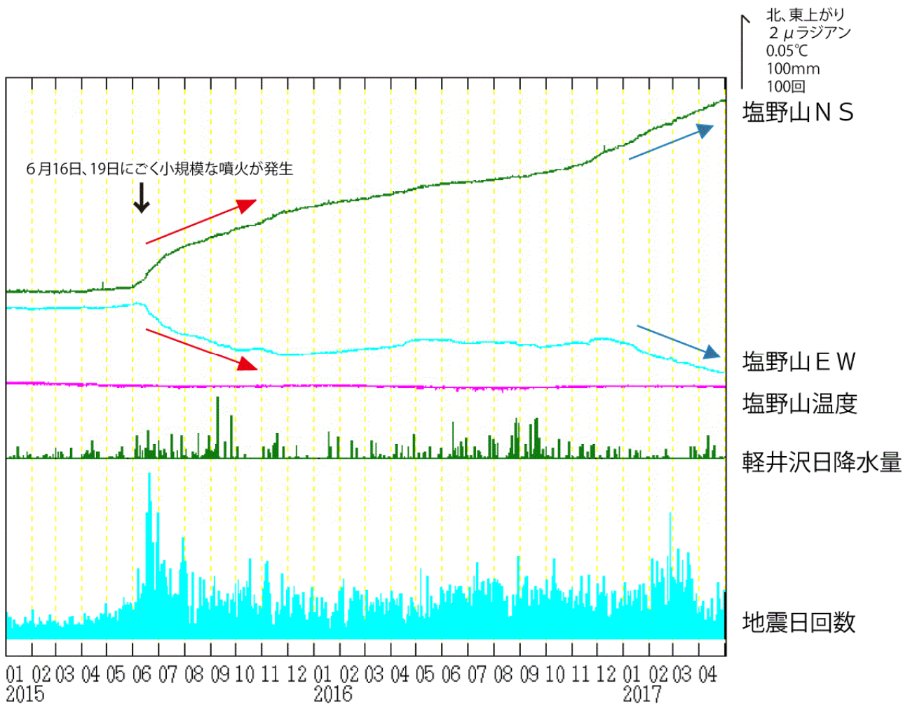
図8 浅間山 塩野山観測点における傾斜データ（2015 年 1 月 1 日～2017 年 4 月 30 日）
