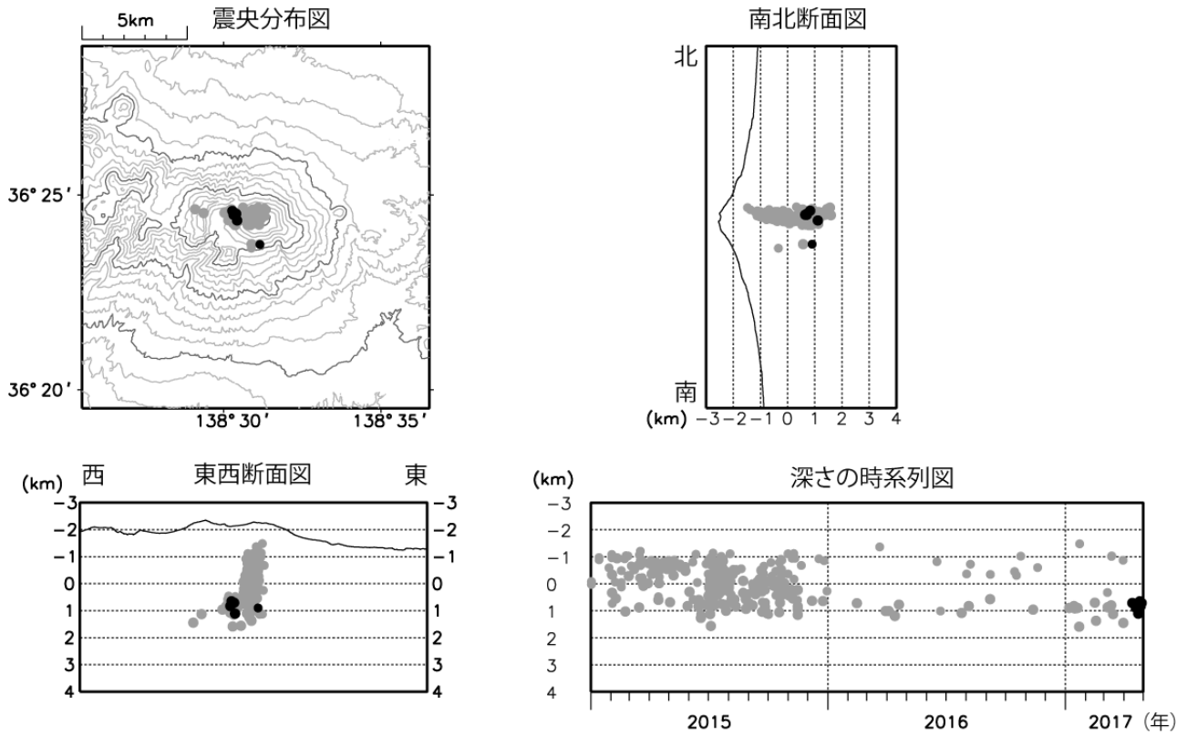
図 5 浅間山 震源分布図（2015 年 1 月 1 日～2017 年 4 月 30 日）
