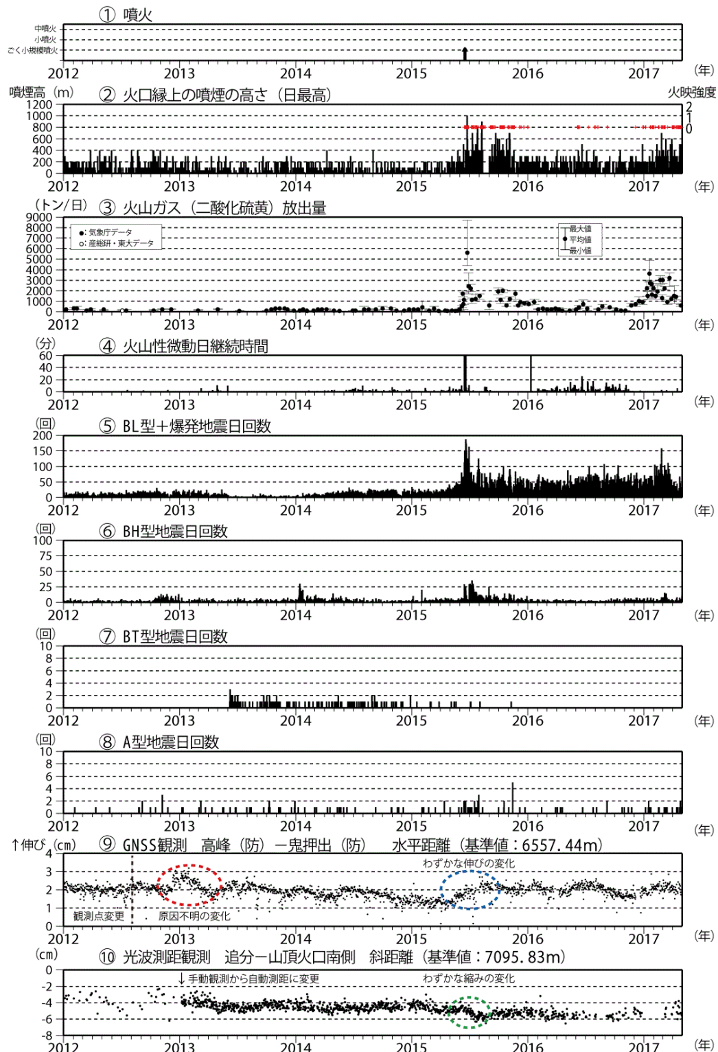
図 4 浅間山 最近の火山活動経過図（2012 年 1 月 1 日～2017 年 4 月 30 日）
