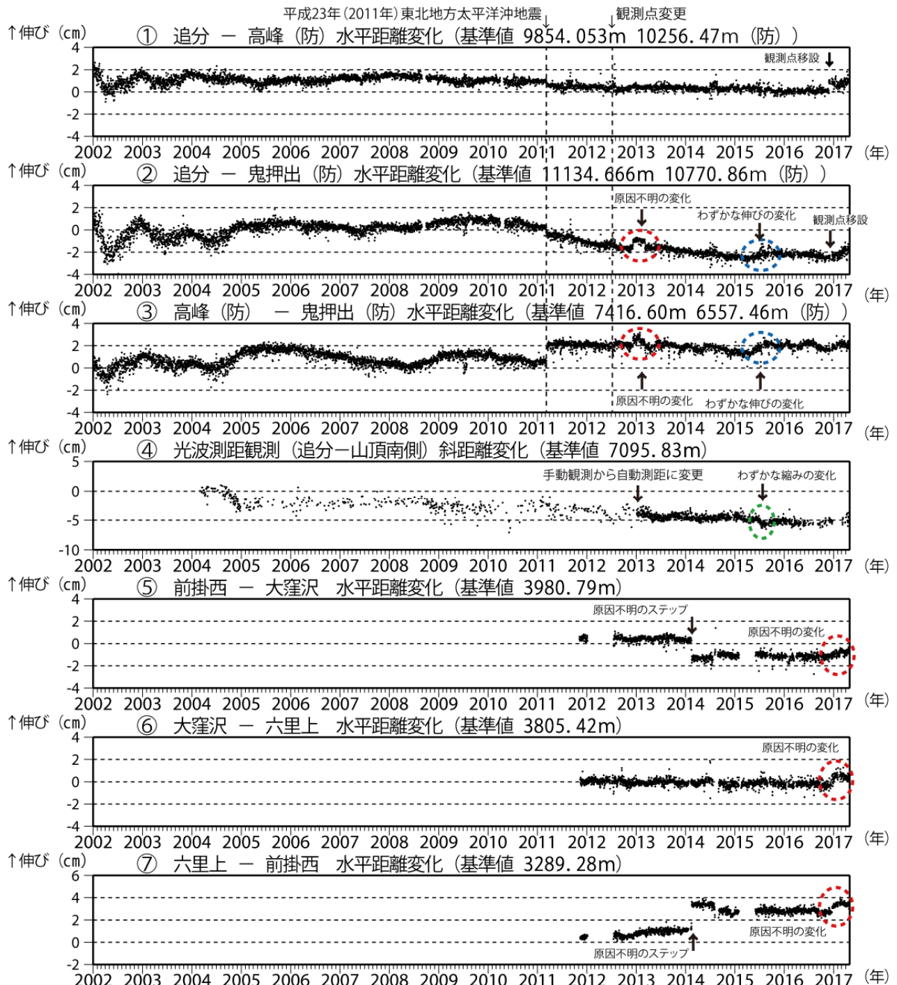
図6 浅間山 GNSS 連続観測及び光波測距観測の結果 (2002 年 1 月 1 日～2017 年 4 月 30 日)
