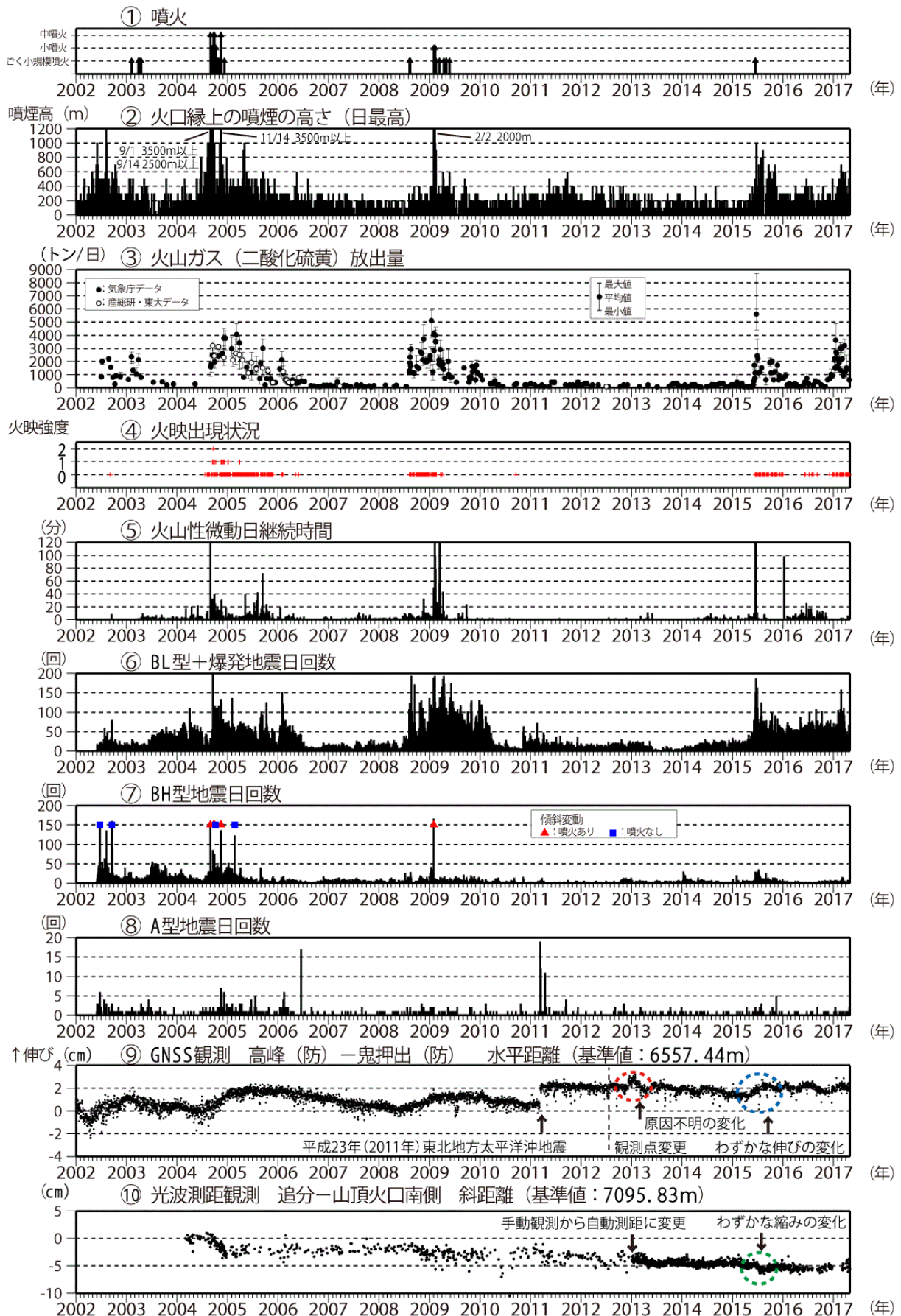
図3 浅間山 火山活動経過図 (2002年1月1日～2017年4月30日)
