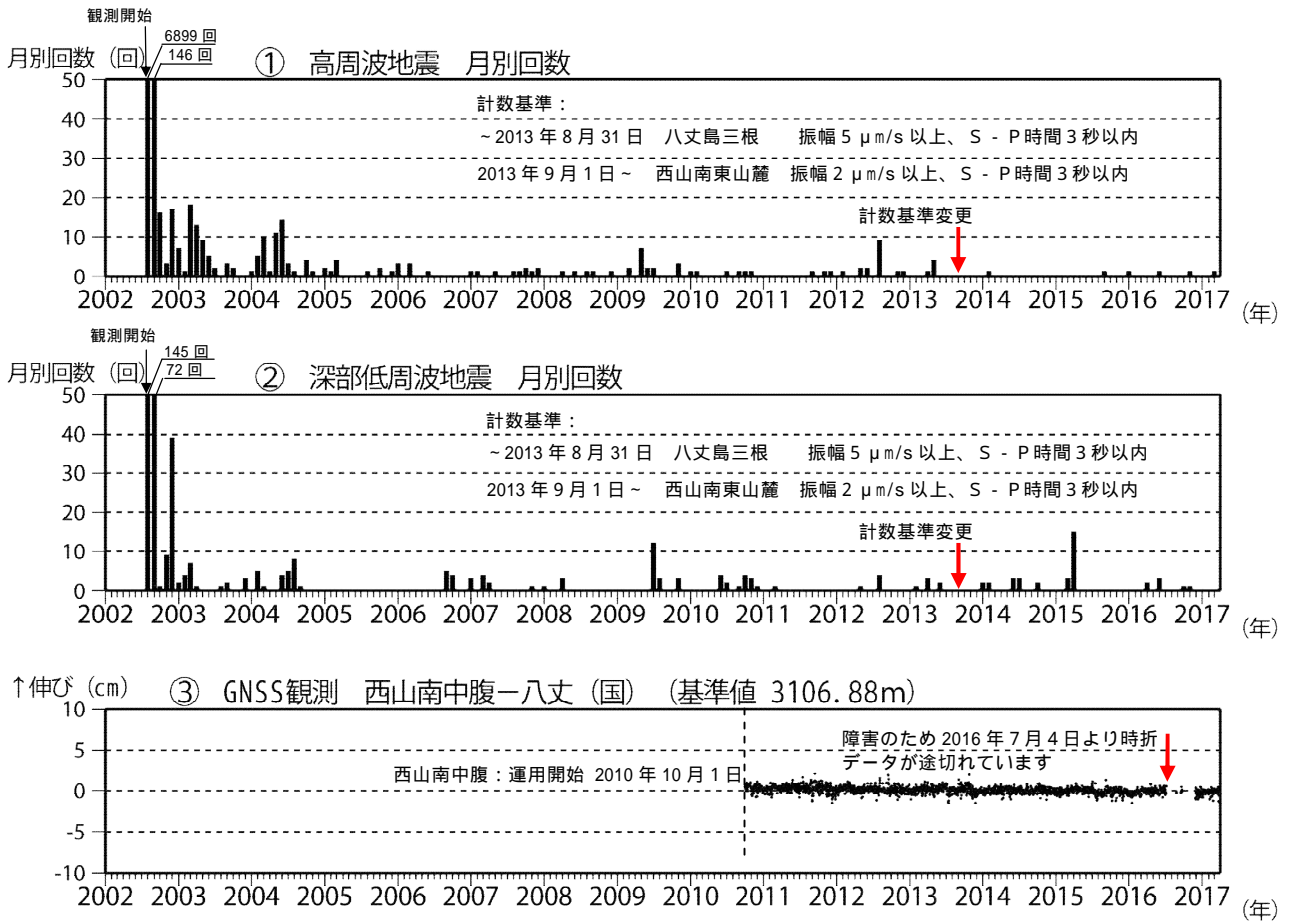
図2 八丈島 火山活動経過図(2002年8月13日~2017年3月31日)
