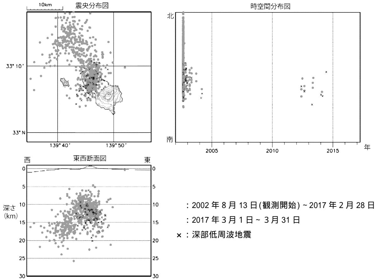
図3 八丈島 震源分布図(2002年8月13日~2017年3月31日) ・今期間、八丈島付近に震源が求まる高周波地震及び深部低周波地震はありませんでした。
